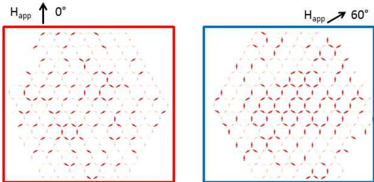
Figure IV.13 Aimantations dont la direction a changé pour un champ appliqué de 1.02 kOe. A gauche, 0° ; à droite, 60°.
