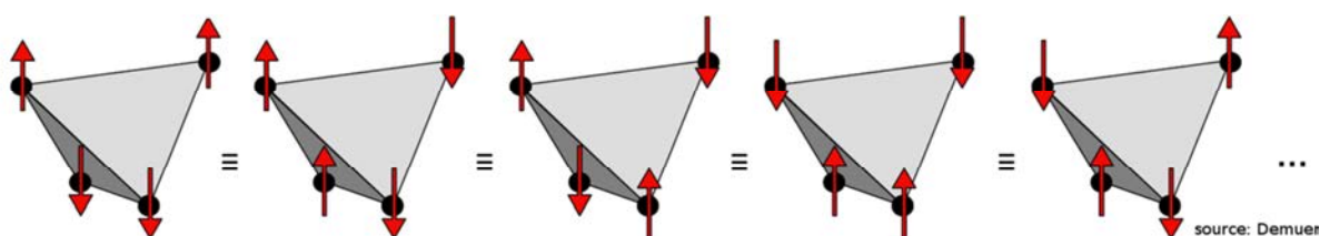
Figure I.2 Exemple du cas à 3 dimensions de spins classiques en interactions, ceux-ci sont disposés aux sommets d'un tétraèdre (figure extraite de la thèse de Y. Chapuis [CHA10])
