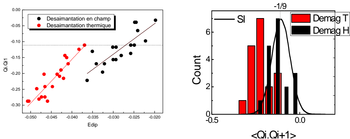
Figure V.7 A gauche : variation du corrélateur de charges en fonction de l'énergie dipolaire longue portée pour la désaimantation thermique (en rouge) et sous champ (en noir) ; à droite : nombre de configurations ayant un corrélateur de charges donné pour la désaimantation thermique (en rouge) et sous champ (en noir). La courbe noire représente la courbe attendue dans un modèle SI.
