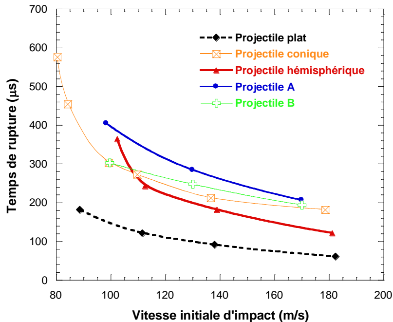
Fig.III.29 Temps de rupture fonction de la vitesse initiale d'impact pour différentes projectiles.
