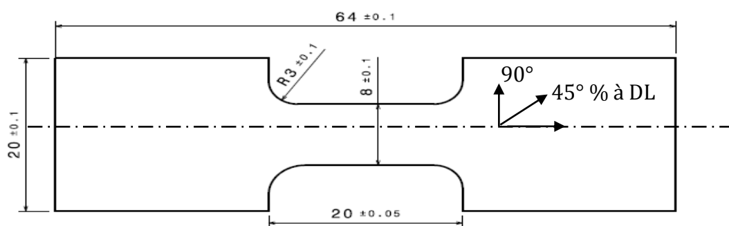
Fig. II. 3 Géométrie de l'éprouvette de traction suivant la direction de laminage.
