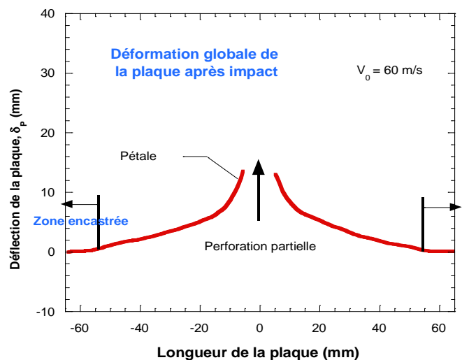
Fig.II.15 a- Profilomètre utilisé pour la mesure de déflexion permanente des plaques; b- Résultats expérimentaux de la déflexion de la plaque, V_0 = 60 m/s.
