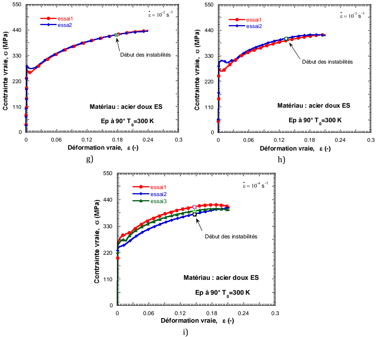
Fig.V.5 Résultats des essais de traction sur l'acier doux. a-, b-, c- Eprouvette à 0^\circ ; d-, e-, f- Eprouvette à 45^\circ ; g-, h-, i- Eprouvette à 90^\circ .
