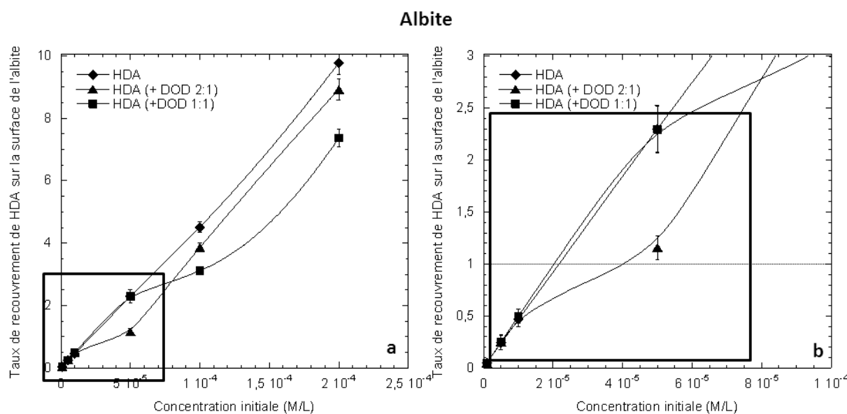
Figure 7-7 - Taux de recouvrement de la surface de l'albite par HDA (a) et zoom sur la zone de recouvrement \theta=1 à l'aide de HDA (b) en fonction du type de mélange HDA - DOD à pH 8.
