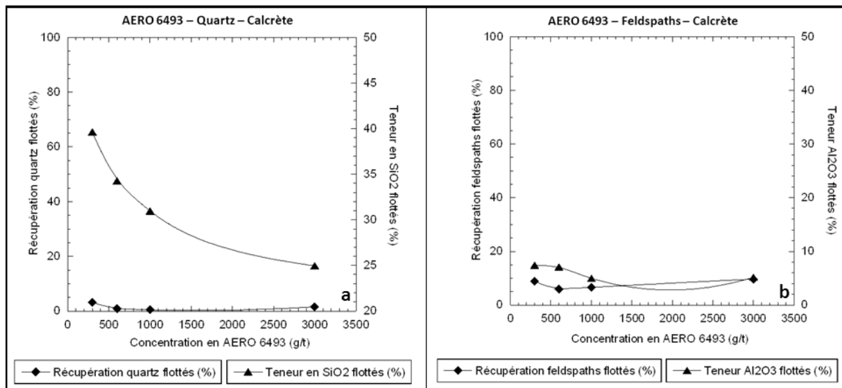
Figure 8-3 - Taux de récupération du quartz et teneur en SiO 2 (a) et taux de récupération des feldspaths et teneur en Al 2 O 3 (b) dans les flottés en fonction de la concentration en AERO 6493.
