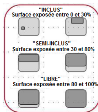
Figure 3-5 - Définition du caractère textural déduit du pourcentage de la surface exposée, (Coetzee et Theron, 2007).
