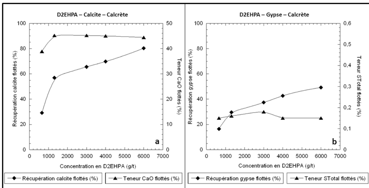
Figure 8-6 - Taux de récupération de la calcite et teneur en CaO (a) et taux de récupération du gypse et teneur en STotal (b) dans les flottés en fonction de la concentration en D2EHPA (calcrète).
