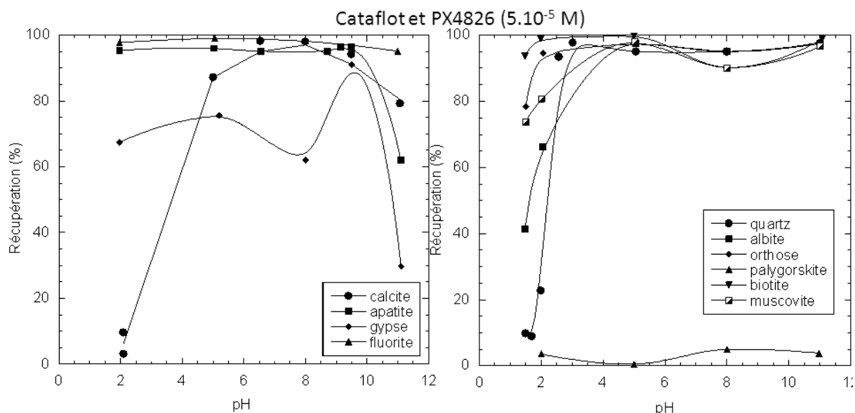
Figure 6-6 - Flottation des minéraux du calcium et des silicates à l'aide du Cataflot CSO et PX4826 ( 5 \cdot 10^{-5} M) suivant le pH
