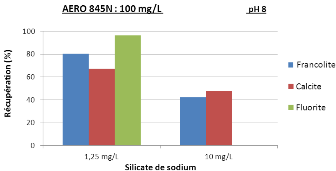
Figure 6-20 - Influence de la concentration en silicate de sodium sur la carbonato-fluoro apatite, la calcite et la fluorite à l'aide de 100 mg/L d'AERO 845 N à pH 8.
