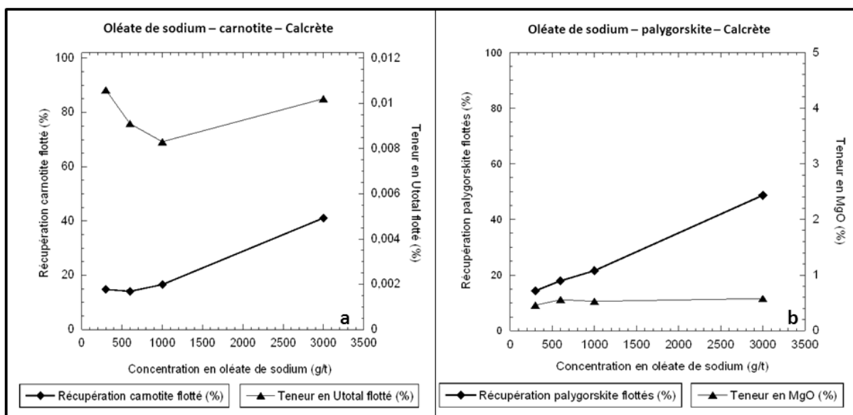
Figure 8-13 - Taux de récupération de la carnotite et teneur en UTtotal (a) et taux de récupération de la palygorskite et teneur en MgO (b) dans les flottés en fonction de la concentration en oléate de sodium à pH 8 (calcrète).
