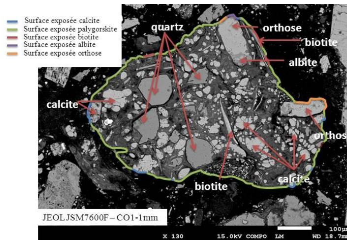
Figure 3-4 – Surfaces exposées des minéraux inclus et de la phase minérale majoritaire d'une particule mixte.
