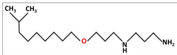
Figure 2-21 – Formule chimique semi-développée du PX4817 (N-[Isodécyloxy]propyl]propane-1,3-diamine (C-16)
