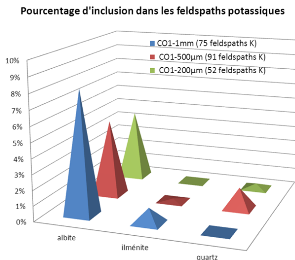
Figure 4-17 – Pourcentage d'inclusion dans les feldspaths potassiques en fonction du degré de broyage.
