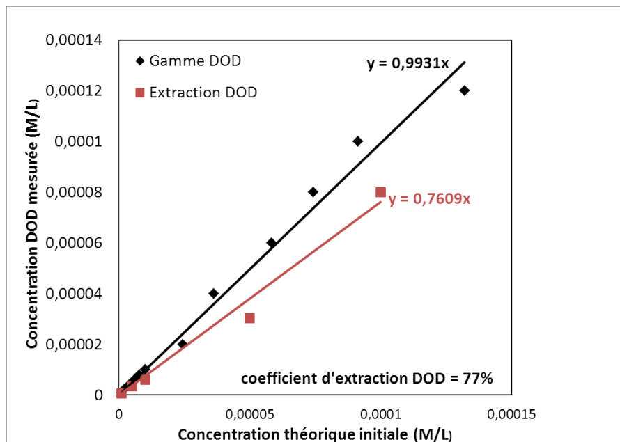
Figure 3-21 – Coefficient d'extraction du dodécane
