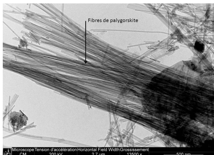
Figure 2-5 - fibres de palygorskite, minéral de Trekkopje, faciès calcrète (Image MET tirée de cette étude)
