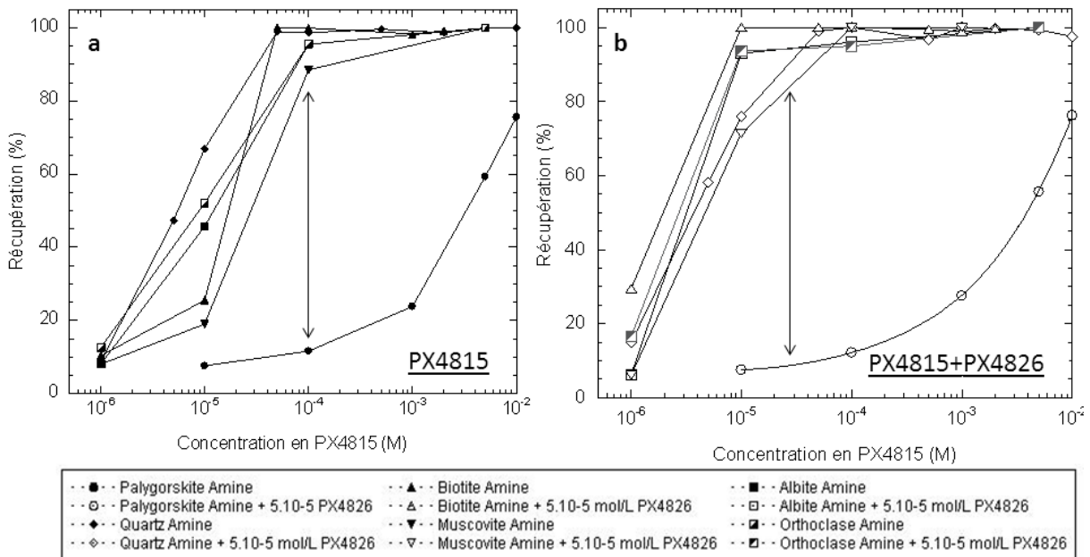
Figure 6-2 - Taux de récupération du quartz, du microcline, de l'albite, de la biotite, de la muscovite et de la palygorskrite par flottation à pH 8 à l'aide de PX4815 seul (a) ou avec un réactif non ionique PX4826 (b).
