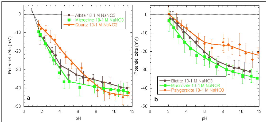
Figure 5-12 – Potentiel zêta du quartz, albite et microcline (a), de la biotite, de la muscovite et de la palygorskite (b) dans 10^{-1} M de NaNO 3 en fonction du pH.
