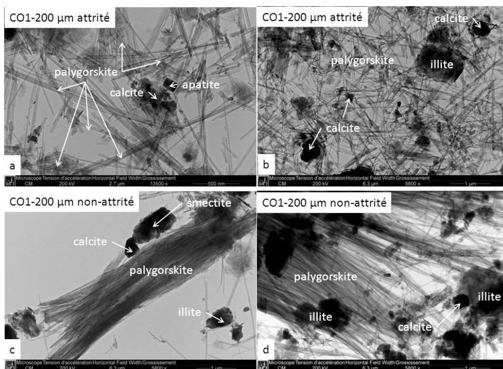
Figure 4-4 – Photographies réalisées au microscope électronique à transmission (MET) FEI CM20, a. cristaux de palygorskite, calcite, apatite dans CO1-200 μm attrité, b. cristaux de palygorskite, calcite, illite dans CO1-200 μm attrité c. fuseau de palygorskite, cristaux de calcite, smectite et illite dans CO1-200 μm non-attrité, d. amas d’argile – palygorskite, illite, calcite dans CO1-200 μm non-attrité.
