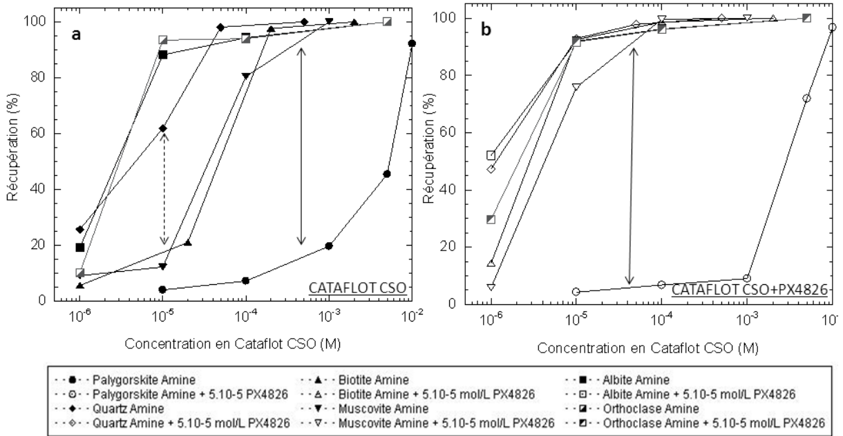
Figure 6-1 - Taux de récupération du quartz, du microcline, de l'albite, de la biotite, de la muscovite et de la palygorskrite par flottation à pH 8 à l'aide de Cataflot CSO seul (a) ou avec un réactif non ionique PX4826 (b).
