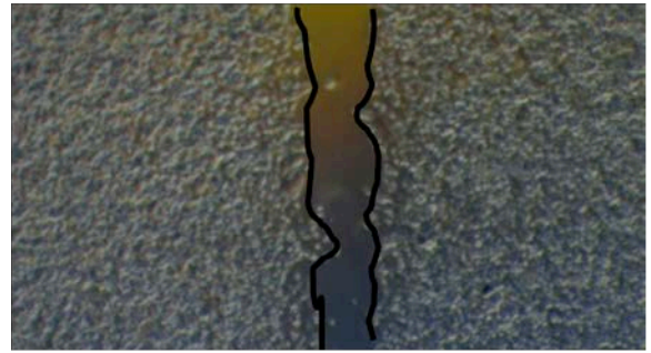
C pCMV-Siah1L
