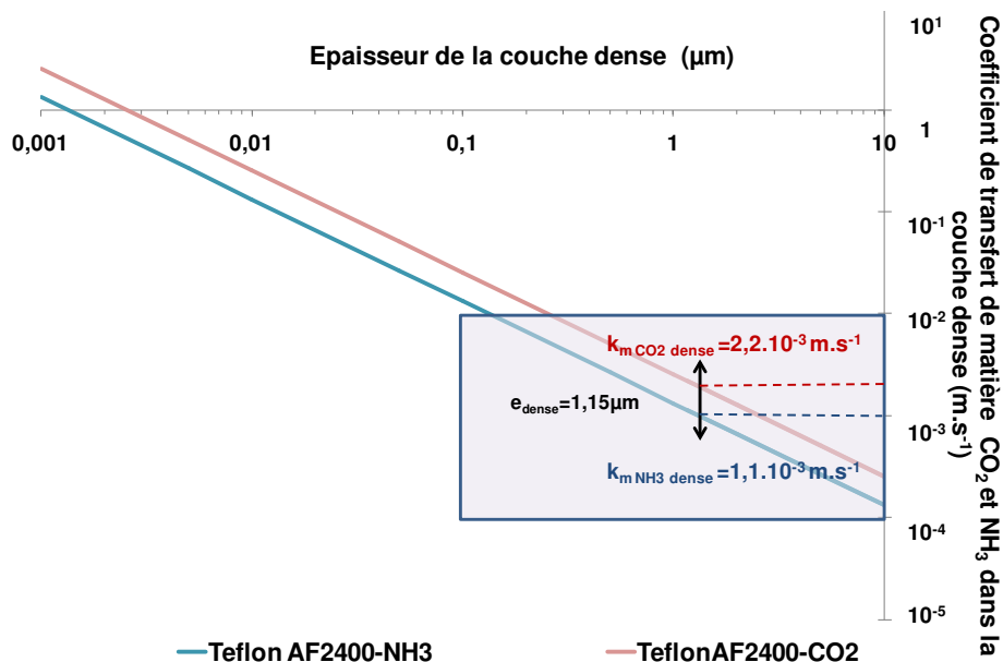
Figure C-2 Coefficient de transfert de matière k_{m i, \text{dense}} du \text{CO}_2 et de \text{NH}_3 au travers du Teflon AF2400 en fonction de son épaisseur
