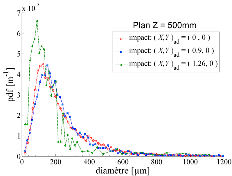
Figure 3.8: Evolution dans la direction X des courbes de pdfs du diamètre en configuration d'impact
