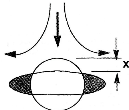
Figure 2.1: Dans le modèle TAB le déplacement x de l'équateur décrit la déformation de la goutte.
