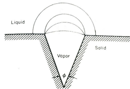
Figure 1.7: Schéma d'un site d'ébullition, d'ouverture \Phi
