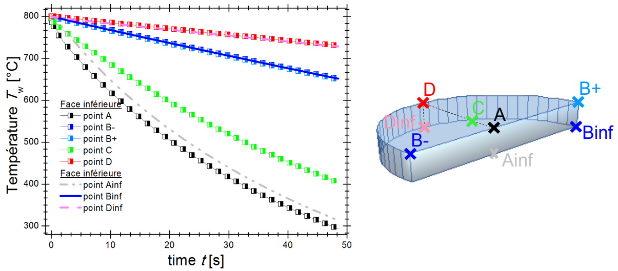
Figure 4.7: Evolution de la température de la plaque en fonction du temps, en différents points sur les faces supérieure et inférieure.
