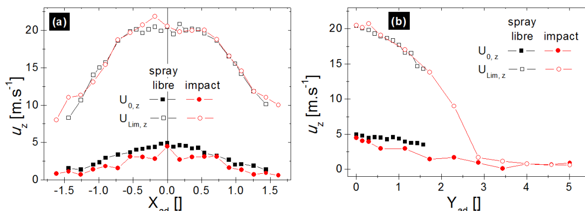
Figure 3.13: Comparaison entre le spray libre et le spray impactant des vitesses U_{0,z} (symboles pleins) et U_{\text{Lim},z} (symboles creux), le long des axes X (a) et Y (b).
