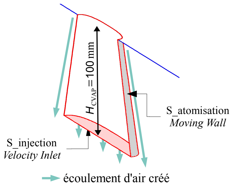
Figure 2.16: Visualisation du Cône Virtuel d'Atomisation Primaire (CVAP) et de la surface d'initialisation, représentée dans le domaine entier sur la figure 2.15. Les conditions limites sont inscrites en lettres italiques.
