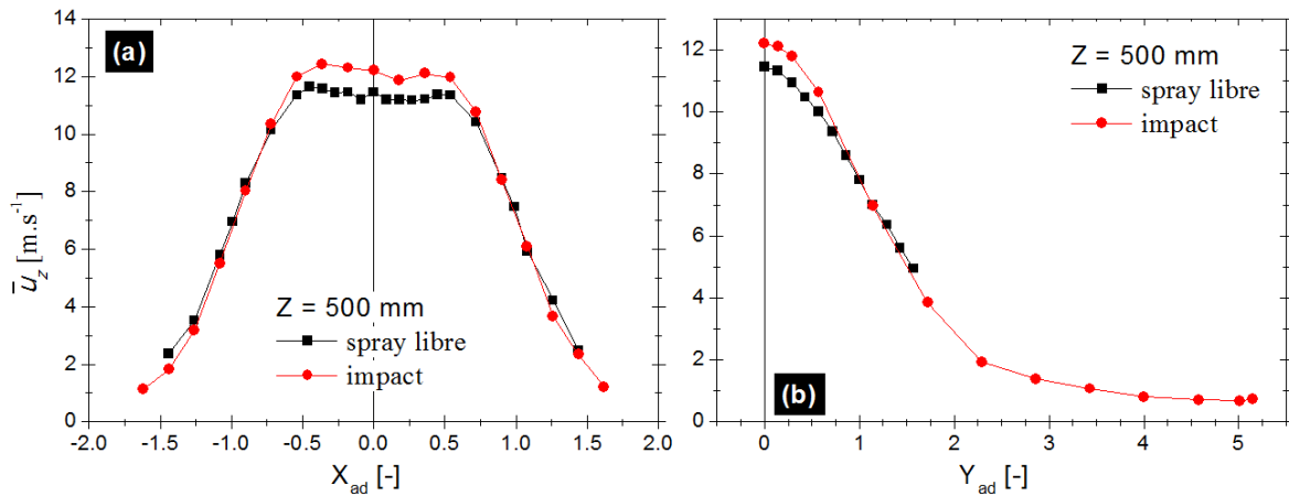
Figure 3.10: Comparaison de la vitesse axiale moyenne \bar{u}_z pour le spray libre et le spray impactant, le long des profils Y_{ad}=0 (a) et X_{ad}=0 (b), dans le plan Z = 500 mm.
