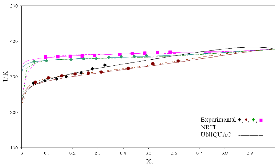
(b) Fructose
