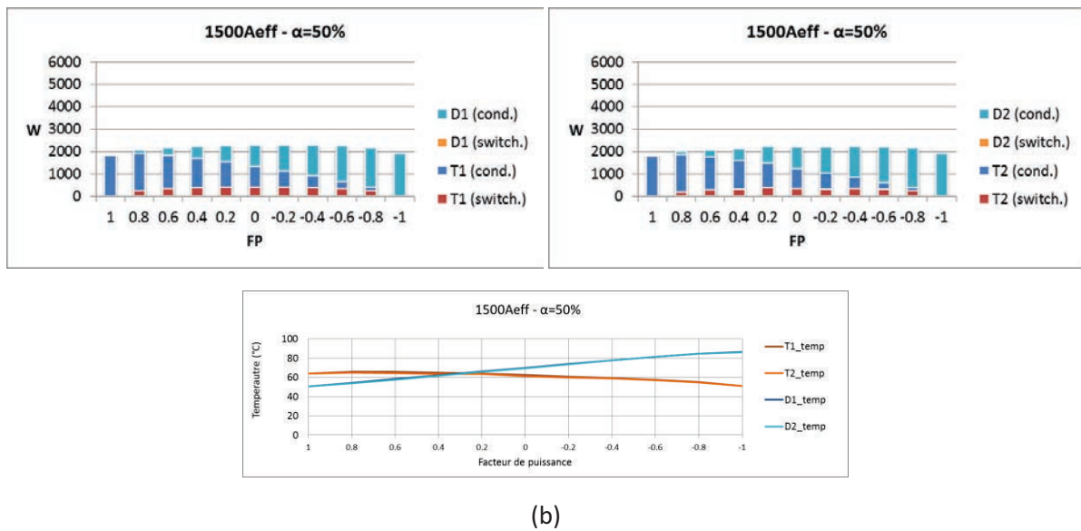
Figure 40 : Evolution des pertes et des températures de jonction en fonction du rapport cyclique et du facteur de puissance
