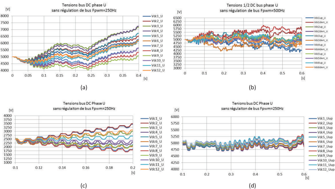
Figure 21 : Divergence des bus DC phase U: (a) Pont en H configuration en triangle ; (b) pont en H 3-niveaux configuration triangle ; (c) pont en H configuration étoile ; (d) \frac{1}{2} pont en H configuration étoiles-symétriques (MMC)
