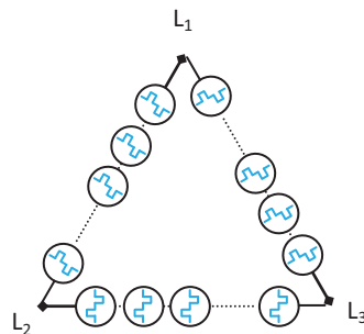
Figure 60 : Couplage de modules en triangle
