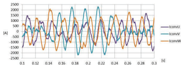
Figure 26 : Courants triphasés traversant les modules
