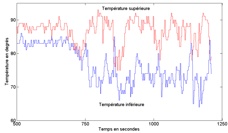
FIGURE 5.21 – Températures des thermocouples de la colonne 16
