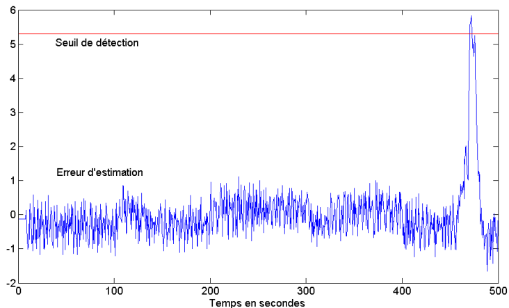
FIGURE 5.4 – Détection du collage
