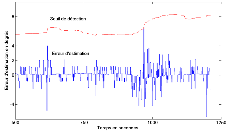
FIGURE 5.20 – Situation de fausse alarme sur la colonne 3
