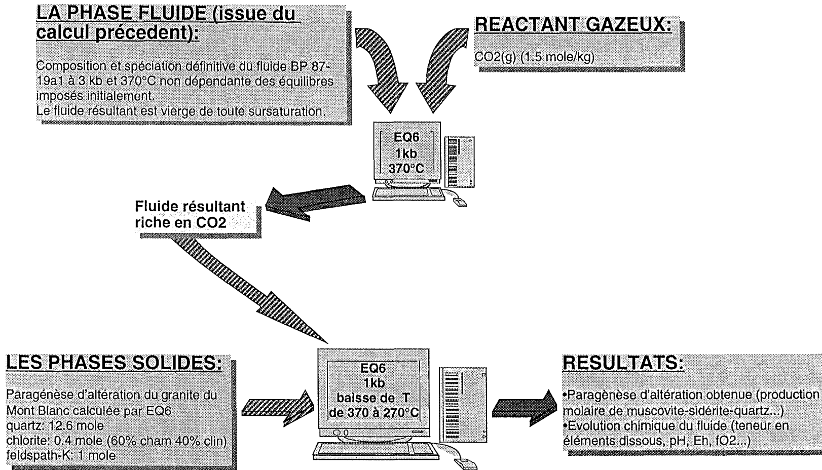
Figure 35: Les différentes étapes de la simulation de l'altération de la paragenèse du stade I d'altération (quartz-chlorite-albite-adulaire) en quartz(améthyste)-muscovite-ankérite.
