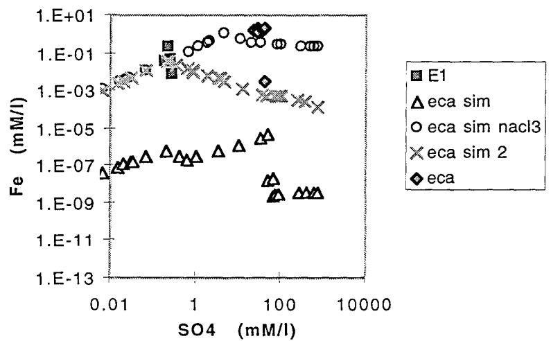
Figure 75: Diagrammes binaires des teneurs en éléments Ca, Mg et Fe en fonction de la teneur en sulfate dans les fluides de l'Ecarpière. eca: fluides prélevés sur le site (SBS9, SBS11,...) - eca sim, eca sim 2, eca sim nacl3: fluides simulés avec EQ6 - E1: fluide expérimental.
