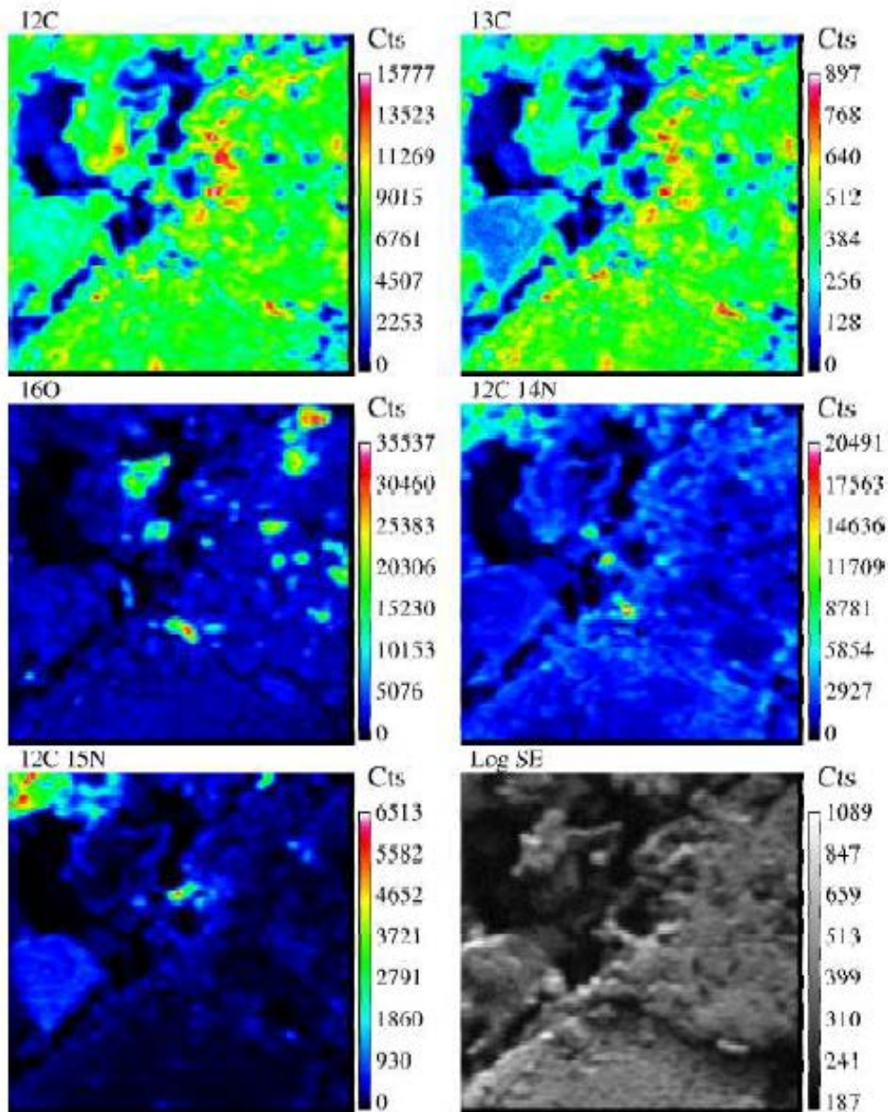
Figure 4 : Images NanoSIMS de feuilles de litière de hêtre doublement marquées au ^{13}\text{C} et ^{15}\text{N} issues de l'étude menée par Hatton et al. (2012). Par comparaison des images ^{12}\text{C}^{14}\text{N} et ^{12}\text{C}^{15}\text{N} on observe une distribution du ^{15}\text{N} similaire à la distribution du ^{14}\text{N} .
