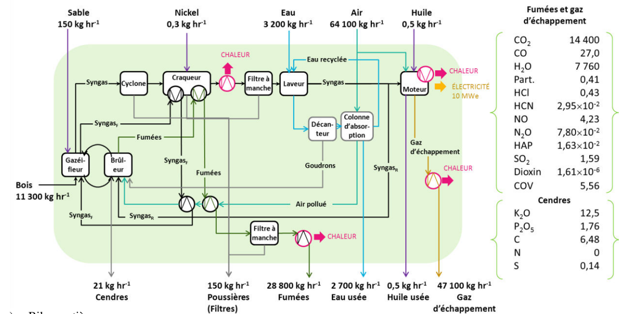
a) Bilan matière
