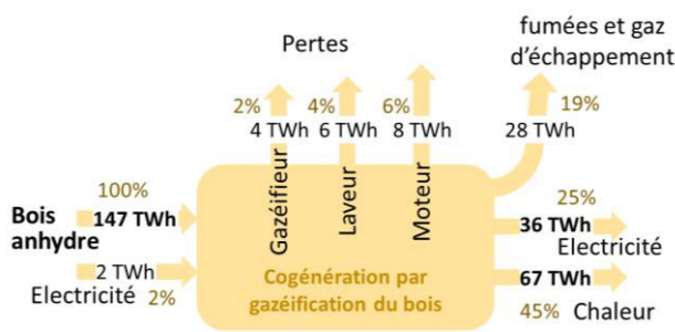
b) Bilan énergie
