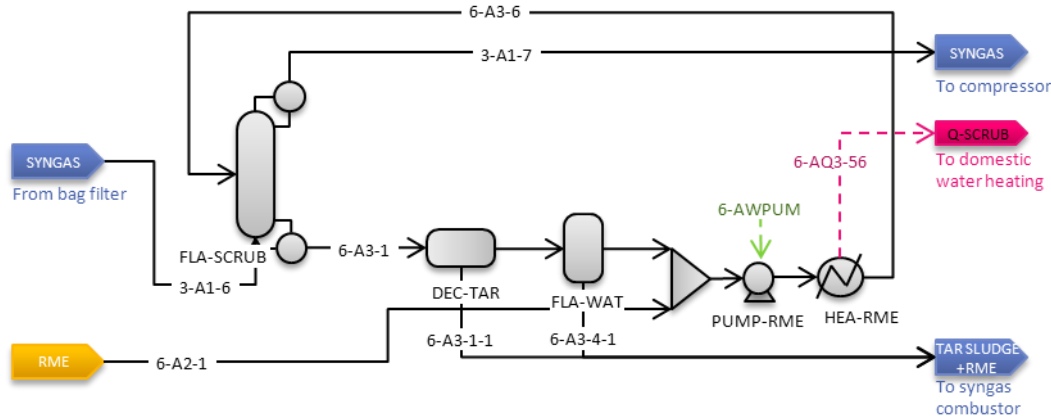
Figure 1-2/5. Schéma du modèle Aspen Plus du laveur au RME.
