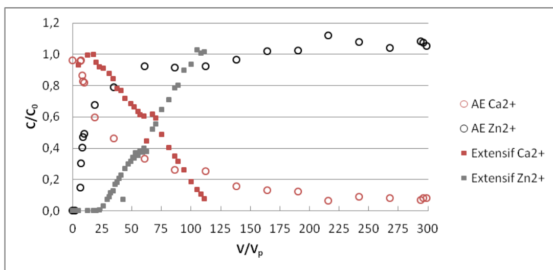
Figure 31 - Evolution du rapport C/C_0 de Ca 2+ et Zn 2+ pour l'argile expansée (AE) et le substrat extensif en fonction du volume écoulé sur le volume poreux de la colonne
