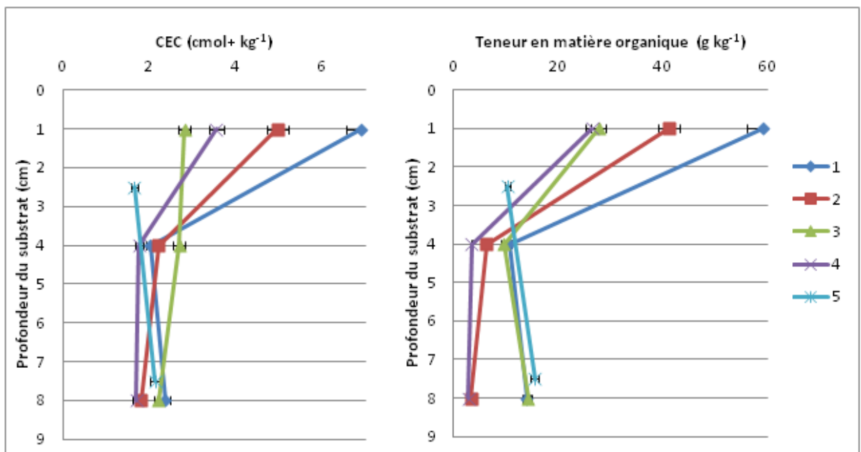
Figure 56 - Variabilité de la CEC et de la teneur en matière organique entre les différents points de prélèvements sur la toiture Extensive
