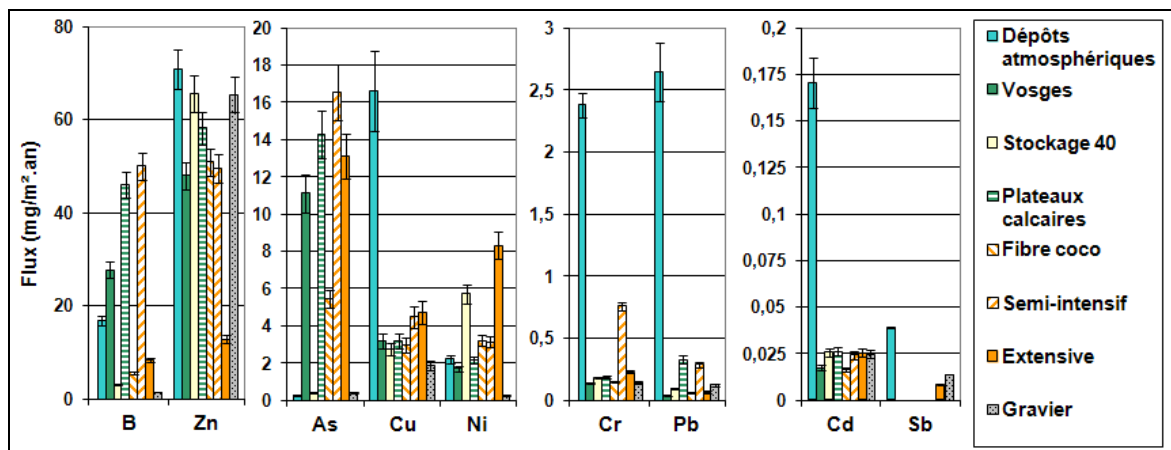
Figure 41 – Comparaison des flux d'ETM moyen annuel en entrée et sortie des différentes toitures
