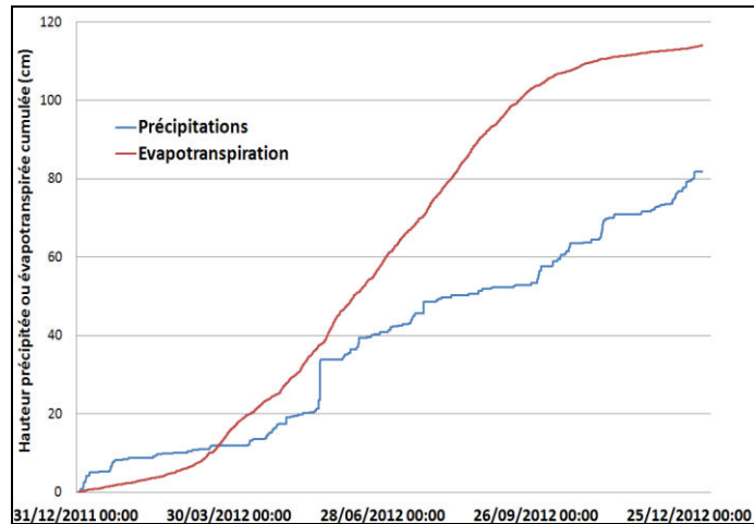
Figure 90 : Comparaison de l'évapotranspiration calculée et des précipitations réelles sur 2012
