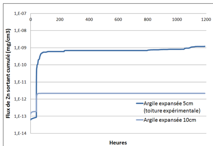
Figure 92 : Impact de la hauteur de drainage sur les flux de zinc cumulé en sortie de toiture
