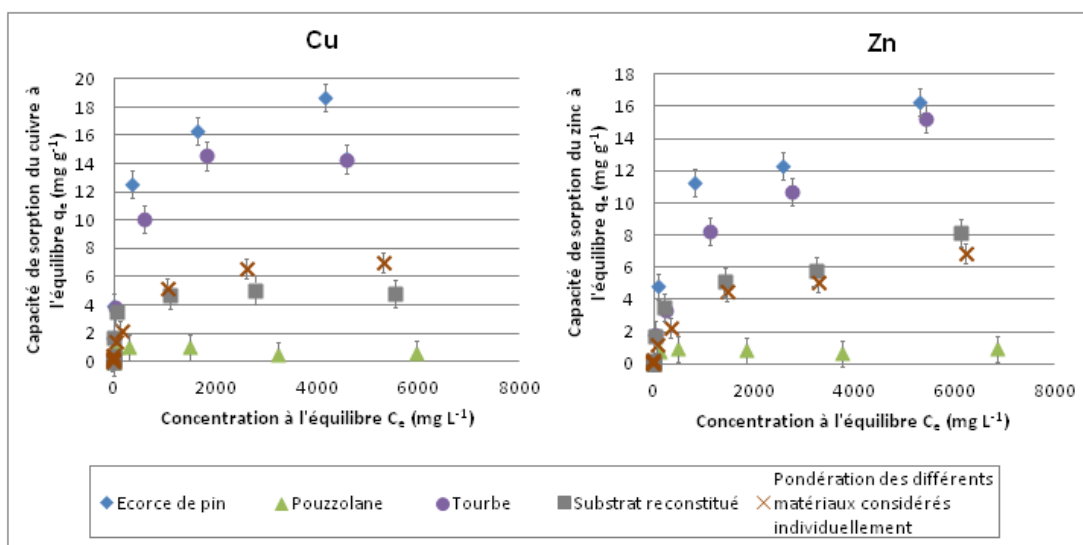
Figure 29 - Evolution de la capacité de sorption du Cu par les principaux matériaux constitutifs du substrat extensif considérés individuellement et en mélange
