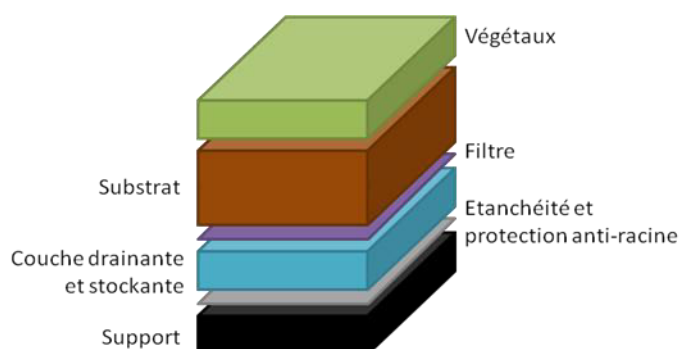
Figure 4 - Structure multicouches d'une toiture végétalisée
