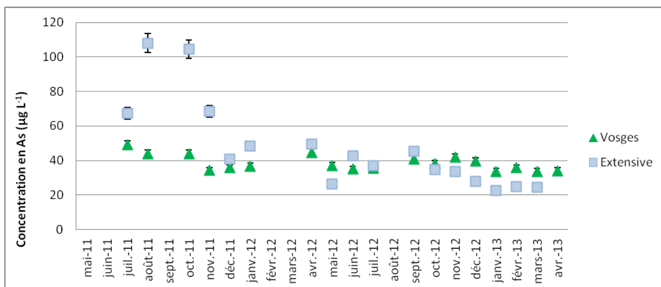
Figure 39 – Comparaison de l'évolution des concentrations totales en arsenic en sortie des toitures végétalisées Vosges et Extensive entre mai 2011 et avril 2013
