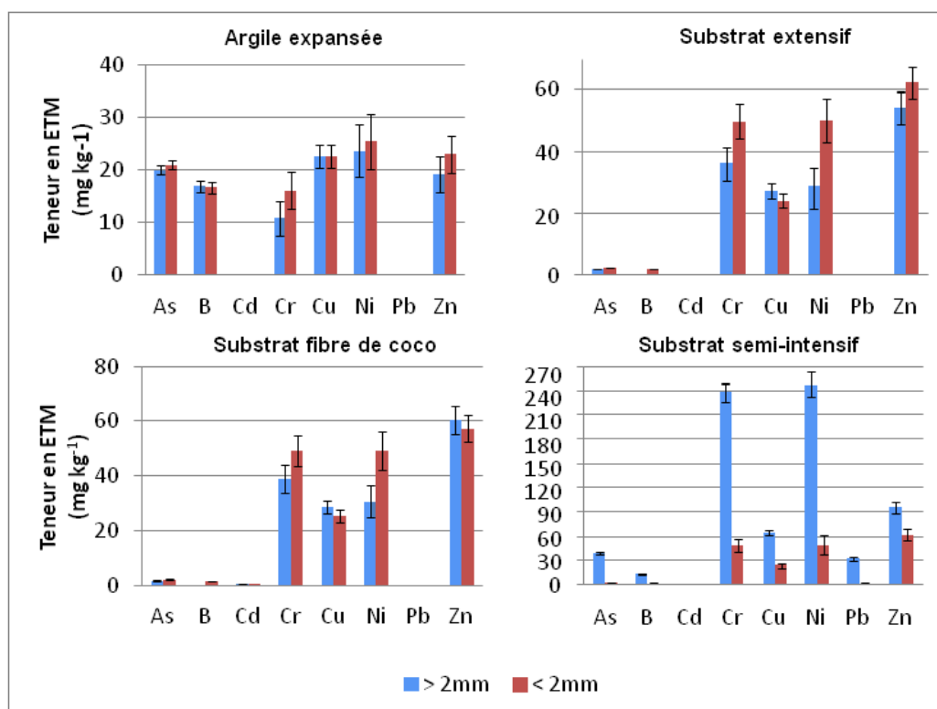
Figure 23 - Variation des teneurs en ETM dans les fractions granulométriques des trois substrats et l'argile expansée
