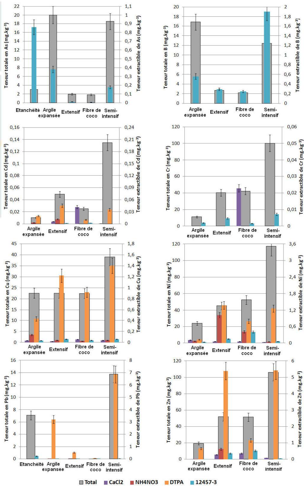
Figure 24 - Extractibilité des ETM sur les trois substrats, l'argile expansé et l'étanchéité selon différentes méthodes
