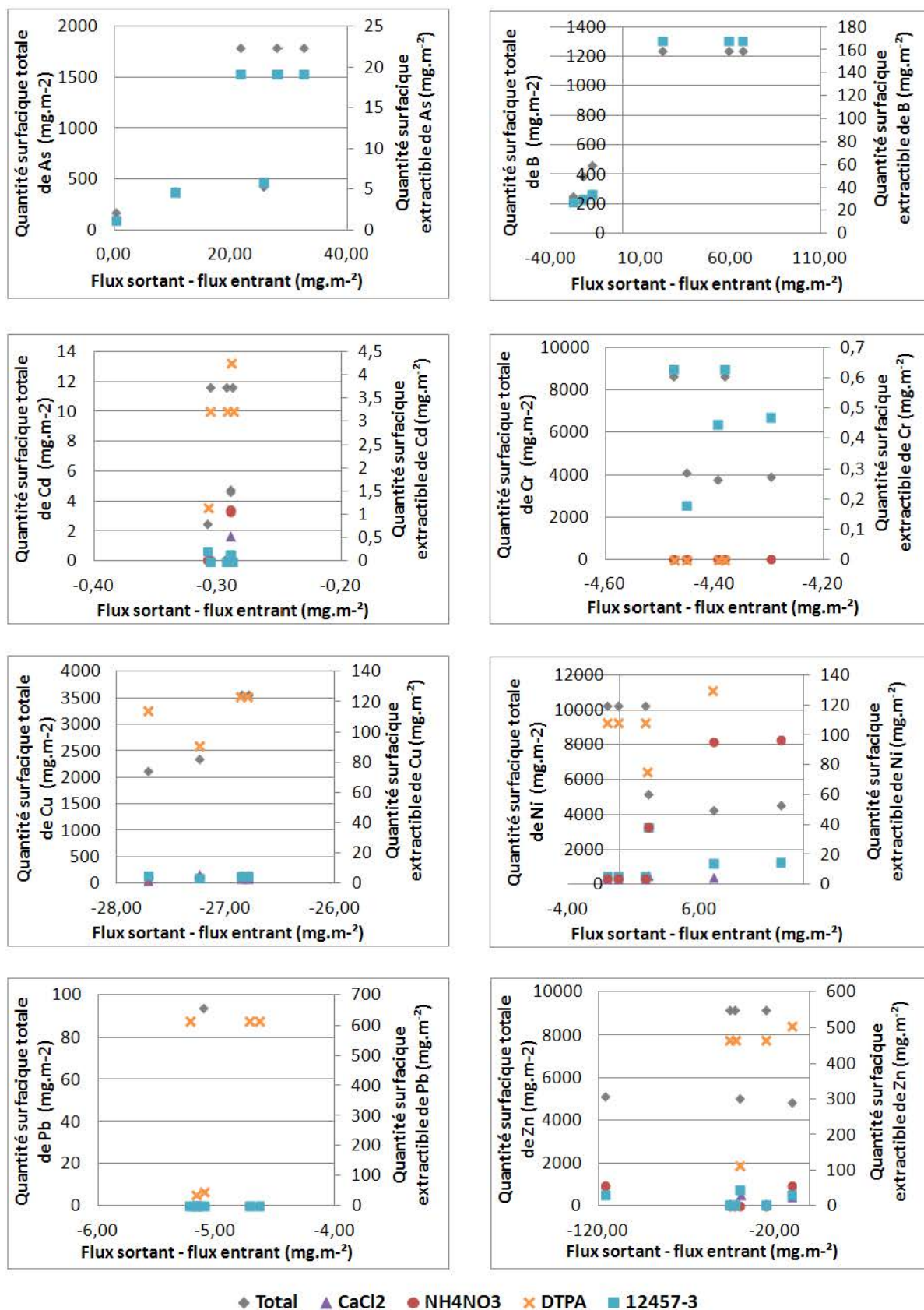
Figure 85 - Corrélations entre les différences de flux sortie-entrée et les quantités d'ETM totales et extractibles dans les différentes structures végétalisées
