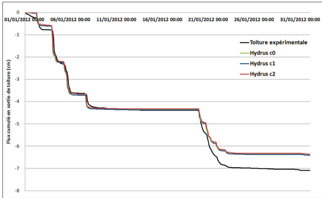
Figure 89 : Comparaisons des flux cumulés à l'exutoire pour différents modèles en janvier 2012
