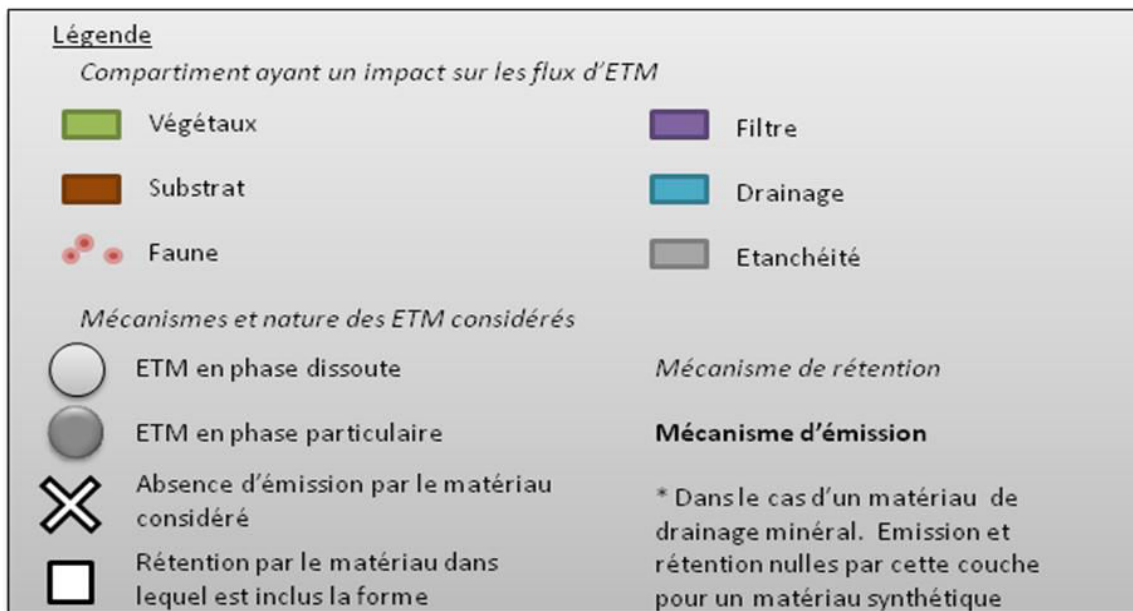
Figure 86 - Schéma récapitulatif des principaux mécanismes induisant une rétention et une émission d'ETM au sein d'une structure de toiture végétalisée
