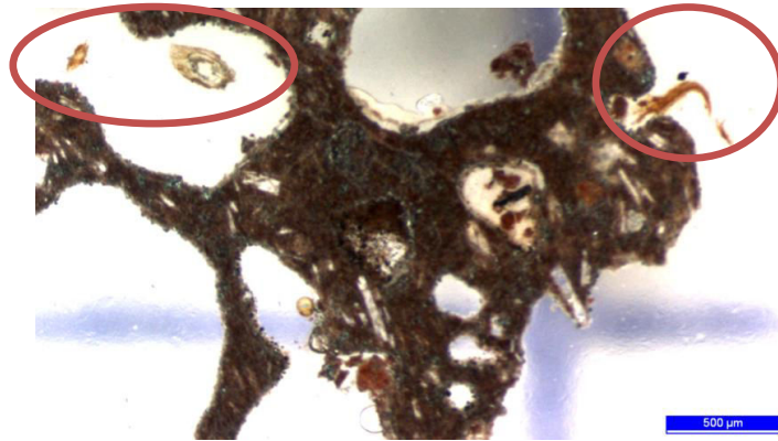
Figure 67 - Racines de S. floriferum introduites dans les porosités d'un grain de pouzzolane (point de prélèvement 2)
