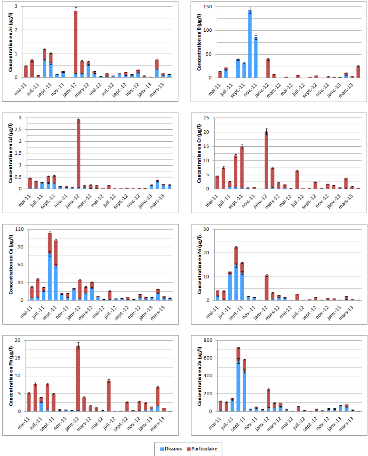
Figure 36 - Concentrations en ETM en phases dissoutes et particulaires dans les dépôts atmosphériques sur la période de suivi des toitures végétalisées expérimentales
