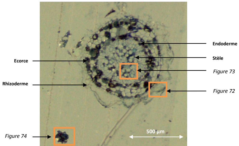
Figure 71 – Structure primaire d’une racine de S. spurium observée à la loupe binoculaire
