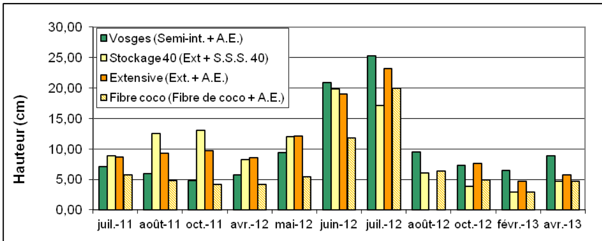
Figure 44 - Evolution de la hauteur moyenne des plants de S. reflexum germanium selon les associations de substrats et drainages de juillet 2011 à avril 2013
