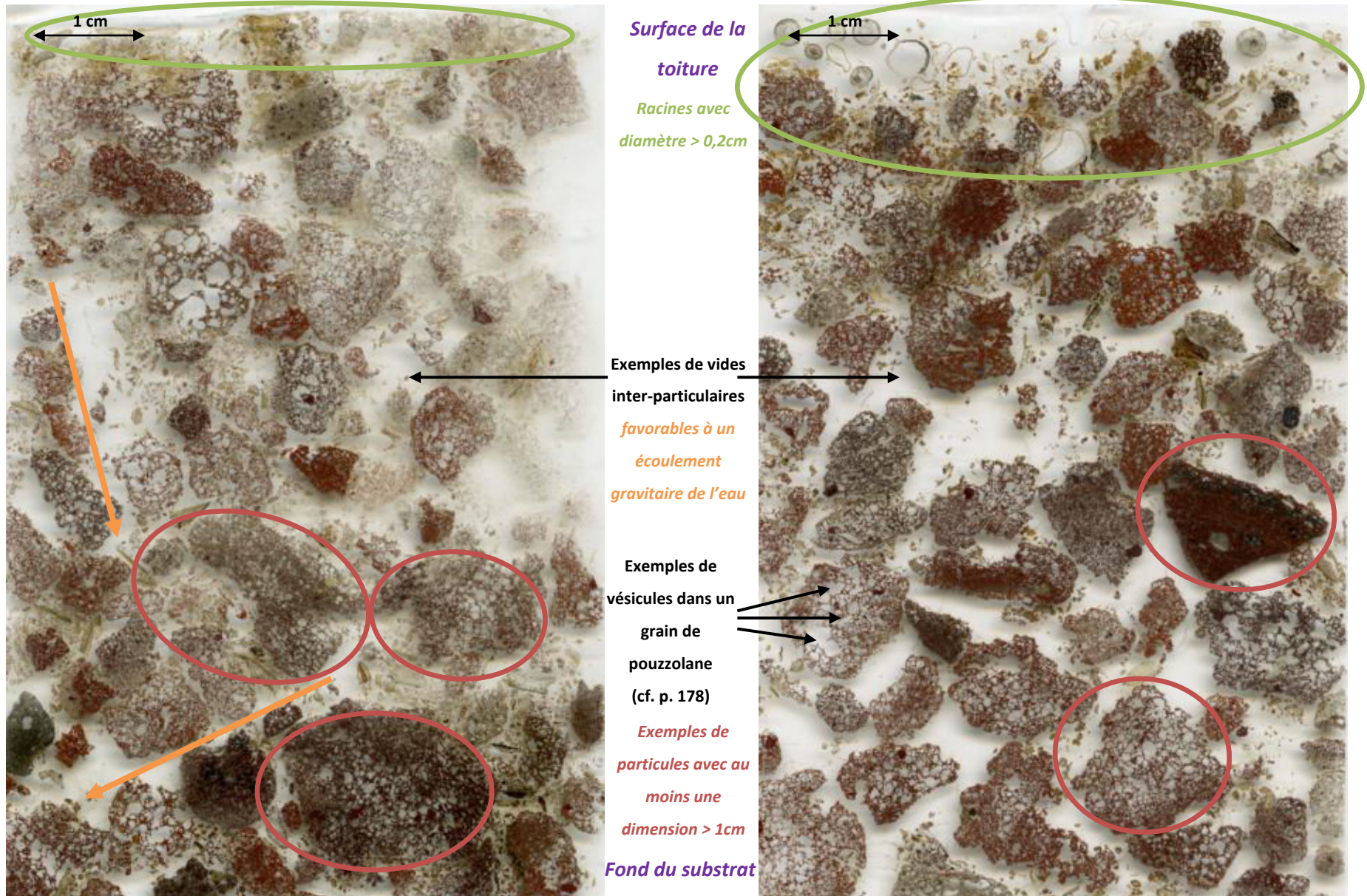
Figure 59 - Lames minces de substrat extensif prélevées aux points de prélèvement 3 ( S. album ) et 4 ( S. reflexum ) sur la toiture Extensive
