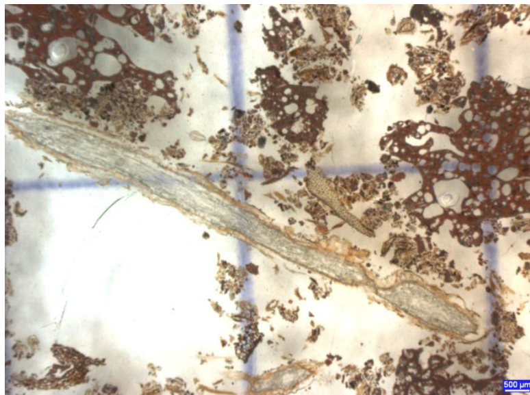
Figure 66 – Agrégation et accumulation de particules au-dessus de racines de S. spurium (haut) et S. floriferum (bas) (points de prélèvement 1 et 2)
