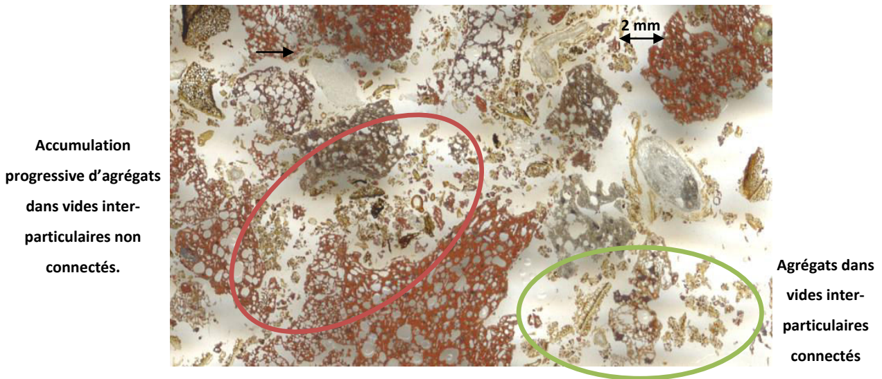
Figure 63 - Formation d'agrégats dans des vides inter-particulaires (point de prélèvement 2)
