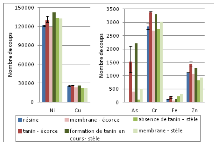
Figure 75 – Evaluation de la quantité d'ETM présents par sonde EDX dans les différents tissus racinaires de S. spurium
