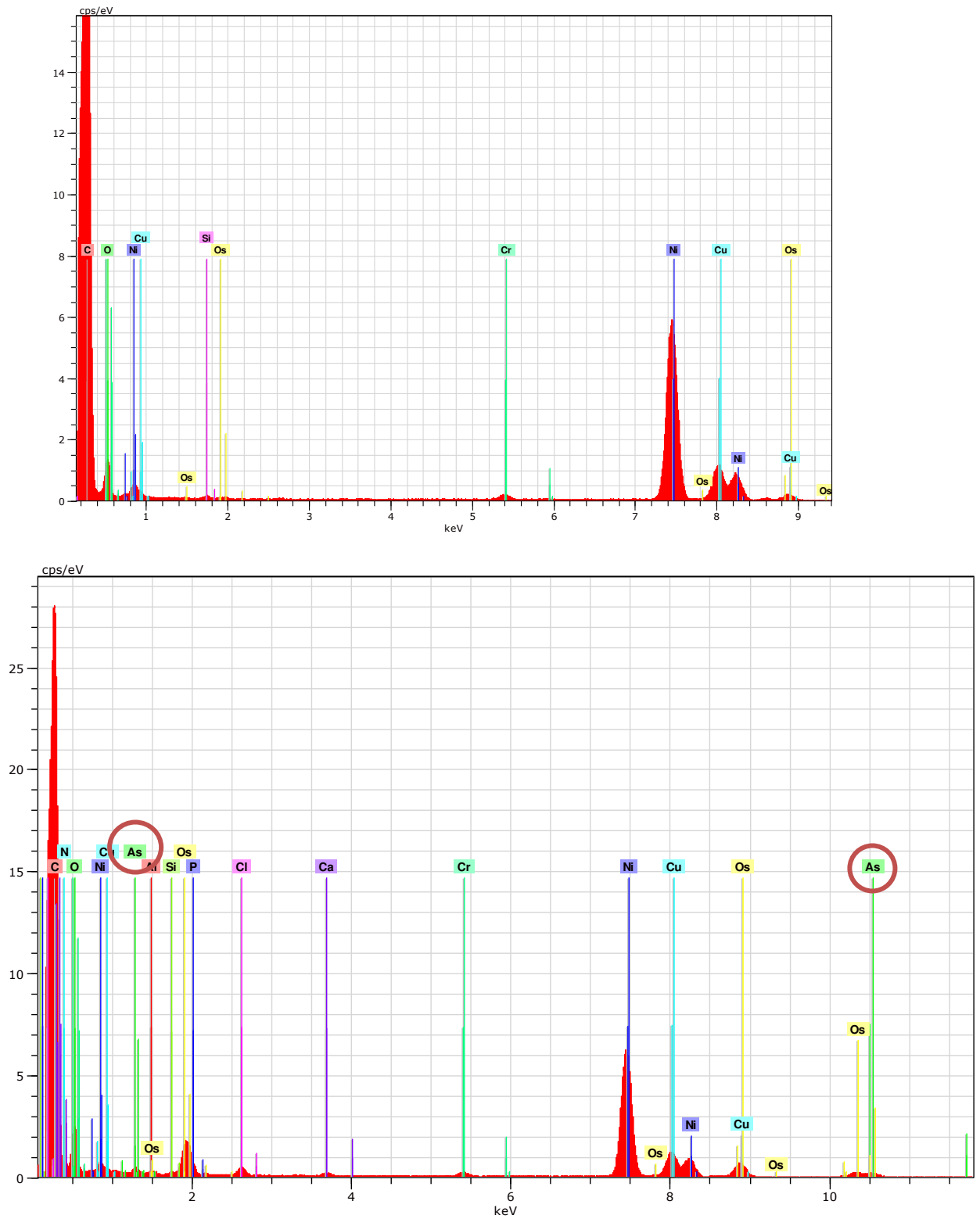
Figure 76 - Spectres obtenus par analyse élémentaire par EDX dans différentes zones de la lame de S. spurium (résine témoin en haut, cellule contenant un complexe polyphénolprotéines en bas)
