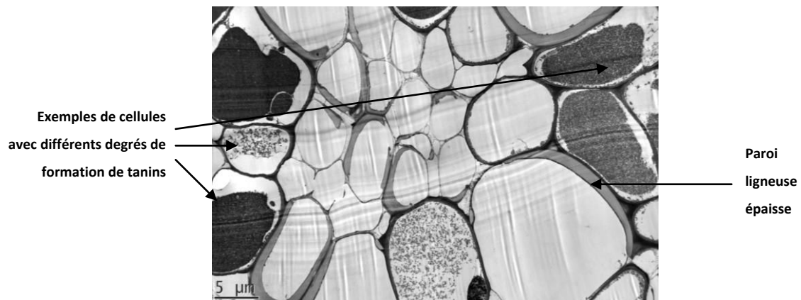
Figure 73 - Cellules du stèle. Observation au MET d’une coupe transversale de S. spurium
