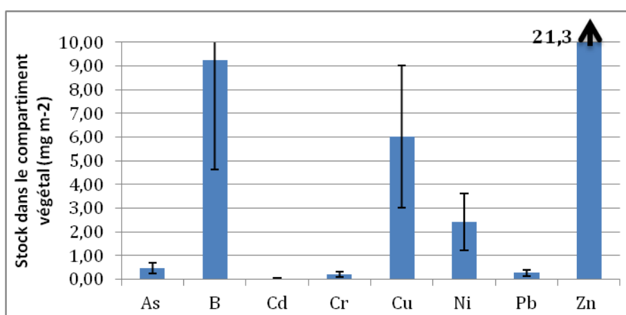
Figure 84 - Teneurs en ETM dans le compartiment végétal de la toiture extensive en avril 2013
