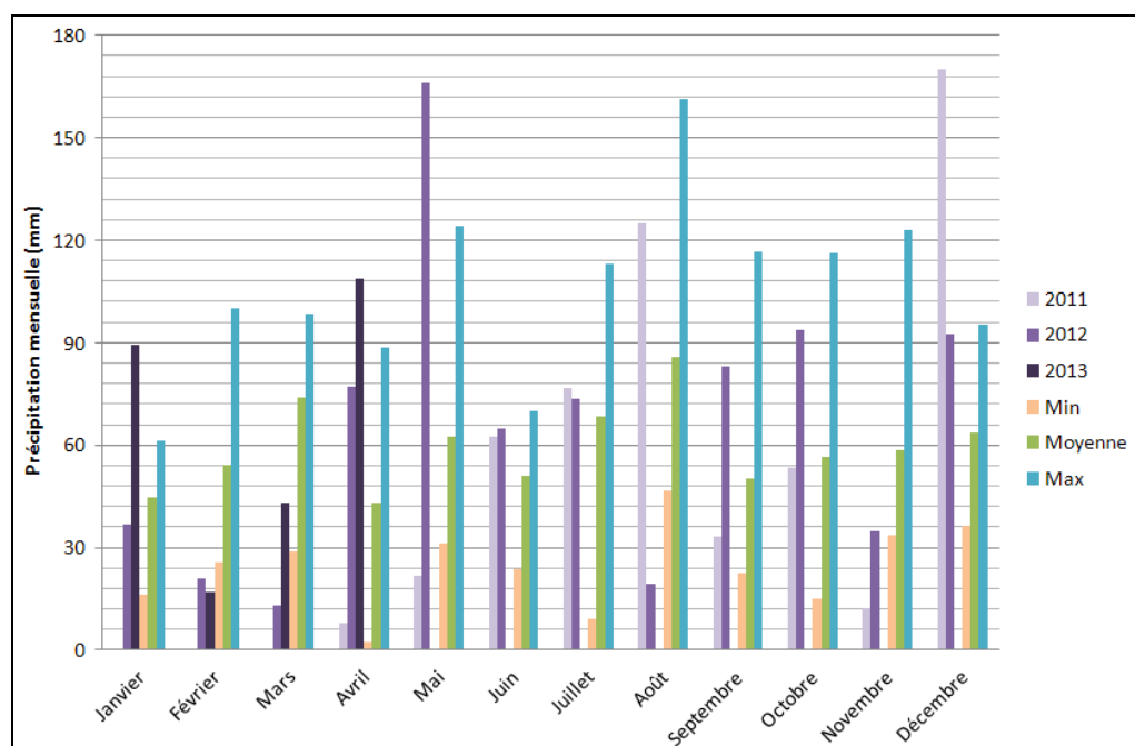
Figure 35 - Pluviométrie mensuelle d'avril 2011 à avril 2013 et comparaison avec les minimums, moyennes et maximums mensuels de 2005 à 2009
