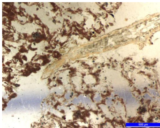
Figure 68 - Racine de S. floriferum introduite entre deux grains de pouzzolane probablement en contact au préalable (point de prélèvement 2)
