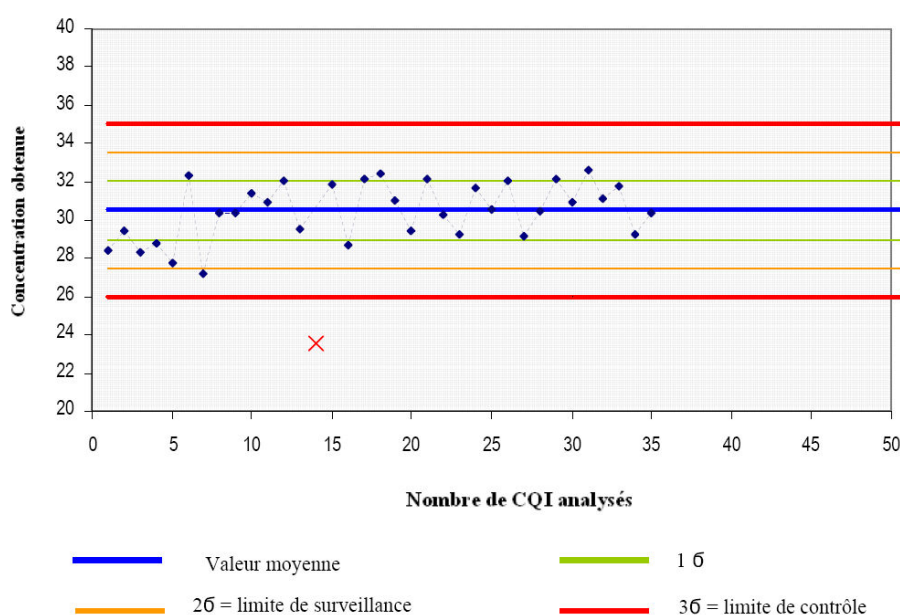
Figure 16 - Exemple d'une carte de contrôle établie à l'aide des CQI. Source : Lamprea, 2009
