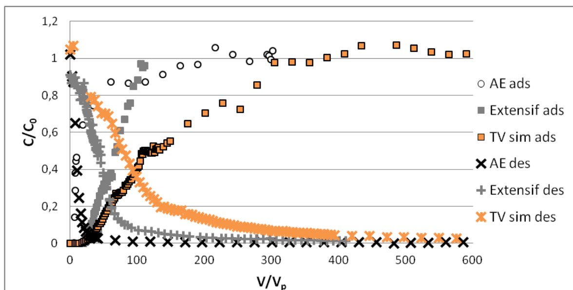
Figure 34- Comparisons des courbes de sorption et désorption des différents matériaux en fonction de V/V_p
