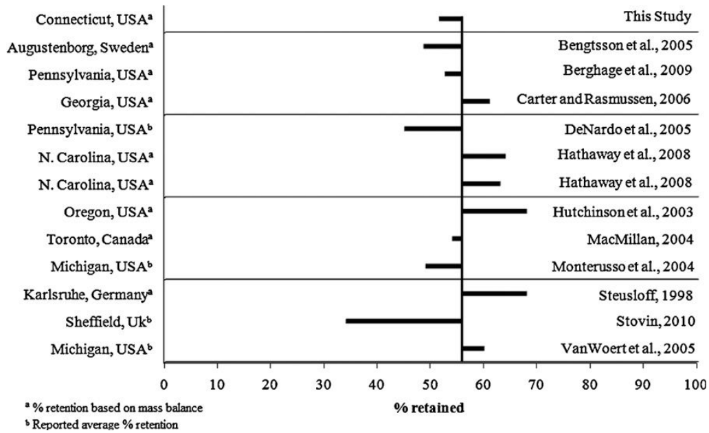
Figure 7 - Analyses des volumes de pluie retenus recensés dans le cadre de différentes études de toitures végétalisées. Source : Gregoire & Clausen, 2011
