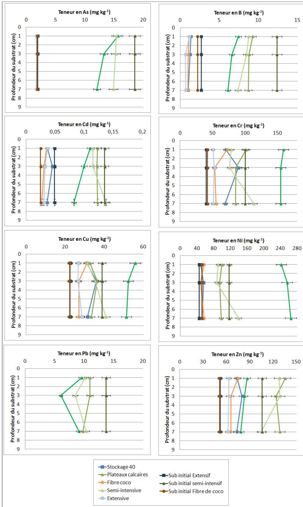
Figure 51 - Evolutions des teneurs en ETM sur les profils de substrat des parcelles expérimentales
