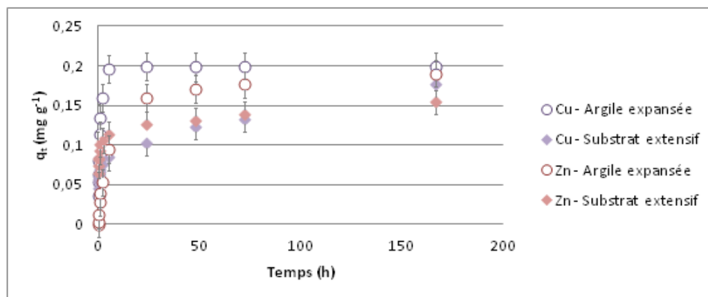
Figure 27 - Evolution de la quantité de Cu et Zn sorbée au cours du temps sur l'argile expansée et le substrat extensif non concassé
