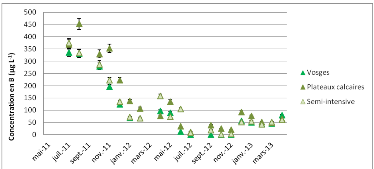
Figure 38 – Diminution des concentrations totales en B en sortie des toitures végétalisées Vosges, Plateaux calcaires et Semi-intensive entre mai 2011 et avril 2013
