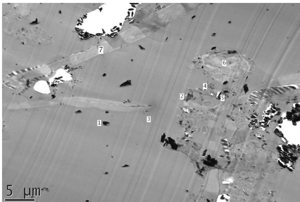
Figure 79- Observation au MET d'une lame de substrat extensif et emplacement des mesures à la sonde EDX
