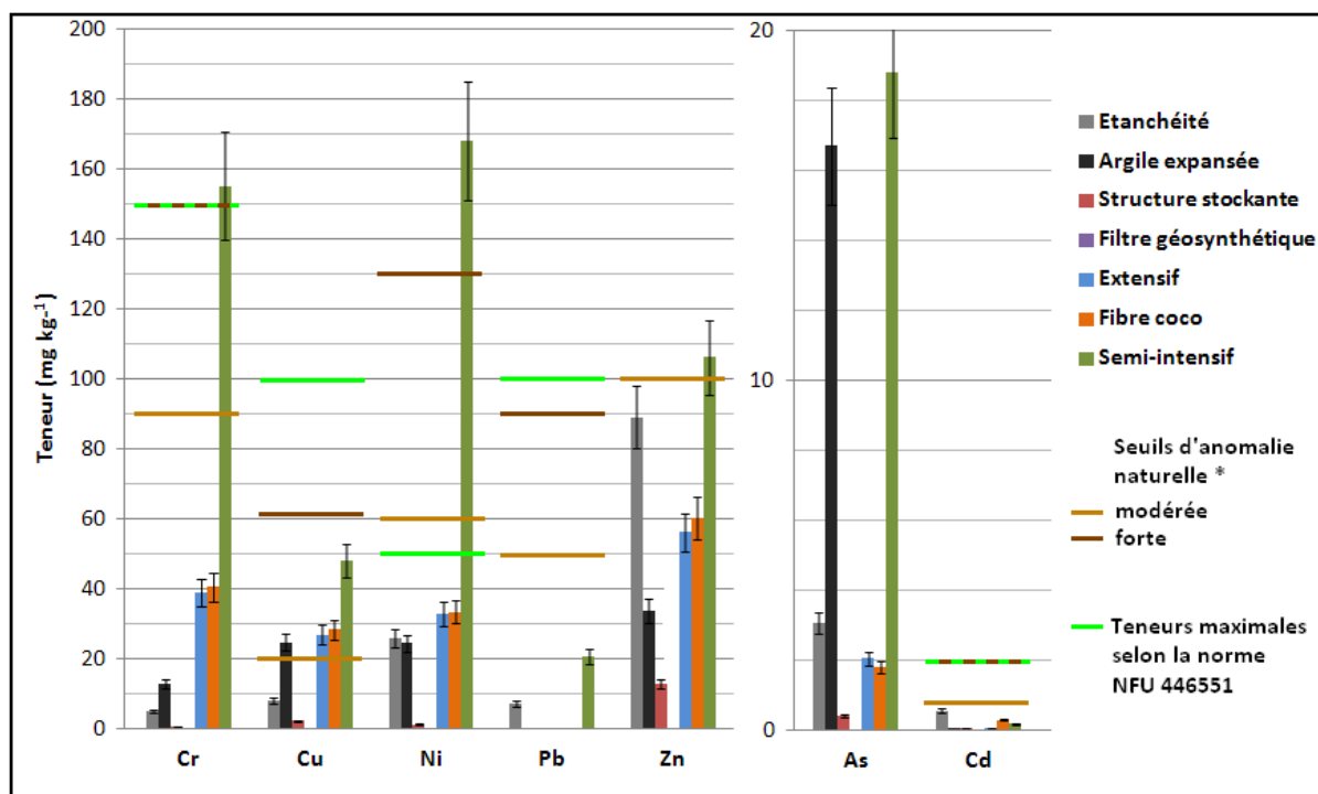
Figure 22 - Teneurs initiales en ETM dans les différents matériaux constitutifs des toitures végétalisées comparées à des seuils d'anomalie naturelle et une norme relative aux supports de culture (*Baize, 2000)
