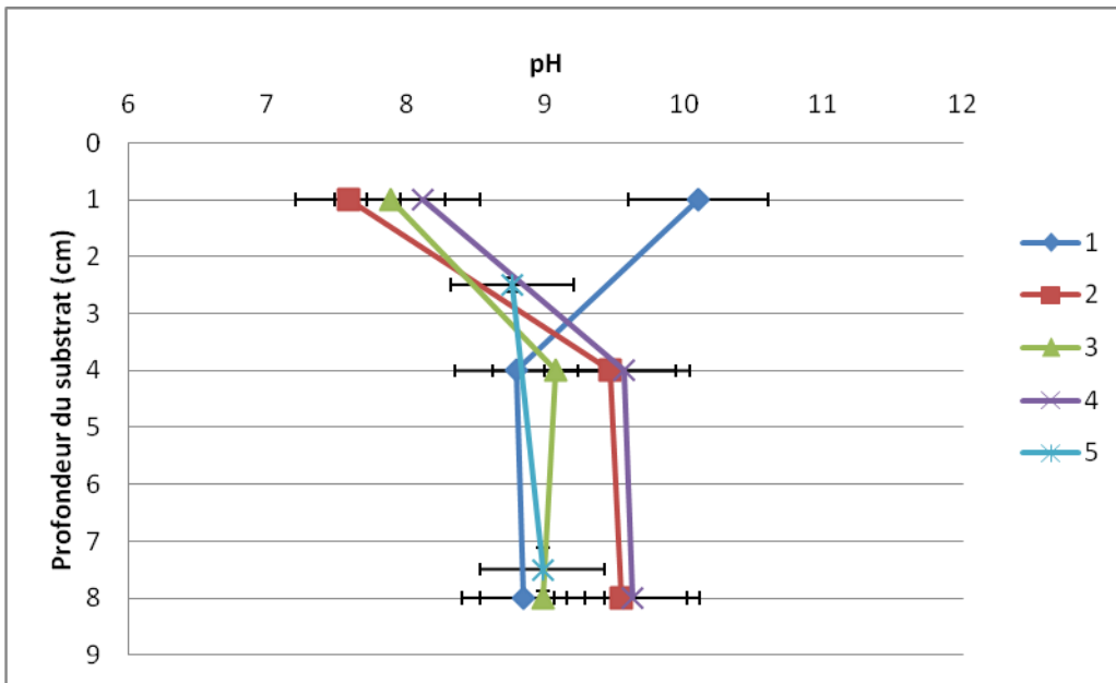
Figure 55 - Variabilité du pH entre les différents points de prélèvements sur la toiture Extensive
