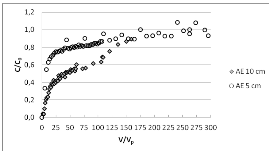
Figure 32 - Impact de la hauteur d'argile expansée sur la courbe de percée de Zn
