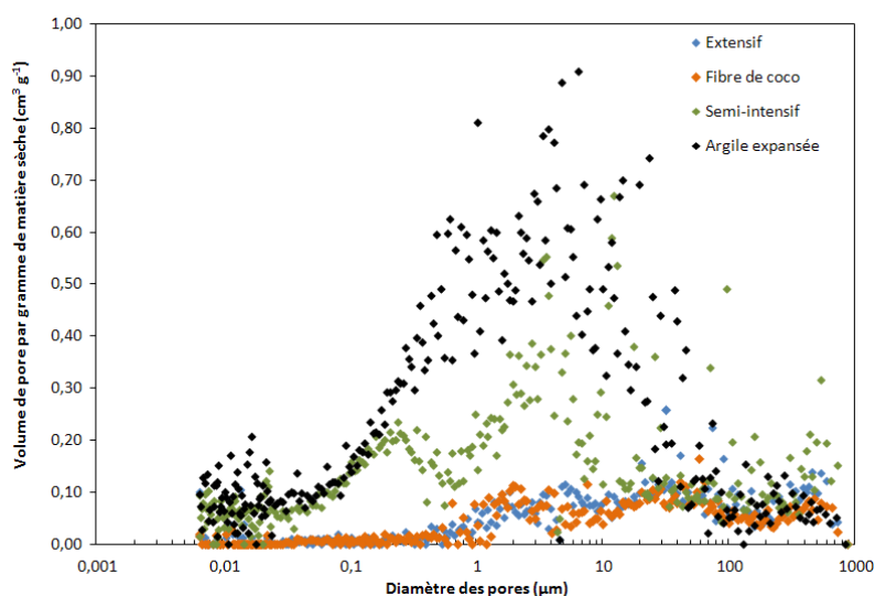
Figure 21 – Répartition du nombre de pores en fonction de leur diamètre dans les trois substrats et l'argile expansée par analyse de la porosité au mercure
