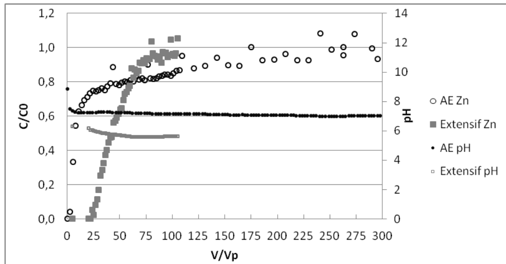
Figure 30 - Evolution de C/C_0 pour le Zn et du pH par rapport à V/V_p pour l'argile expansée et le substrat extensif en configuration similaire au ratio de hauteur des toitures végétalisées expérimentales
