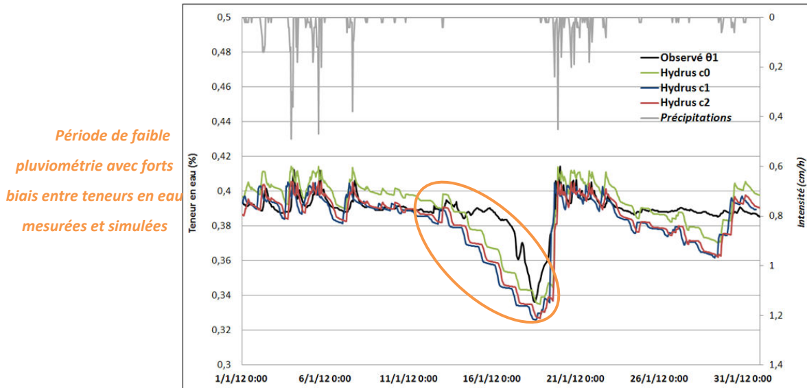
Figure 88 : Comparaisons des teneurs en eau observées et simulées via différents modèles avec le logiciel HYDRUS-1D sur janvier 2012
