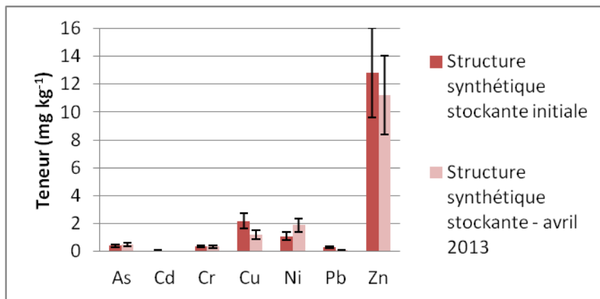
Figure 53 - Evolution des teneurs en ETM dans la structure synthétique stockante entre le matériau initial et celui prélevé en avril 2013
