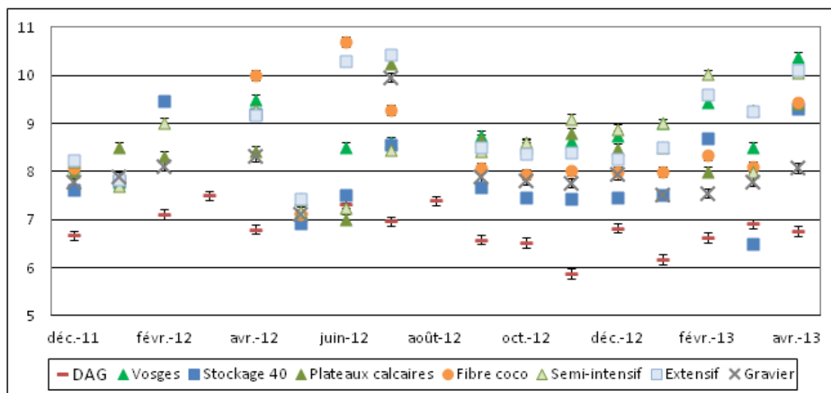
Figure 37 - Evolution du pH en entrée et sortie de toitures entre décembre 2011 et avril 2013
