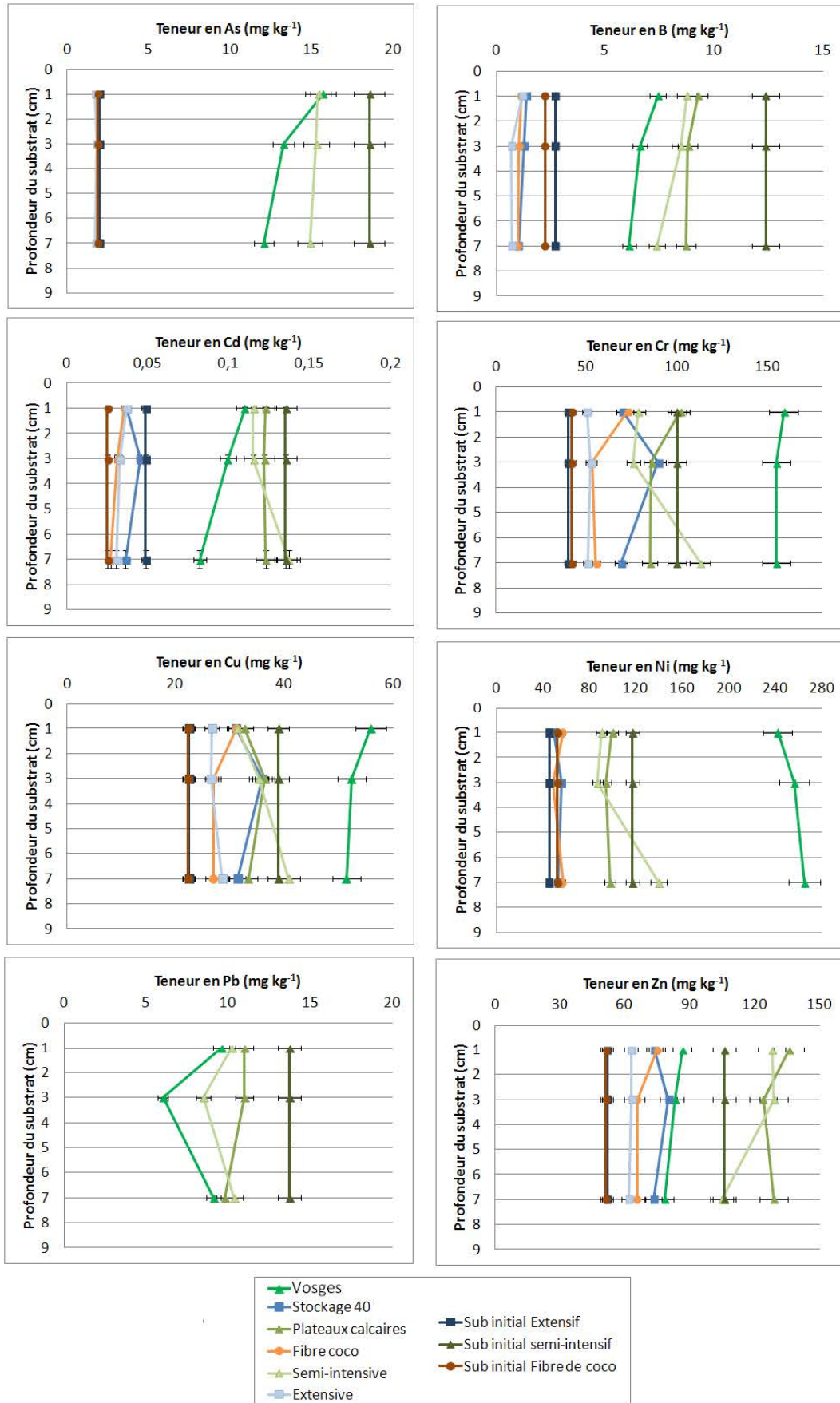
Figure 48 - Evolution des paramètres globaux sur les profils des différentes toitures végétalisées entre octobre 2010 et avril 2013
