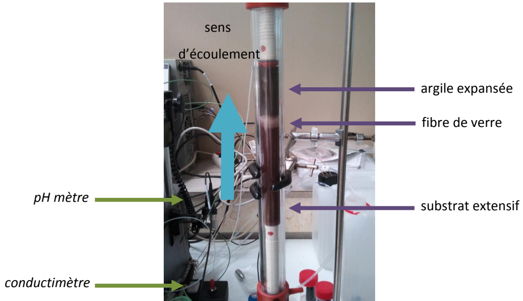
Figure 17- Photo de la colonne dans le cadre de l'essai de sorption de Zn TV sim
