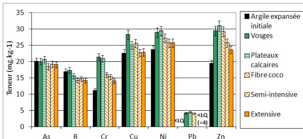
Figure 54 - Evolution des teneurs en ETM dans les couches de drainage constituées d'argile expansée
