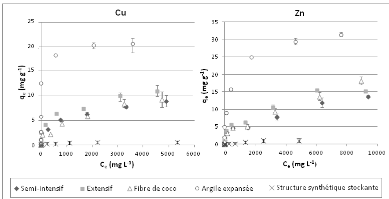
Figure 25 - Evolution de la sorption de Cu et Zn sur les trois substrats et les deux drainages en fonction de la concentration à l'équilibre
