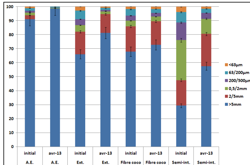
Figure 49 - Evolution de la répartition granulométrique entre octobre 2010 et avril 2011 dans les substrats et l'argile expansée
