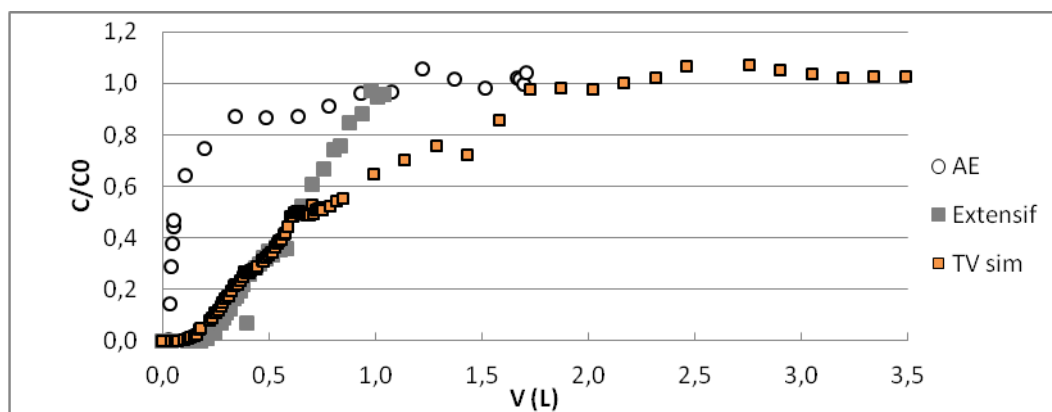
Figure 33 - Impacts de la superposition du substrat et de l'argile expansée sur l'évolution du rapport C/C_0 en fonction du volume écoulé
