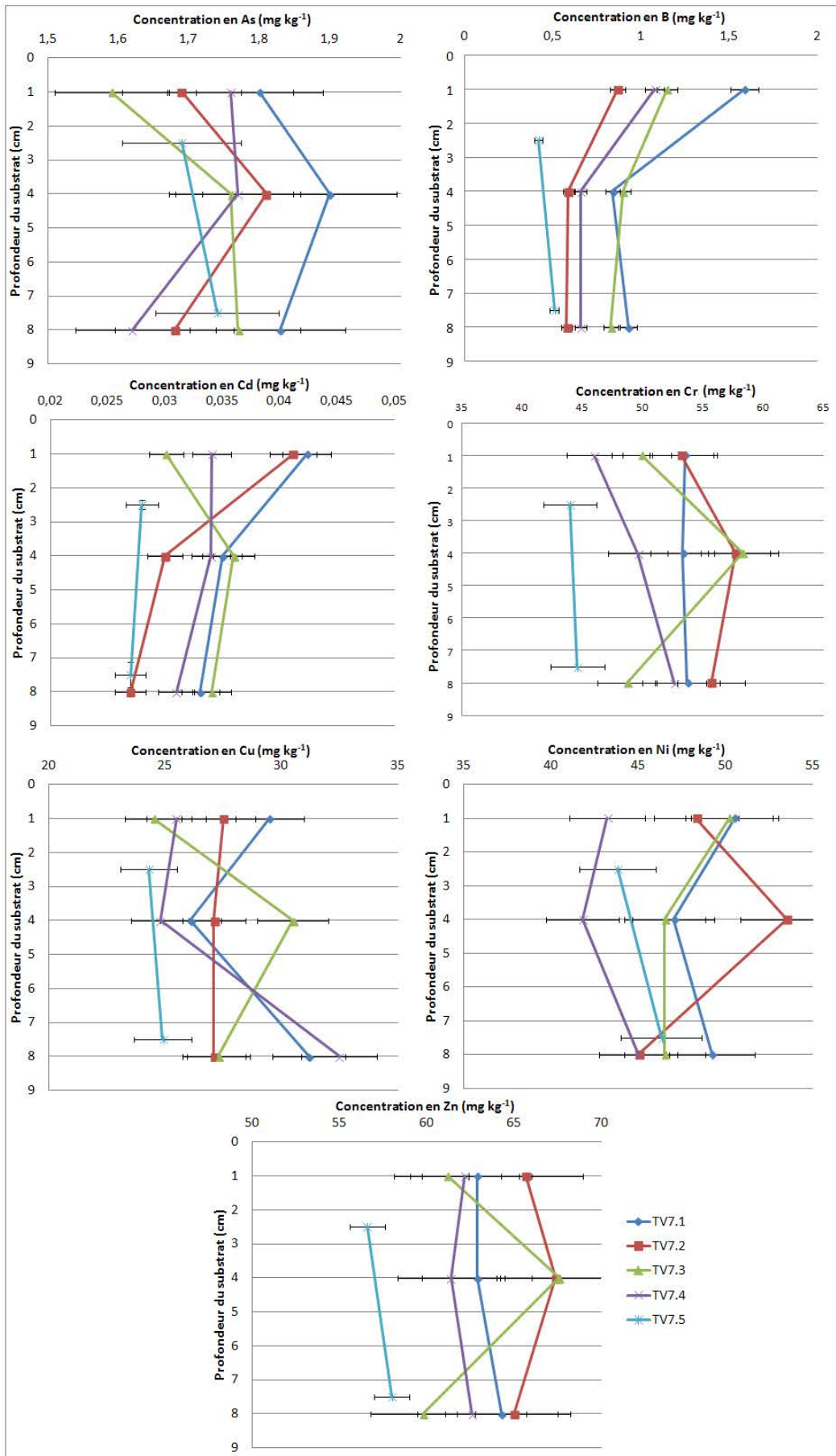
Figure 57 - Variabilité des teneurs en ETM entre les différents points de prélèvements sur la toiture Extensive
