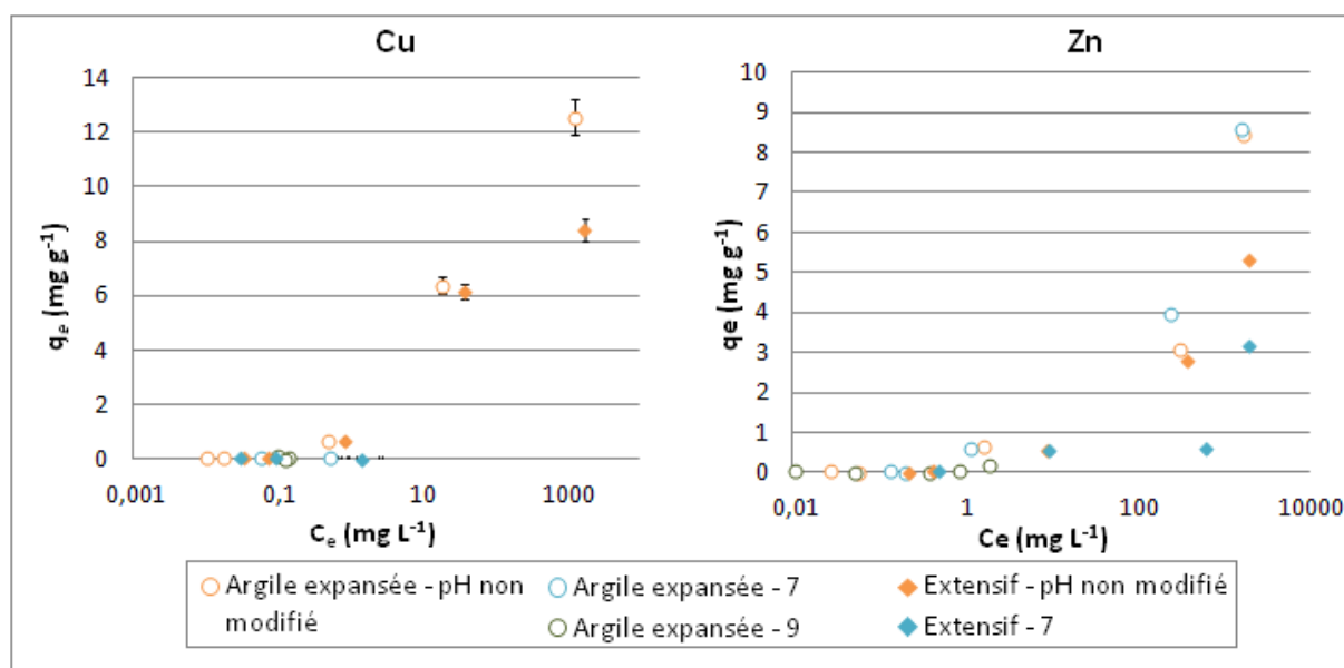
Figure 28 - Evolution de la capacité de sorption pour Cu et Zn de l'argile expansée et du substrat extensif non concassé en fonction de la concentration à l'équilibre à différents pH
