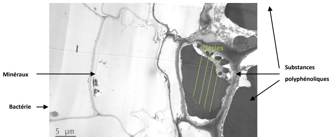
Figure 72 - Cellule périphérique et écorce de S. spurium observées au MET
