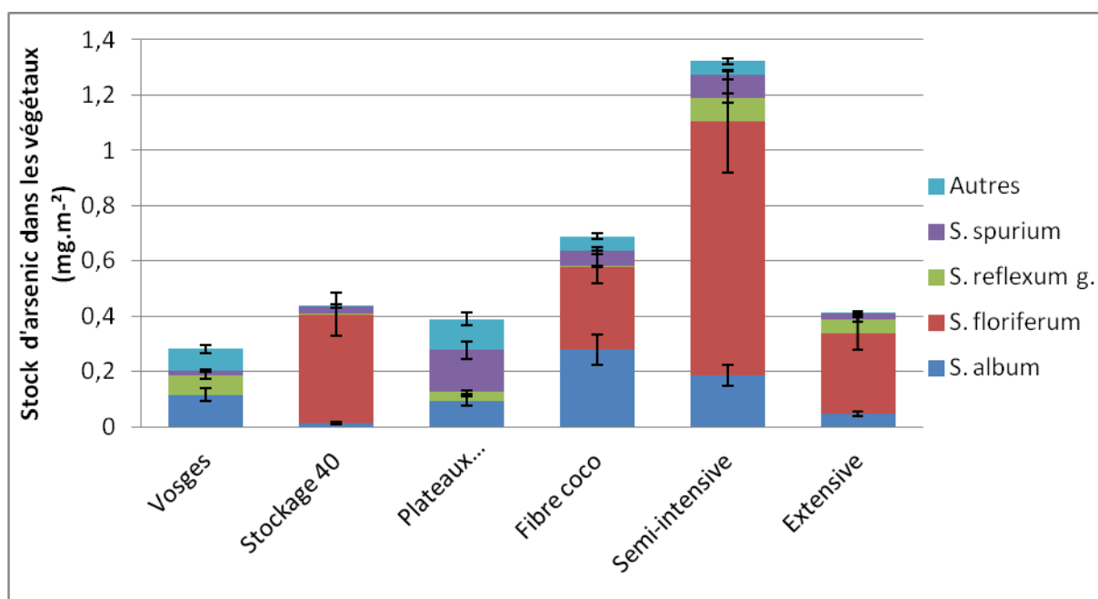
Figure 83 - Estimation du stock d'arsenic par parcelle végétalisée réparti entre les principales espèces présentes
