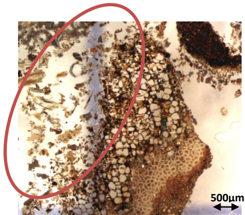
Figure 60 – Dégradation progressive et hétérogène de la matière organique initialement présente dans le substrat (point de prélèvement 2)
