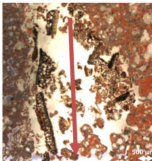
Figure 65- Orientation de particules dans un vide inter-particulaire pouvant indiquer un lessivage de celles-ci (point de prélèvement 3)
