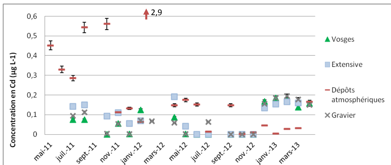
Figure 40 - Comparisons des concentrations totales en cadmium dans les dépôts atmosphériques et les eaux en sortie des toitures Vosges, Extensive et Graviers
