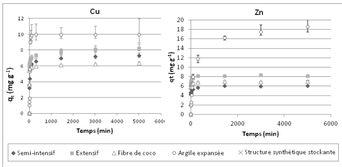
Figure 26 - Evolution de la sorption de Cu et Zn sur les trois substrats et l'argile expansée au cours du temps
