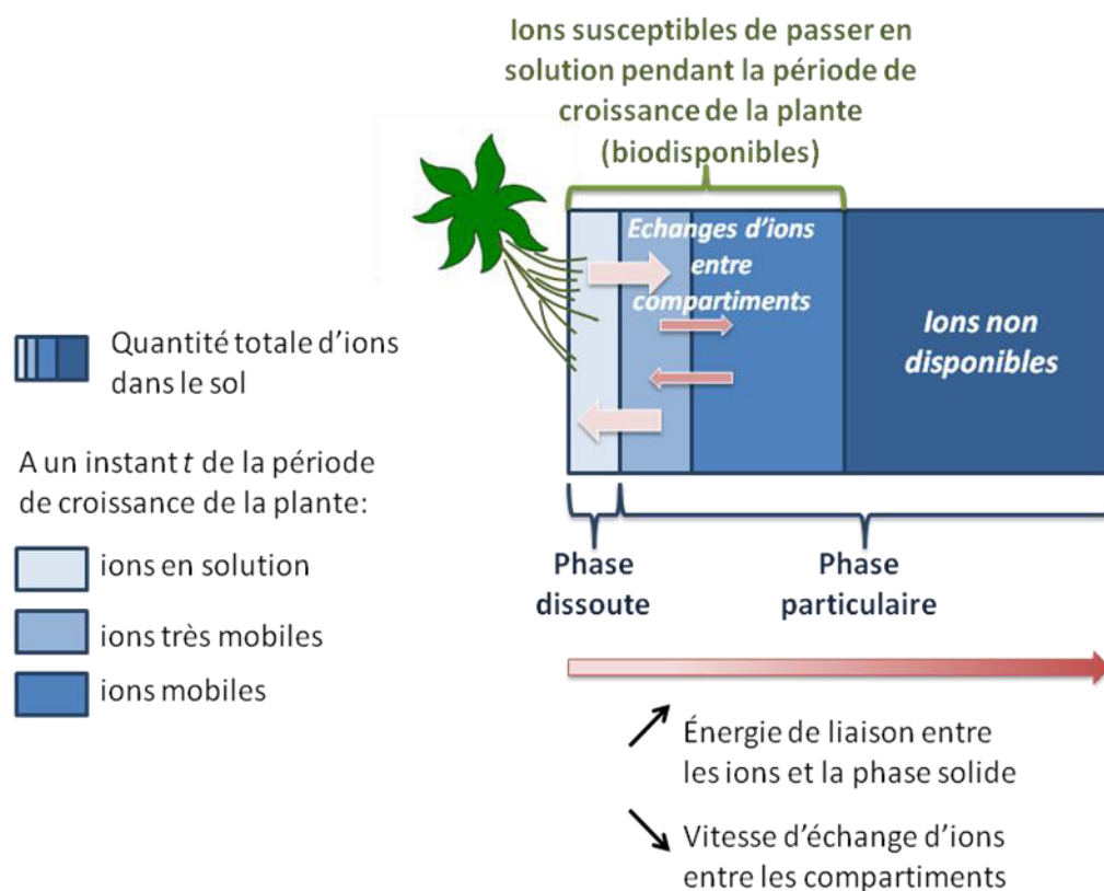
Figure 3 – Répartition et évolution de la biodisponibilité des ions dans le sol au cours de la période de croissance de la plante. Adapté de Morel (1997 a et b)
