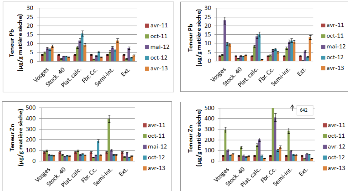
Figure 46.c – Evolution des teneurs en ETM dans les S.album et reflexum g. sur les différentes parcelles végétalisées d'avril 2011 à avril 2013
