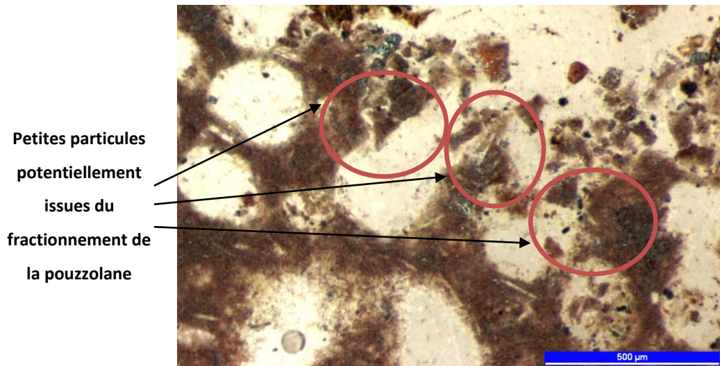
Figure 64 - Observation à plus fort zoom des agrégats et de leurs associations avec la surface de la pouzzolane (point de prélèvement 4)
