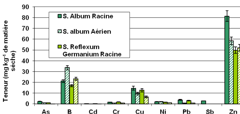
Figure 20 - Comparaison des teneurs initiales en ETM dans S. album et S. reflexum g.
