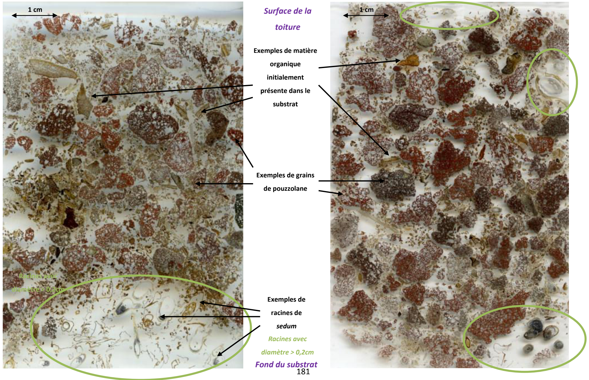
Figure 58 - Lames minces de substrat extensif prélevées aux points de prélèvements 1 ( S. spurium ) et 2 ( S. floriferum ) sur la toiture Extensive
