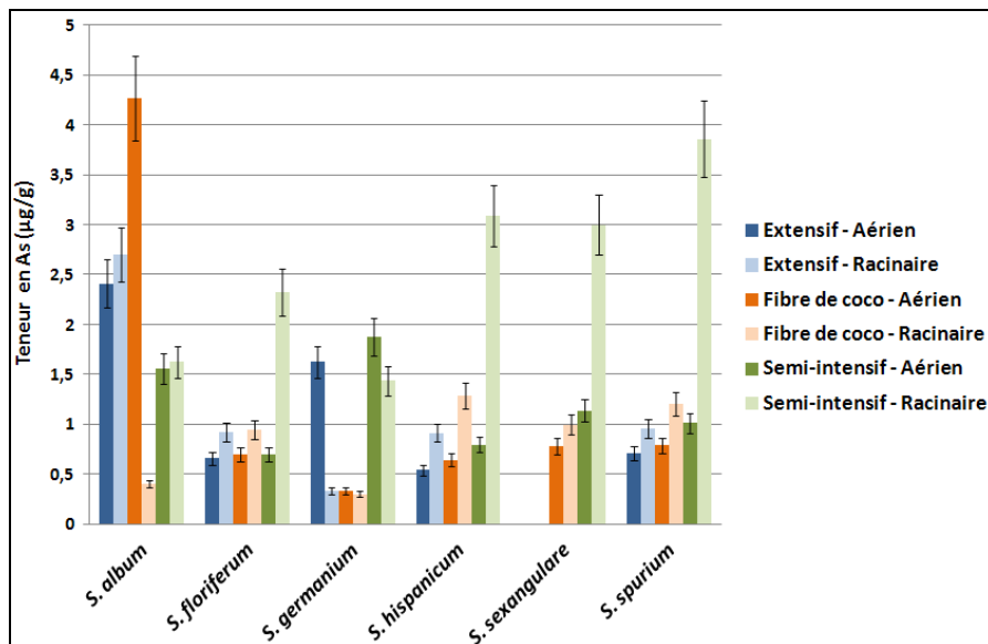
Figure 47 - Teneurs moyennes en As dans les principaux végétaux présents sur les toitures en avril 2013 selon les substrats
