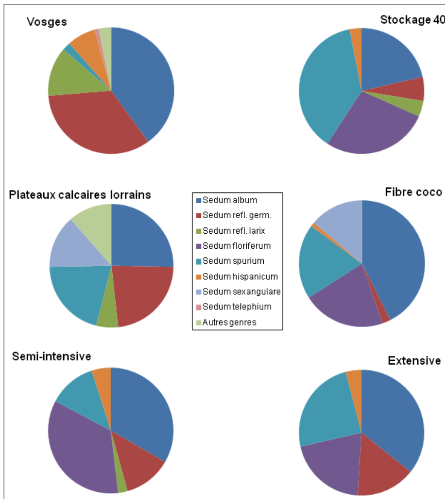
Figure 43 - Part des différents végétaux dans le recouvrement des toitures végétalisées en avril 2013
