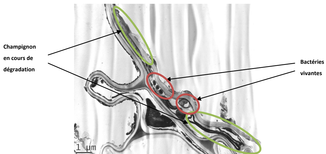
Figure 80 - Micro-organismes présents dans les cellules externes de la racine de S. spurium
