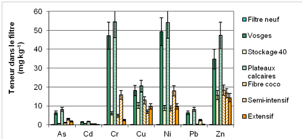
Figure 52 - Evolution des teneurs en ETM dans le filtre géosynthétique
