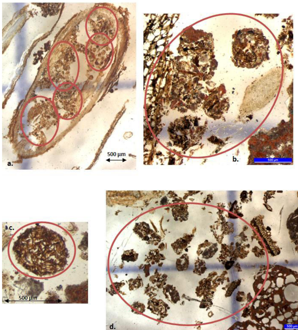
Figure 70 – Exemples de boulettes fécales de diamètre proche de 125 \mu\text{m} dans une racine morte de S. spurium (a) et de l'ordre de 500 \mu\text{m} dans les vides interparticulaires (b, c, d) (points 2 et 3)
