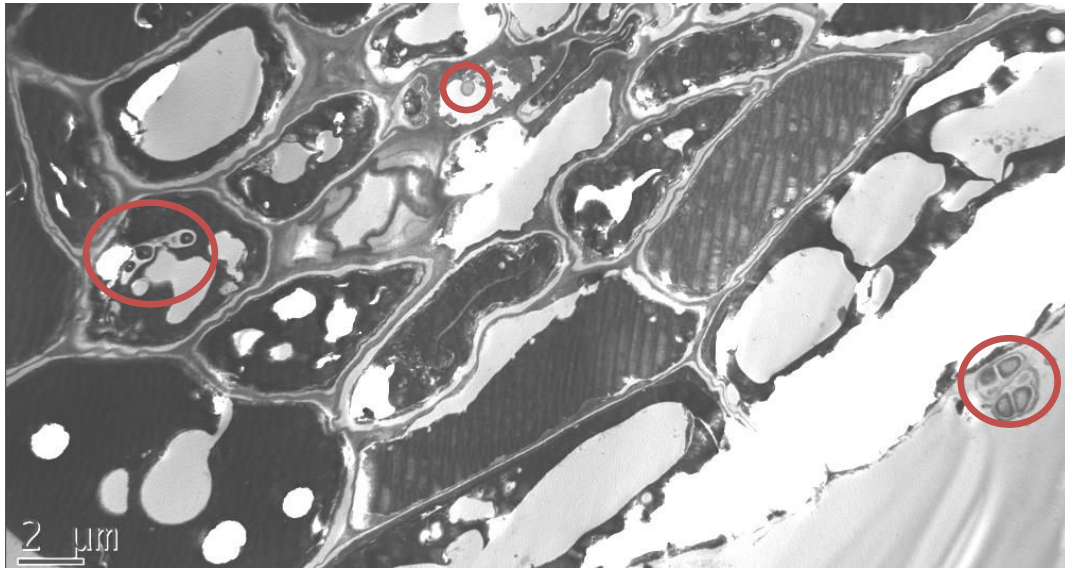
Figure 81 - Bactéries présentes autour et dans la racine dégradée de S. spurium
