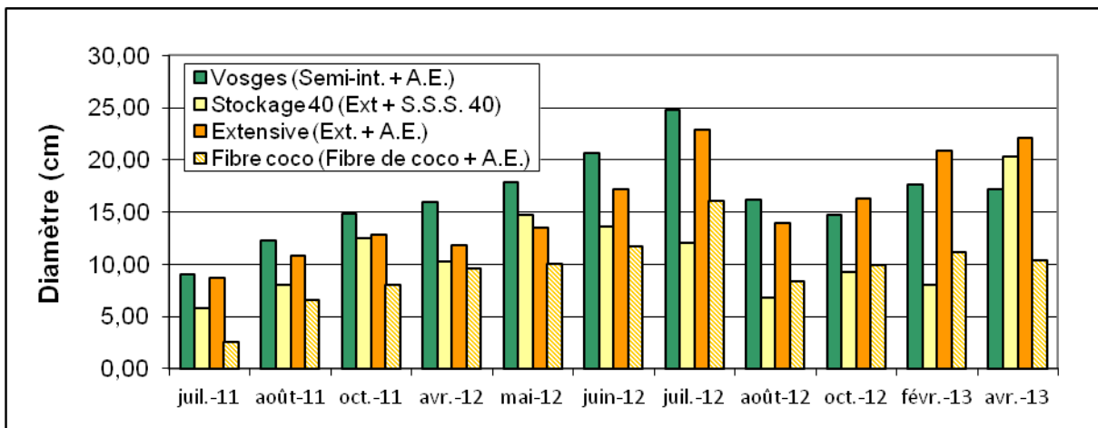
Figure 45 - Evolution du diamètre moyen des plants de S. reflexum germanium selon les associations de substrats et drainages de juillet 2011 à avril 2013
