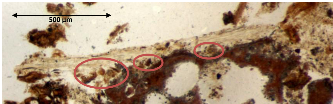
Figure 69 - Racine de S. floriferum en contact direct avec un grain de pouzzolane semblant induire un fractionnement de petites particules de pouzzolane dans la zone de contact (point de prélèvement 2)
