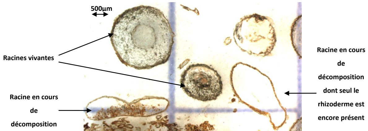
Figure 61 - Racines de S. reflexum vivantes et mortes avec différents stades d'avancement de dégradation (point de prélèvement 4)
