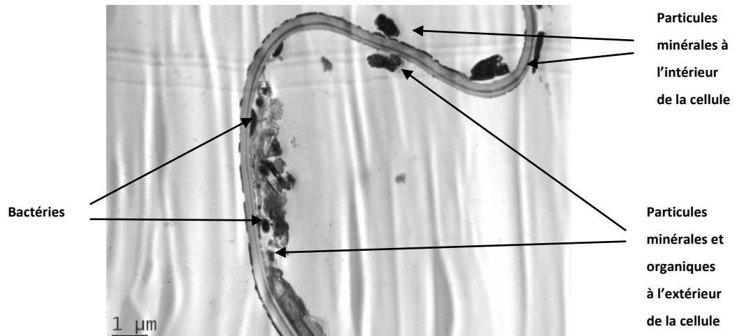
Figure 78- Adhésion de minéraux, de bactéries et de résidus organiques en surface et à l'intérieur des cellules externes de la racine de S. spurium
