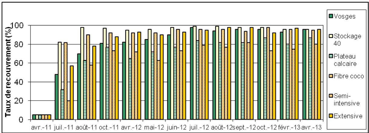
Figure 42 - Evolution du pourcentage de recouvrement par la végétation des différentes toitures d'avril 2011 à avril 2013
