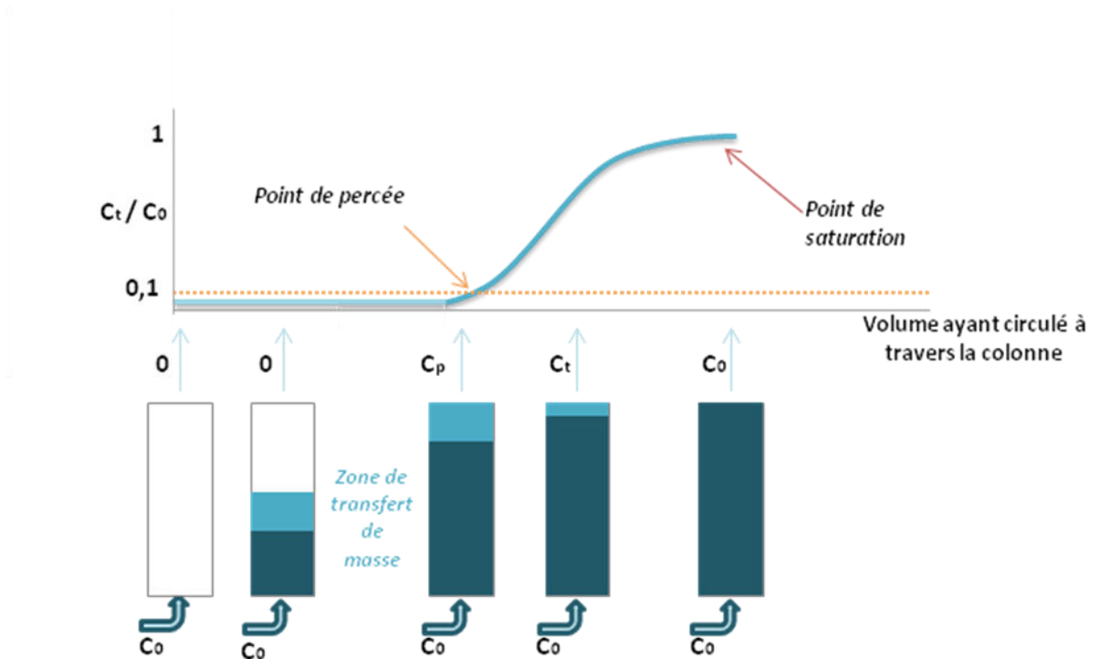
Figure 18 – Courbe de percée classique présentant les différentes étapes d'évolution des concentrations au sein de la colonne en fonction du volume écoulé à travers la colonne.
