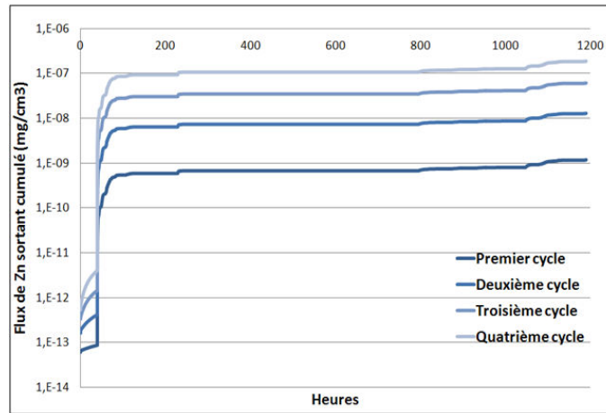
Figure 91 : Evolution des flux de zinc en sortie de toitures au fur et à mesure des cycles de simulation
