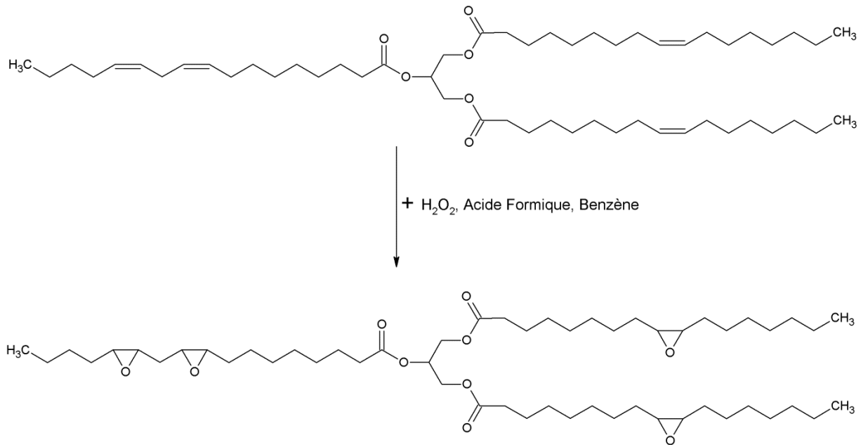
Figure 16 : Epoxydation des triglycérides
