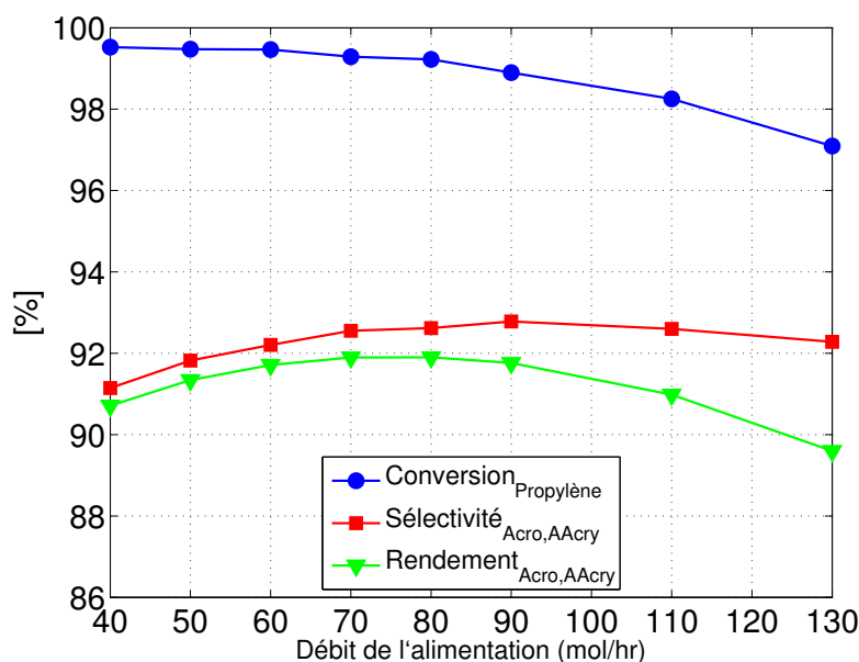
FIGURE 4.7 – Conversion du propylène, sélectivité totale d'acroléine et d'acide acrylique et rendement total en acroléine et en acide acrylique vs débit d'alimentation - Cas A1
