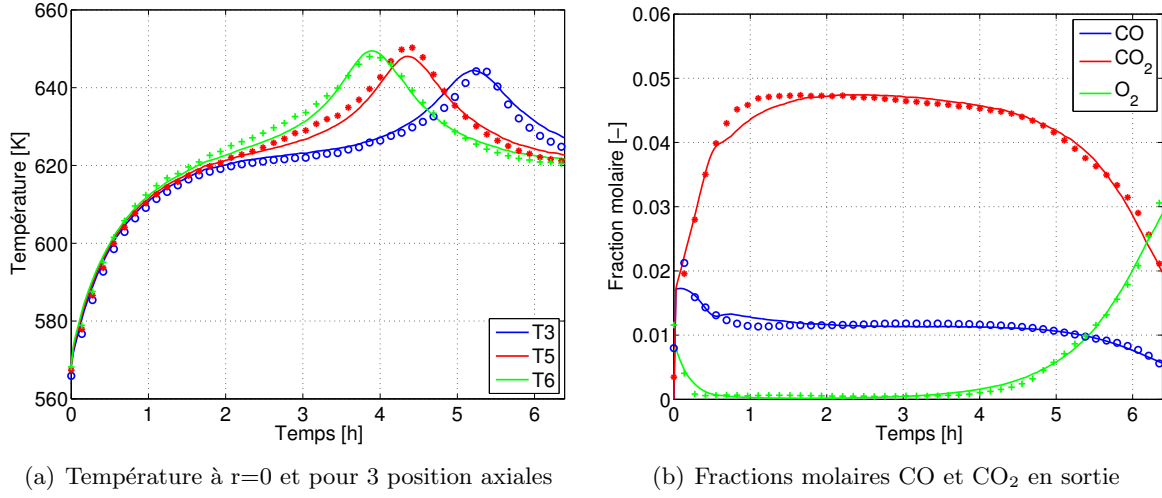
FIGURE 5.8 – Comparaisons entre les prédictions du modèle et les mesures expérimentales ( SF_161012 , modèle 3a)
