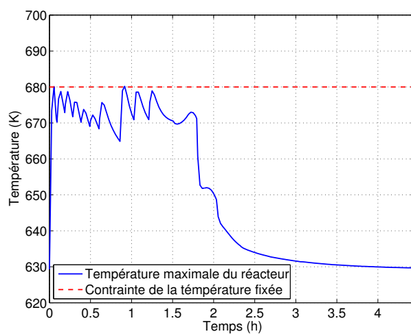
FIGURE 5.31 – Température maximale du réacteur (Cas B)
