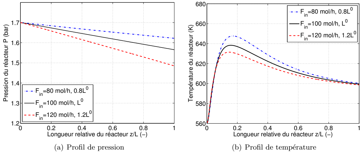
FIGURE 4.5 – Influence de la longueur du lit sur la perte de charge du lit(a) et le profil de température(b) pour la même VVH. ( P_{in}^0, T_c^0 )
