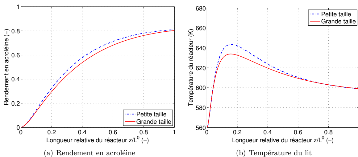
FIGURE 4.1 – Influence de la taille du catalyseur sur le rendement en acroléine (a) et sur le profil de température du lit (b) dans les conditions nominales de fonctionnement ( P_{in}^0, T_c^0, F_t^0, L^0 )
