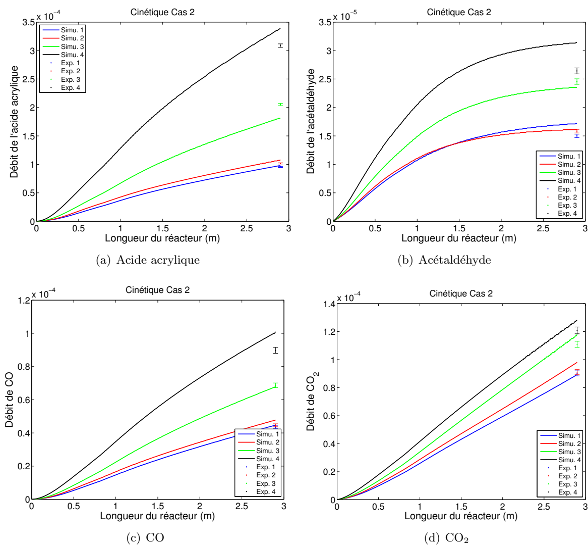
FIGURE 3.13 – Comparaison des débits des sous-produits mesurés à la sortie aux prédictions du modèle pour le réacteur à l'échelle du pilote – Modèle 1
