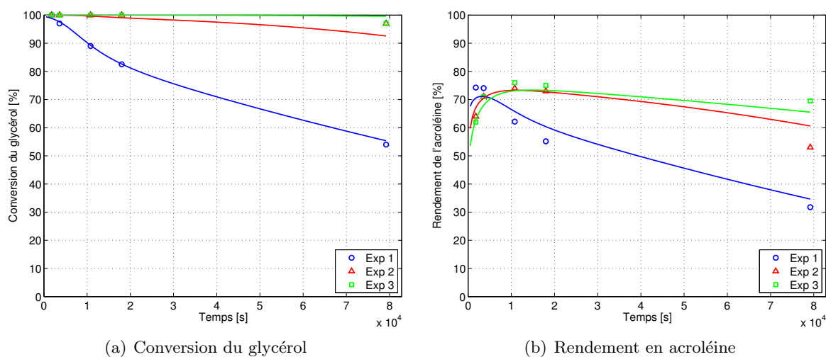
FIGURE 6.7 – Comparaison du taux de conversion du glycérol et du rendements en acroléine à trois différentes positions dans le réacteur (procédé avec catalyseur GHK22)
