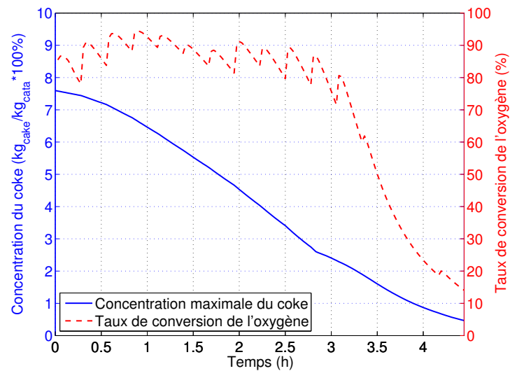
FIGURE 5.15 – Profils de la concentration maximale du coke et du taux de conversion de l’oxygène à la sortie en fonction du temps après optimisation.
