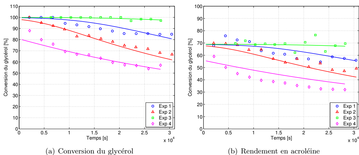
FIGURE 6.8 – Comparaison entre les prédictions du modèle et les mesures expérimentales au laboratoire pour la conversion du glycérol et le rendement en acroléine.
