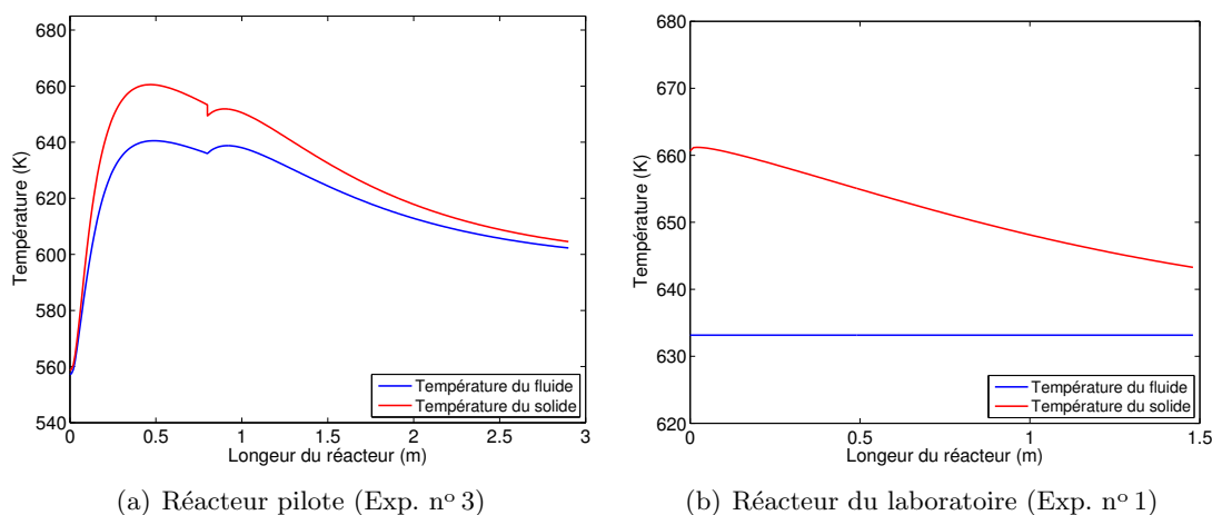
FIGURE 3.16 – Profils des températures du solide et du fluide dans les réacteurs pilote et du laboratoire – Modèle 2a
