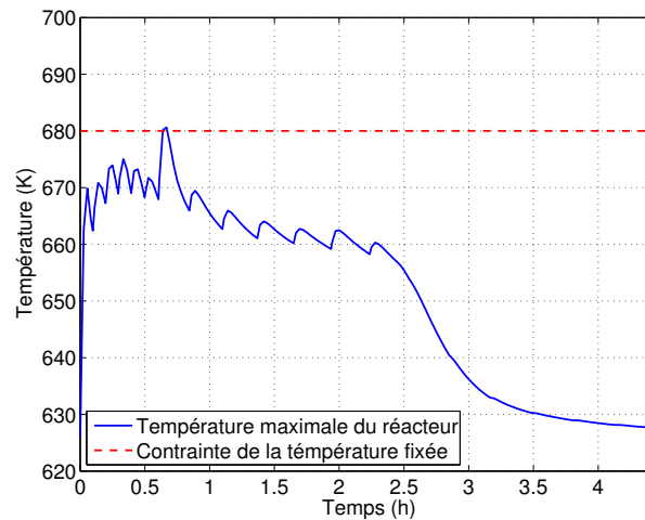
FIGURE 5.21 – Température maximale du réacteur
