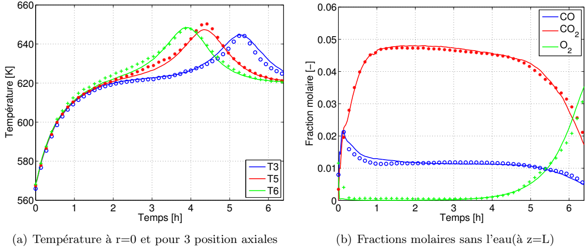
FIGURE 5.6 – Comparaisons entre les prédictions du modèle et les mesures expérimentales (SF_161012) (pour les profils de température et des fractions molaires de CO et CO 2 en sortie) (Modèle cinétique 1 - cas 2)
