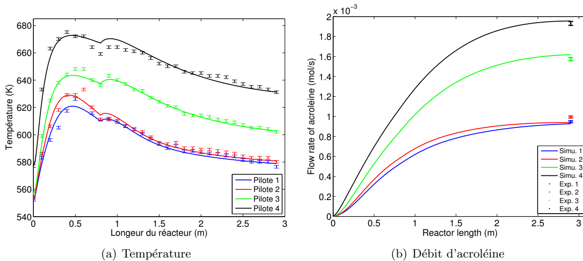
FIGURE 3.17 – Comparaison des profils de température mesurés avec les prédictions du modèle pour le réacteur à l'échelle du pilote – Modèle 2b
