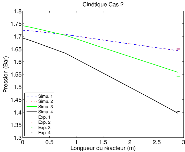
FIGURE 3.14 – Comparaison des mesures de pression aux profils prédits dans le réacteur à l'échelle du pilote – Modèle 1
