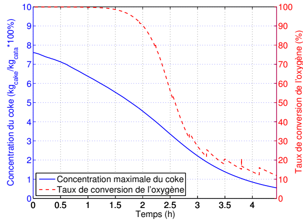
FIGURE 5.20 – Profils de la concentration maximale du coke et le taux de conversion de l’oxygène à la sortie en fonction du temps après optimisation
