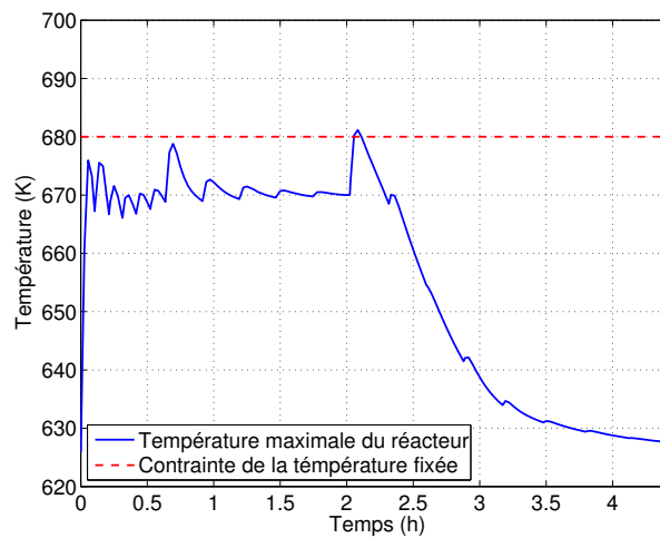
FIGURE 5.25 – Température maximale du réacteur
