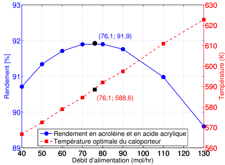
FIGURE 4.6 – Rendement total en acroléine et en acide acrylique et température du fluide caloporteur optimale vs débit d'alimentation - Cas A1
