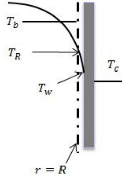
FIGURE 1.1 – Représentation schématique des profils de température dans le lit
