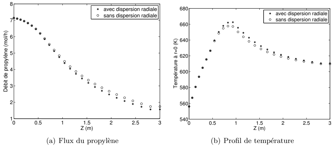
FIGURE 3.7 – Influence de la dispersion radiale sur le flux du propylène et sur le profil de température
