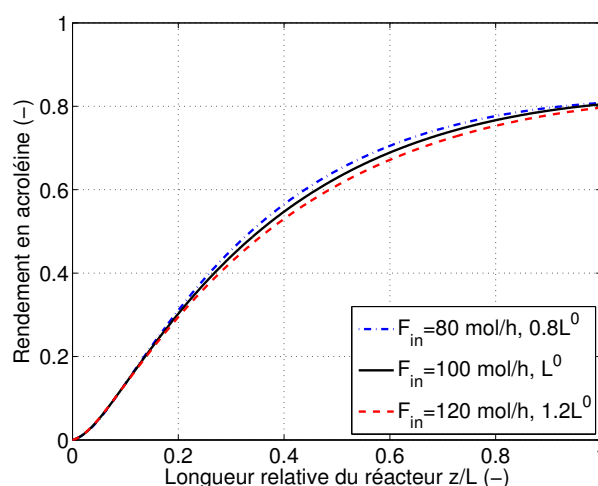
FIGURE 4.4 – Influence de la longueur du lit sur le rendement en acroléine pour la même valeur de VVH ( 1535 \text{ h}^{-1} ) dans les conditions nominales de fonctionnement. ( P_{in}^0, T_c^0 )
