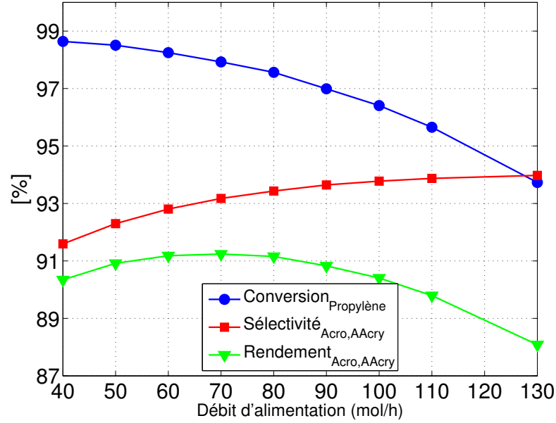
FIGURE 4.11 – Conversion du propylène, sélectivité totale d'acroléine et d'acide acrylique et rendement total en acroléine et en acide acrylique vs débit d'alimentation - Cas B1
