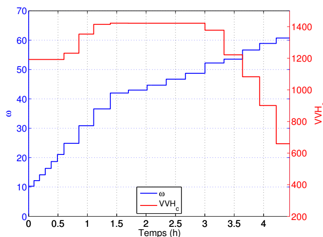
FIGURE 5.27 – Profils optimaux de \omega et du débit de recyclage de gaz ( VVH_c ) (Cas A)
