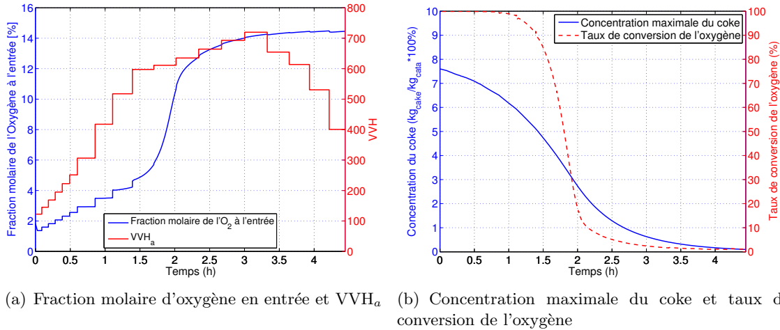
FIGURE 5.28 – Profils des paramètres importants après optimisation (Cas A)
