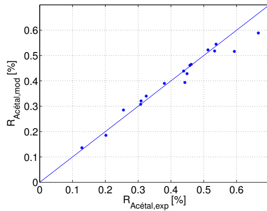
(b) Acétaldéhyde
