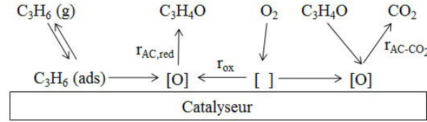
FIGURE 3.5 – Mécanisme réactionnel
