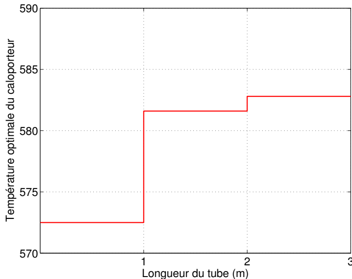
FIGURE 4.15 – Profil optimal de température du fluide caloporteur pour un débit d'alimentation de 70 mol/h
