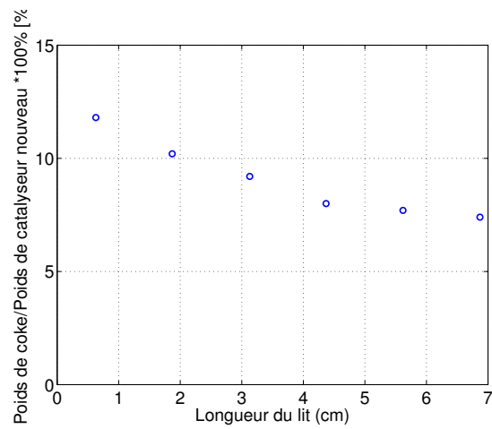
FIGURE 5.5 – Concentration du coke mesurée dans un réacteur à l'échelle du laboratoire (après une production de 24 h)
