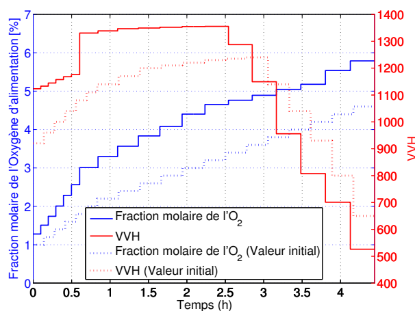
FIGURE 5.19 – Profils initiaux et optimaux des variables de décision
