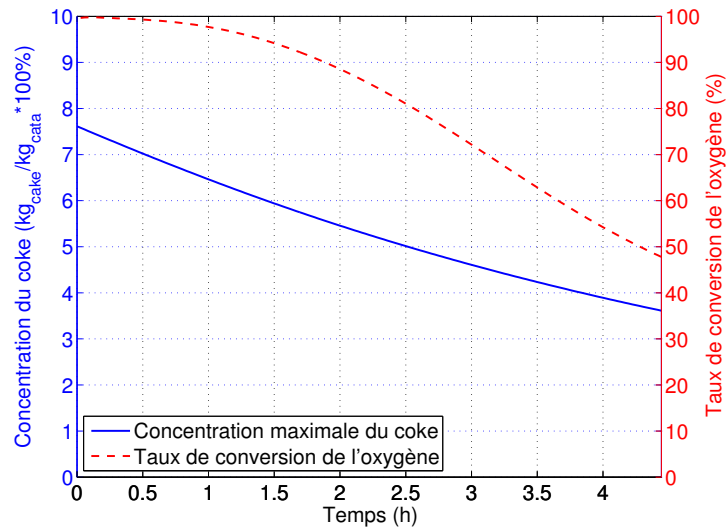
FIGURE 5.12 – Profil temporel de la concentration maximale du coke dans le réacteur et profil temporel du taux de conversion de l'oxygène à la sortie du réacteur après optimisation
