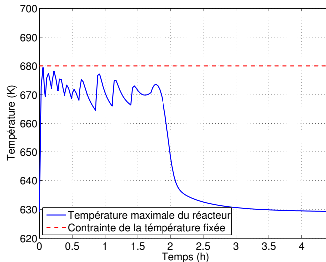
FIGURE 5.29 – Température maximale du réacteur (Cas A)
