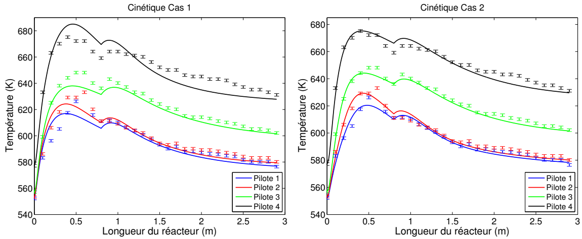
FIGURE 3.11 – Comparaison des profils de température mesurés avec les prédictions du modèle pour le réacteur à l'échelle du pilote – Modèle 1
