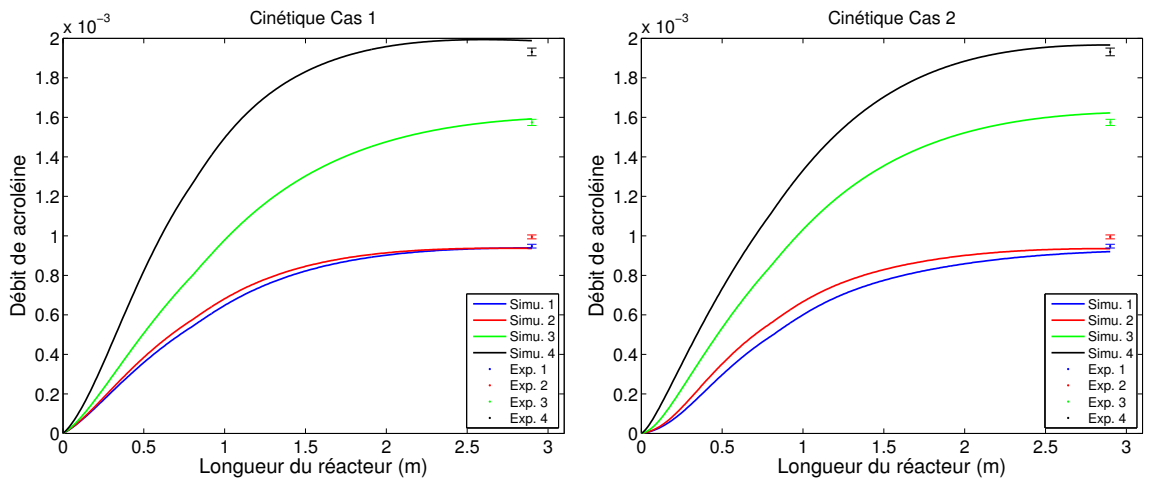
FIGURE 3.12 – Comparaison des débits d'acroléine mesurés à la sortie aux prédictions du modèle pour le réacteur à l'échelle du pilote – Modèle 1
