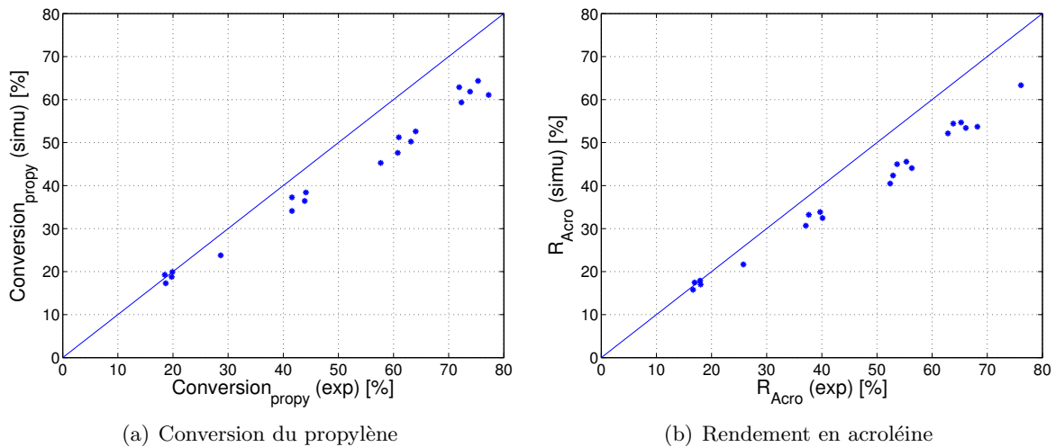
FIGURE 3.15 – Prédiction du modèle en fonction des mesures expérimentales avec la cinétique Cas 2 (expériences à l'échelle du laboratoire – Modèle 1)
