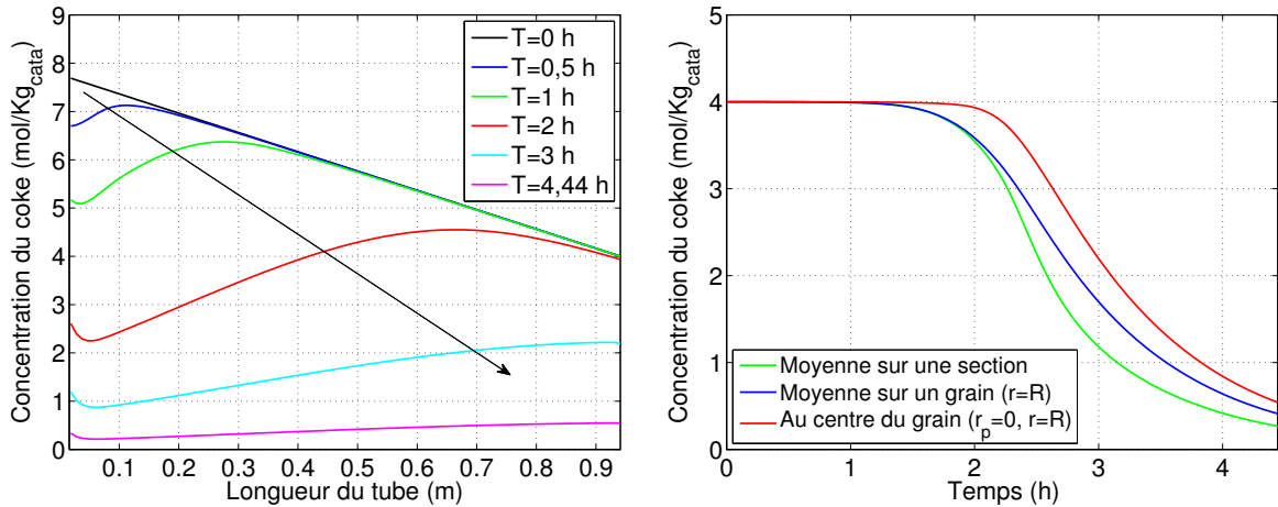
(a) C_{\text{coke}} (à côté de la paroi du réacteur r=R et au centre du catalyseur r_p=0 ) en fonction de la longueur du tube pour différents temps
