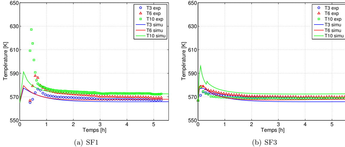
FIGURE 6.6 – Comparaison des prédictions et des expériences de température de trois différents points au centre du réacteur
