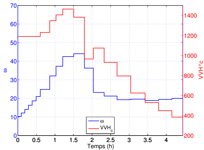
FIGURE 5.30 – Profils optimaux de \omega et du débit de recyclage de gaz ( VVH_c ) (Cas B)
