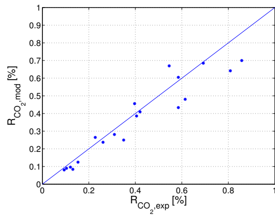
(d) CO 2
