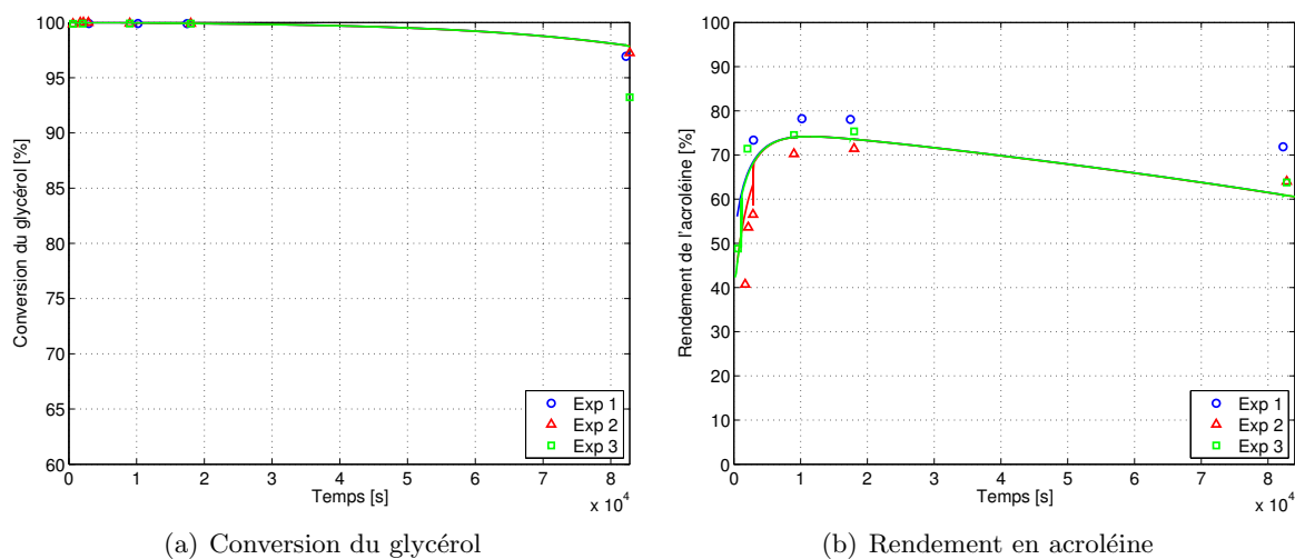
FIGURE 6.4 – Comparaison des prédictions et des expériences du taux de conversion du glycérol et du rendement en acroléine en sortie du réacteur (procédé avec catalyseur GHK24)
