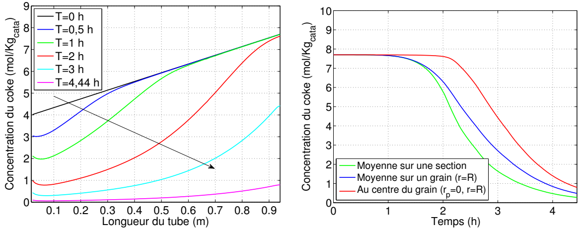
(a) C_{\text{coke}} ( r=R, r_p=0 ) en fonction de la longueur du tube pour différents temps
