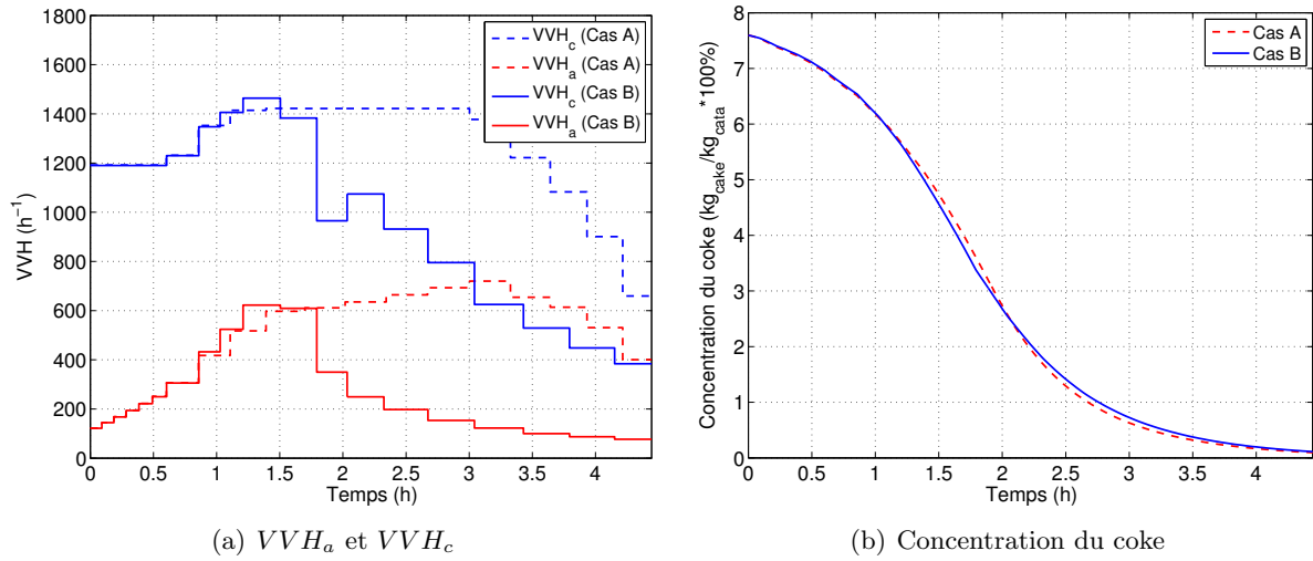
FIGURE 5.32 – Comparaison entre les deux fonctions objectifs (avec et sans débit)
