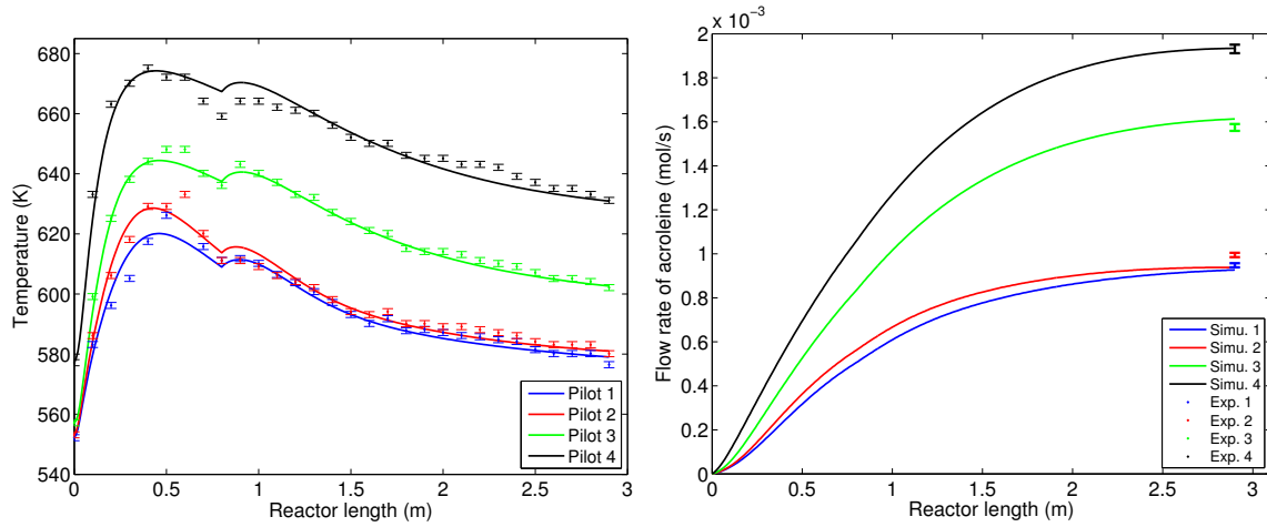
FIGURE 3.21 – Comparaison des profils de température au centre du réacteur mesurés et des débits d'acroléine mesurés à la sortie avec les prédictions du modèle pour le réacteur à l'échelle du pilote – Modèle 3
