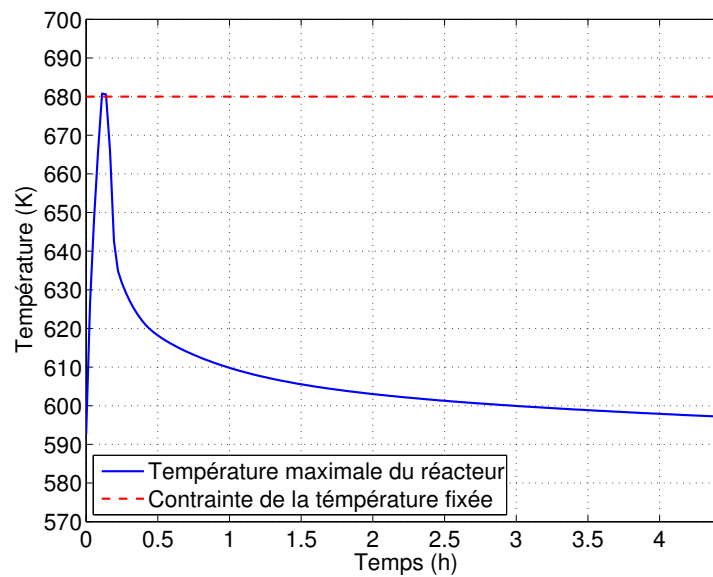
FIGURE 5.13 – Température maximale du réacteur
