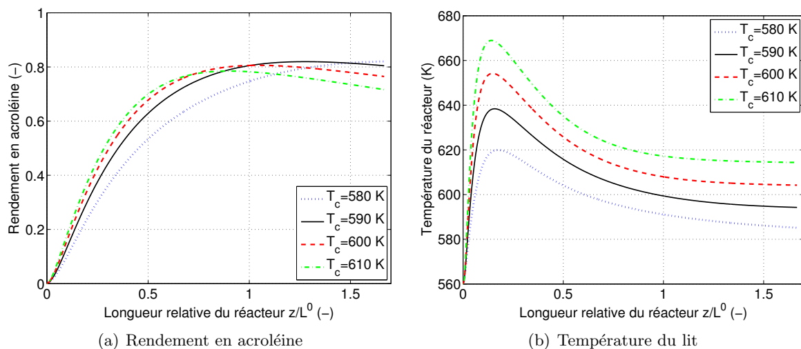
FIGURE 4.2 – Influence de la température du fluide caloporteur sur le rendement en acroléine (a) et sur le profil de température du lit (b) dans les conditions nominales de fonctionnement. ( P_{in}^0, F_t^0, L^0 )
