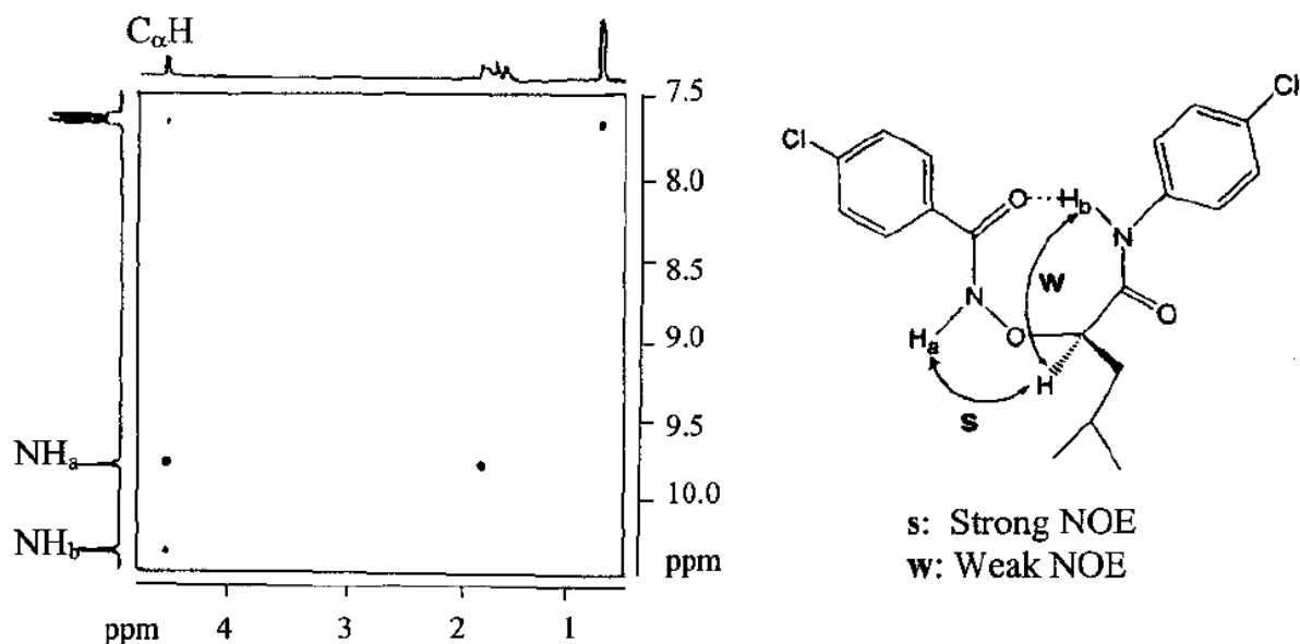
Figure 44 Spectre NOESY du dérivé aminoxy de Yang 218
