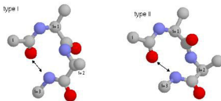
Figure 36 Coudes \beta de type I et II
