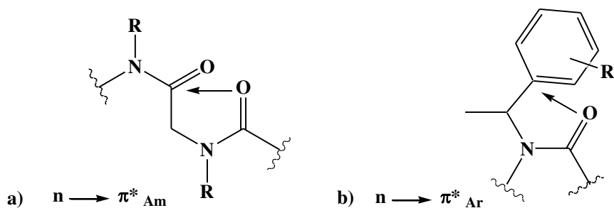
Figure 13 Délocalisations électroniques locales dans les peptoïdes : a) entre carbonyles adjacents b) entre un carbonyle et une chaîne aromatique.
