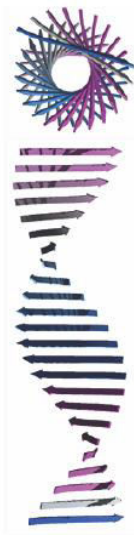
Figure 39 Structures, vue de dessus et vue de côté, des fibres amyloïdes. Seul le coeur de la fibre est représenté. Les feuillets provenant des différentes protéines sont représentés par des flèches. Adapté de Blake 215
