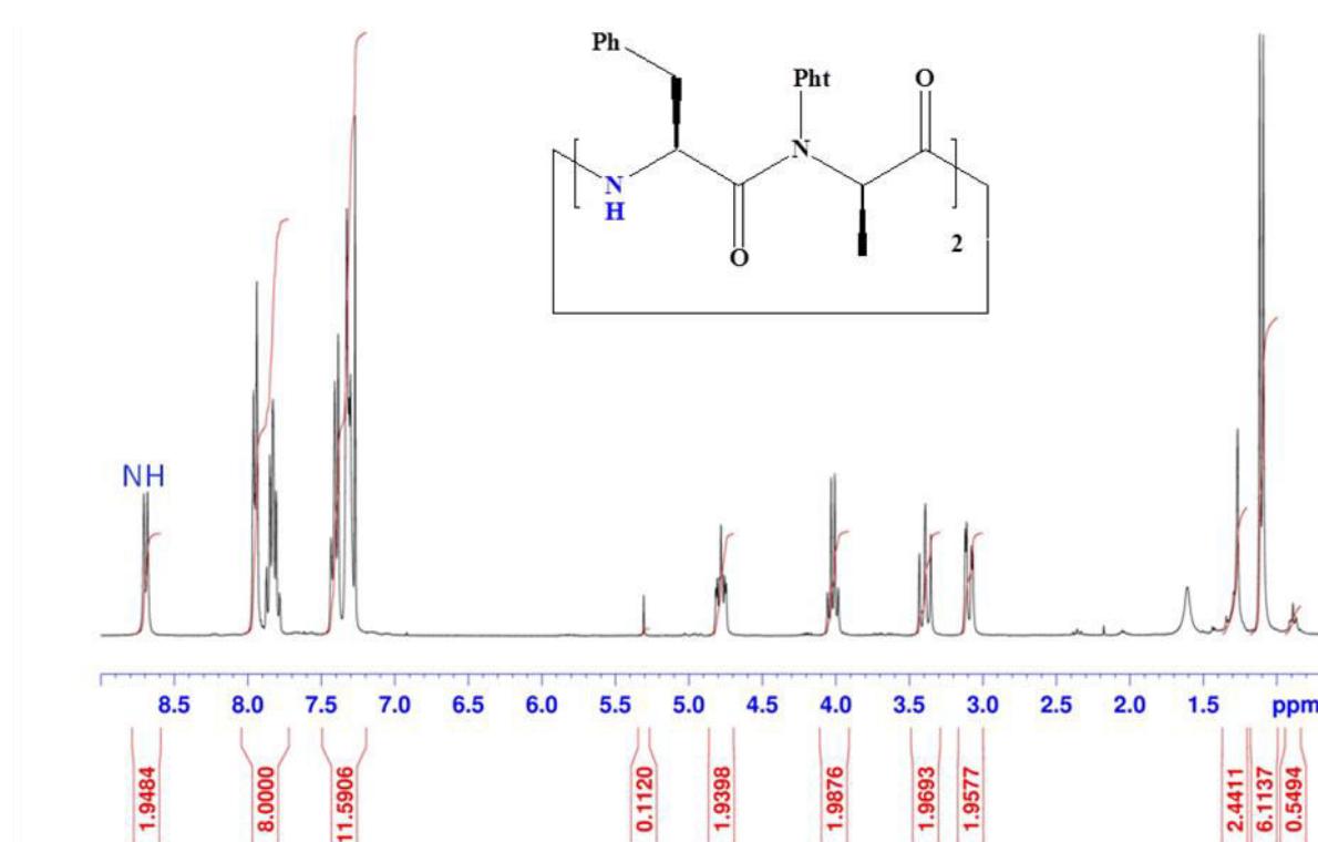
Figure 87 Spectre RMN 1 H (CDCl 3 ) du tétramère cyclique -(S)PheΨ[CON(Pht)](R)Ala 2 - 17a (CDCl 3 /10 mM)
