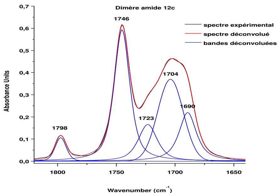
Figure 66 Spectre IR de la zone des vibrateurs CO du dimère amide BocGly Ψ[CON(Ph)]GlyNH 2 12c (CHCl 3 /10 mM)
