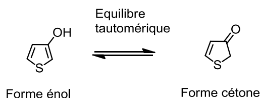
Schéma 13 Tautomérie des 3-hydroxythiophènes 128,129
