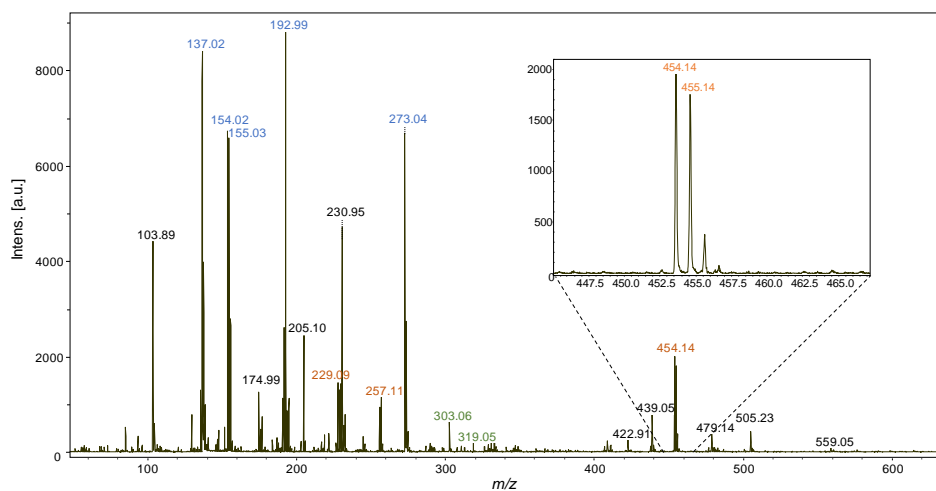
Figure IV-16 : spectre MALDI-TOFMS après un dépôt de 5 µL de DHB sur un échantillon irradié Rpv1 22-8-78.
