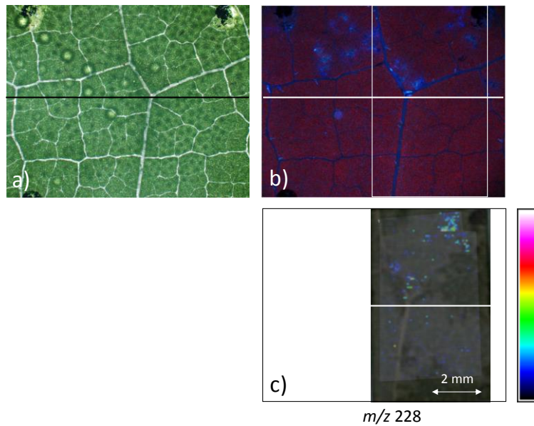
Figure V-25 : analyses de l'échantillon #3 1202. Clichés de microscopie (a) en transmission et (b) en fluorescence, (c) image de la répartition de l'ion m/z 228. Les barres verticales de l'image (b) délimitent la zone analysée en MSI. Les traits horizontaux délimitent la zone infectée (supérieure) de la zone témoin (inférieure).
