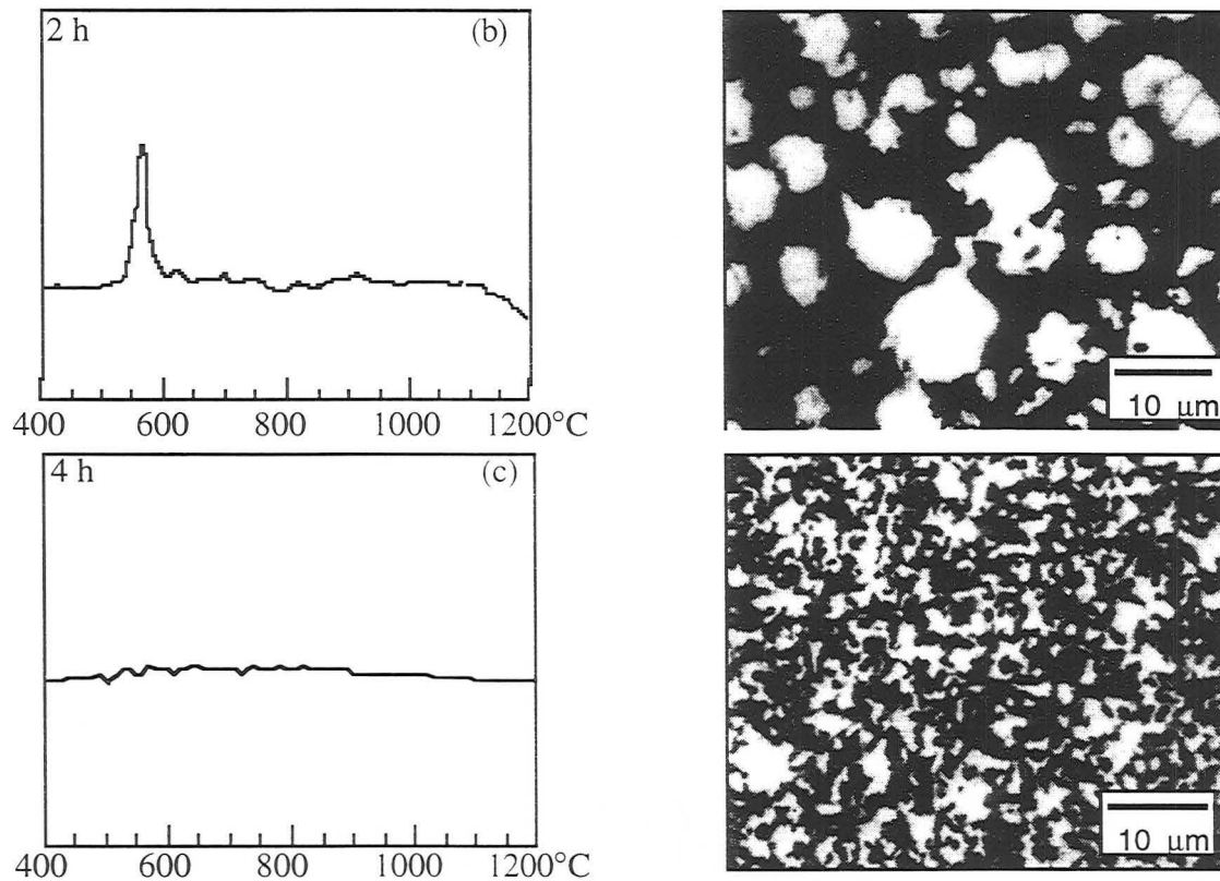
Fig. 20 : Courbes ATD pour des poudres (Al+Cr 2 O 3 ) broyées différents temps et microstructures des matériaux frittés correspondants.
