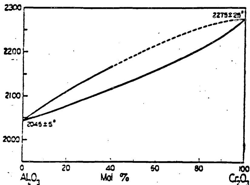
Fig. 1 : Diagramme de phases \text{Al}_2\text{O}_3 - \text{Cr}_2\text{O}_3 (2).
