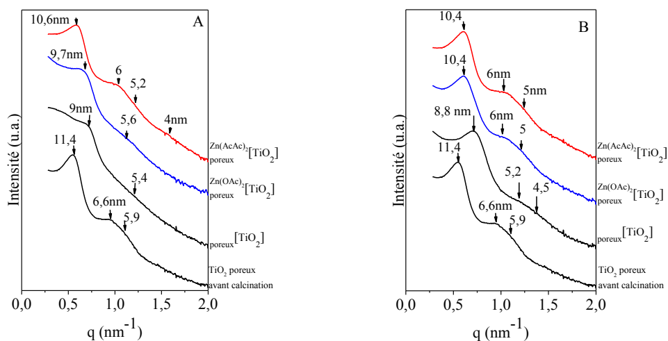
Figure IV-29 – Evolution des diffractogrammes SAXS des \text{TiO}_2 poreux, \text{Zn}(\text{OAc})_2[\text{Ti} - \text{Zn}] et \text{Zn}(\text{AcAc})_2[\text{Ti} - \text{Zn}] en comparaison avec celui de \text{TiO}_2 mésoporeux extrait, non calciné. Calcination au four (A), par IF (B).
