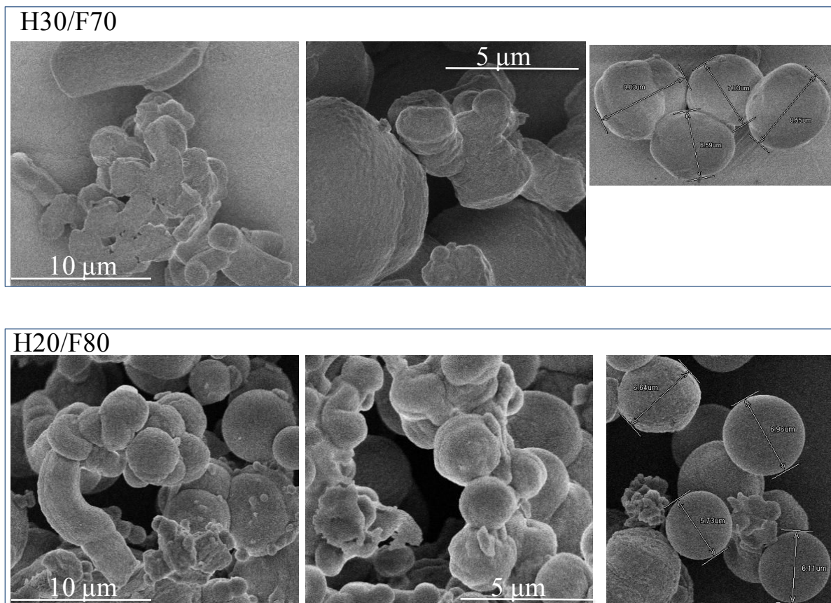
Figure V-8 – Morphologie des particules de silices mésoporeuses des matériaux préparés avec H30/F70 et H20/F80, selon le mécanisme CTM pour R^{\text{F}} = 0,5 .
