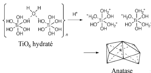
Figure I-18 – Schéma illustrant la nucléation d'anatase en solution contenant d' HCl 151 .
