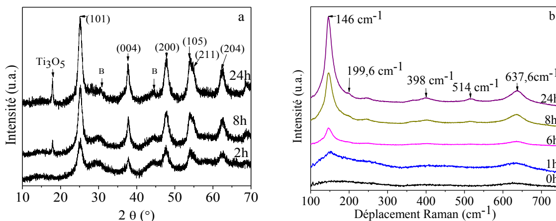
Figure III-45 – Evolution des diffractogrammes rayons X (a) et des spectres Raman (b) des matériaux TiO 2 non calcinés en fonction du temps d'immersion dans l'eau à 120°C.
