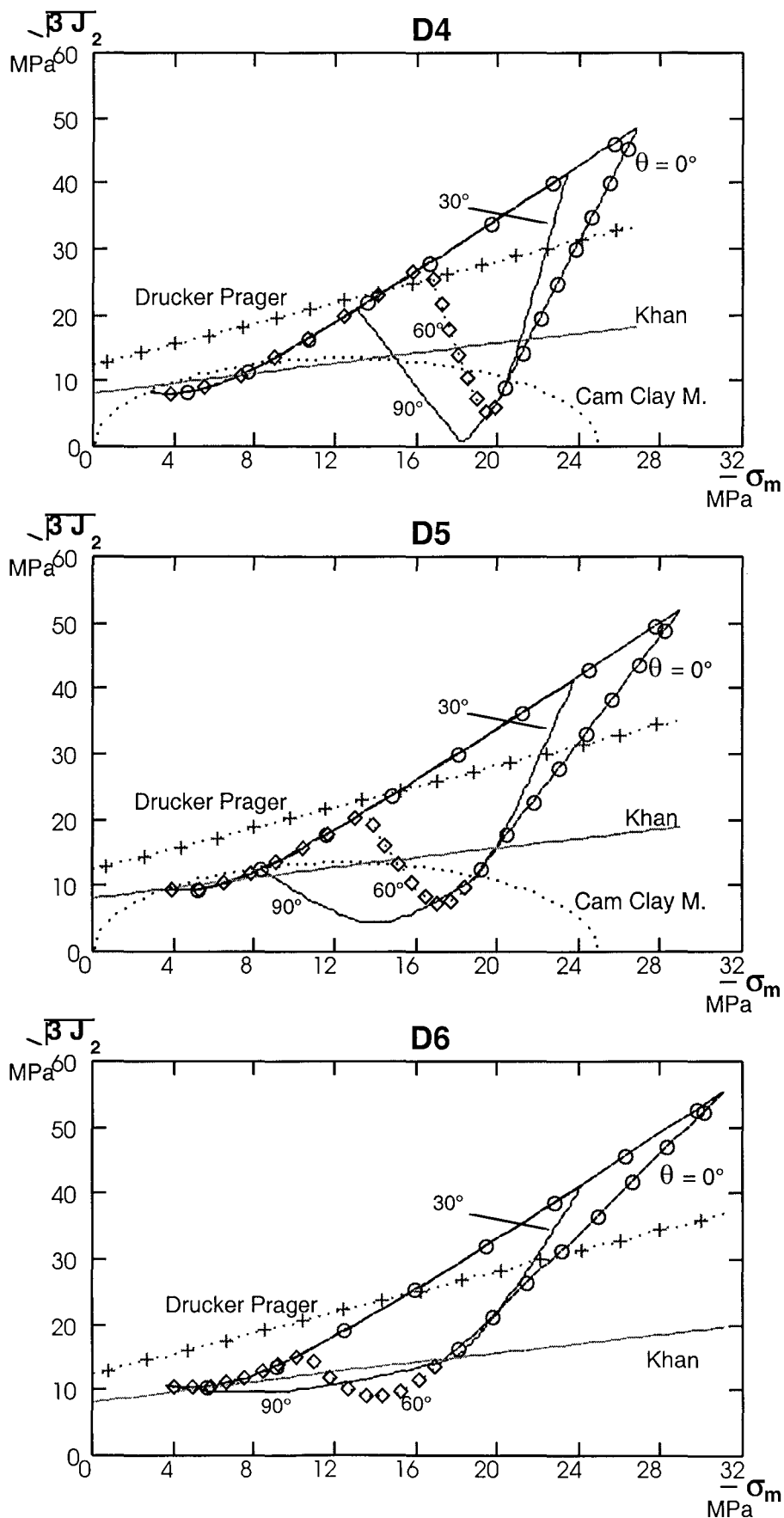
Figure A1.14 - Chemins de contrainte dans le plan |\bar{\sigma}_m| - \sqrt{3}J_2 ( \sigma_{zz,init} = -20 MPa; \sigma_H = -24 MPa) (D4 : \sigma_h = -16 MPa; D5 : \sigma_h = -12 MPa ; D6 : \sigma_h = -8 MPa)
