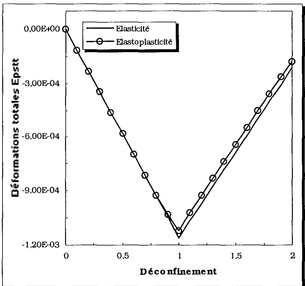
Jauge E_{90}
