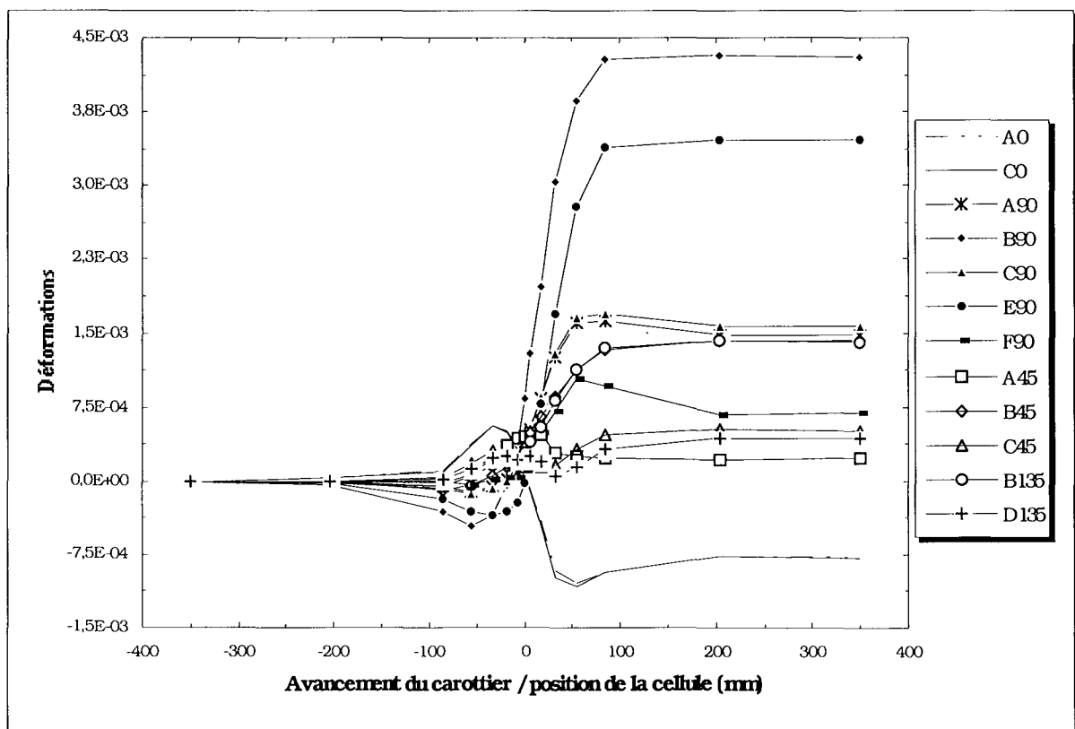
Fig. A2.8 - Évolution de la déformation de la totalité des jauges matériau isotrope transverse, chargement déviatorique T1, orientation ( \beta=90^\circ , \theta=30^\circ ).
