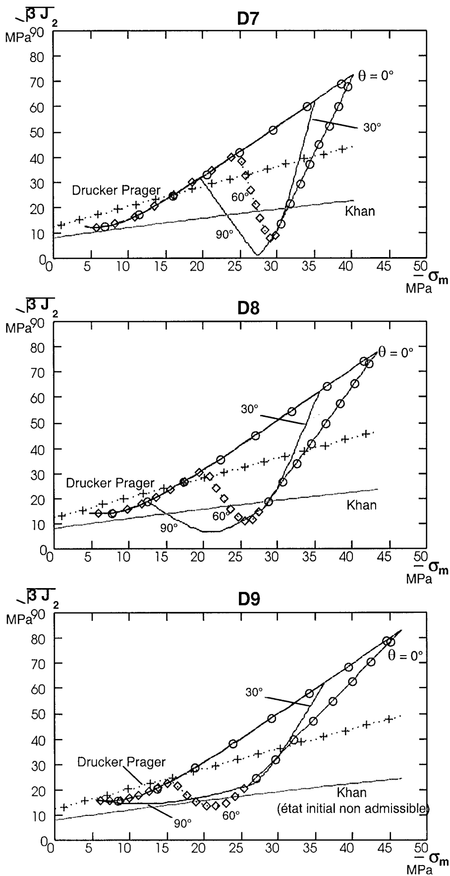
Figure A1.15 - Chemins de contrainte dans le plan |\bar{\sigma}_m| - \sqrt{3} J_2 ( \sigma_{zz,init} = -30 MPa; \sigma_H = -36 MPa) (D7 : \sigma_h = -24 MPa; D8 : \sigma_h = -18 MPa ; D9 : \sigma_h = -12 MPa)
