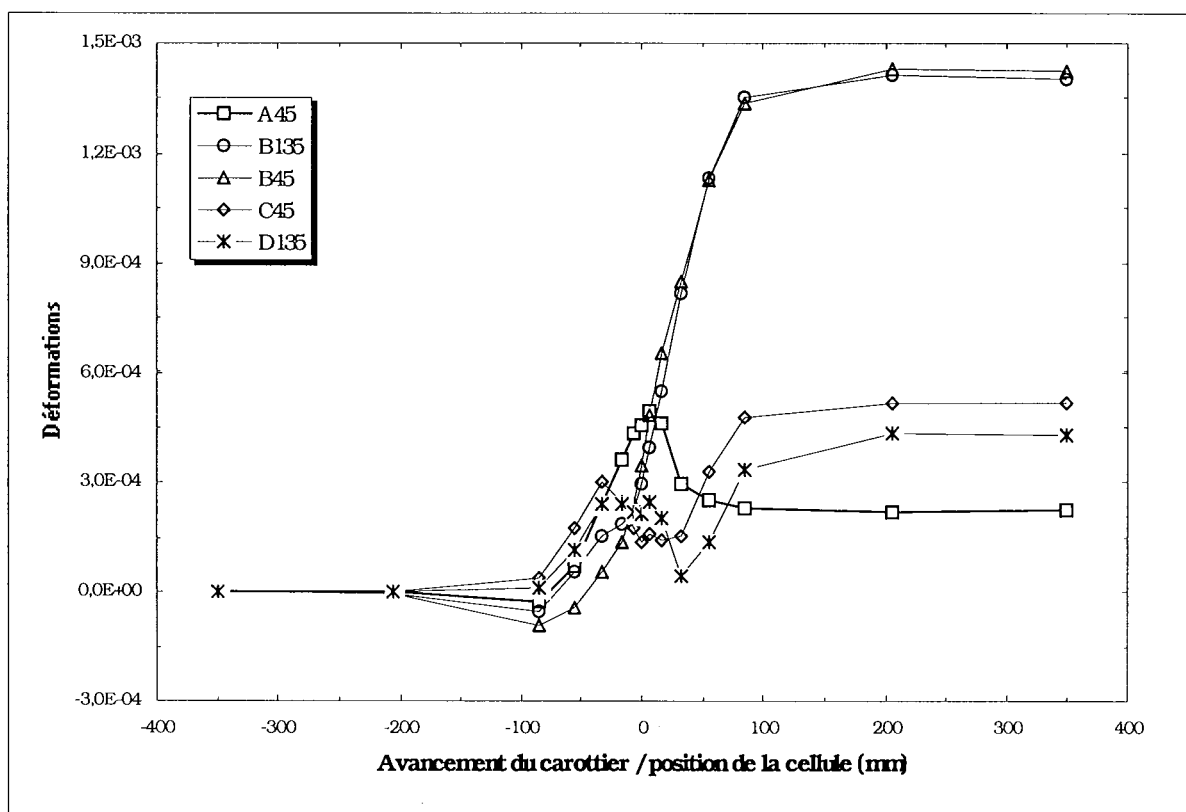
Fig. A2.10 - Évolution de la déformation des jauges inclinées matériau isotrope transverse, chargement déviatorique T1, orientation ( \beta=90^\circ , \theta=30^\circ ).
