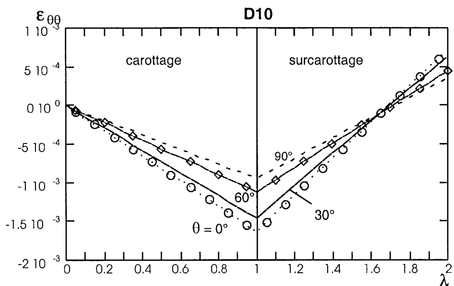
Figure A1.8 - Déformation orthoradiale \varepsilon_{\theta\theta} ( r' = 1 ) en fonction du taux de déconfinement D10 : \sigma_H = -24 MPa , \sigma_h = -18 MPa K = 1,33
