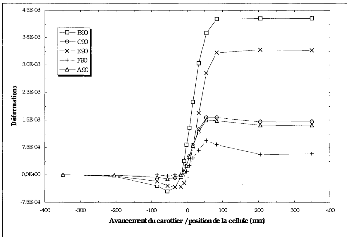
Fig. A2.3 - Évolution de la déformation des jauges circulaires matériau isotrope transverse, chargement déviatorique T1, orientation ( \beta=90^\circ , \theta=45^\circ ).
