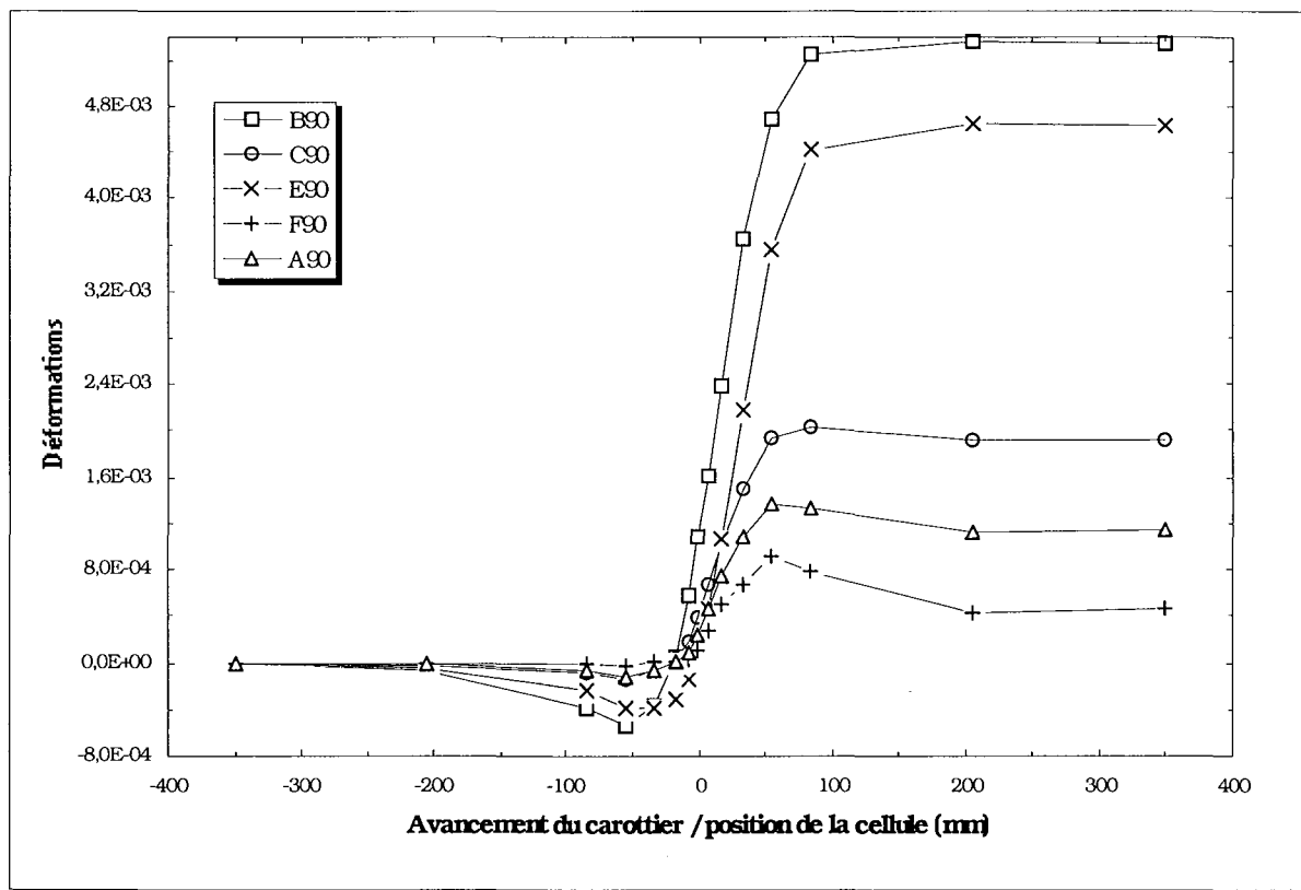
Fig. A2.15 - Évolution de la déformation des jauges circulaires matériau isotrope transverse, chargement déviatorique T1, orientation ( \beta=30^\circ , \theta=60^\circ ).
