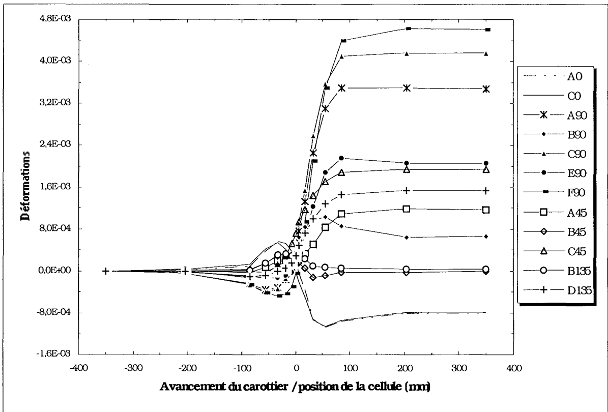
Fig. 84 - Évolution de la déformation de la totalité des jauges matériau isotrope transverse , chargement déviatorique T 2 , orientation (Béta=30°, Téta=60°).
