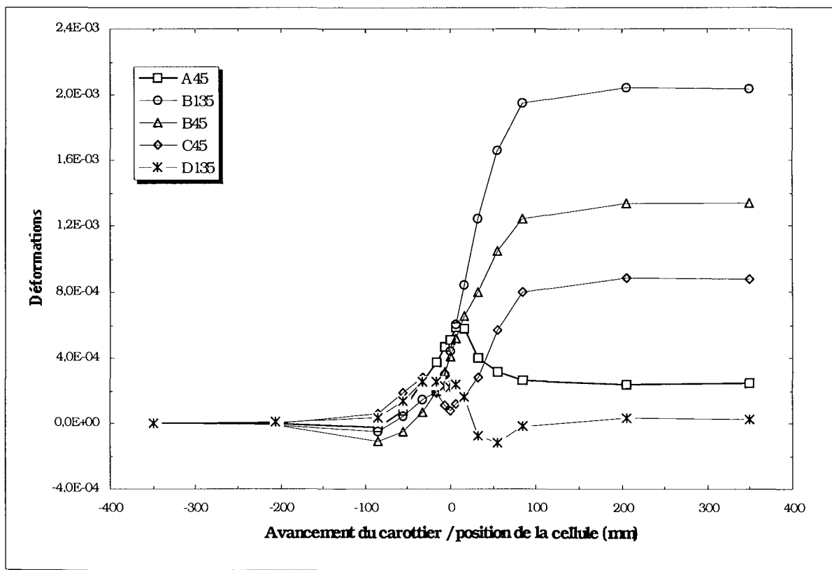
Fig. A2.16 - Évolution de la déformation des jauges inclinées matériau isotrope transverse, chargement déviatorique T1, orientation ( \beta=30^\circ , \theta=60^\circ ).
