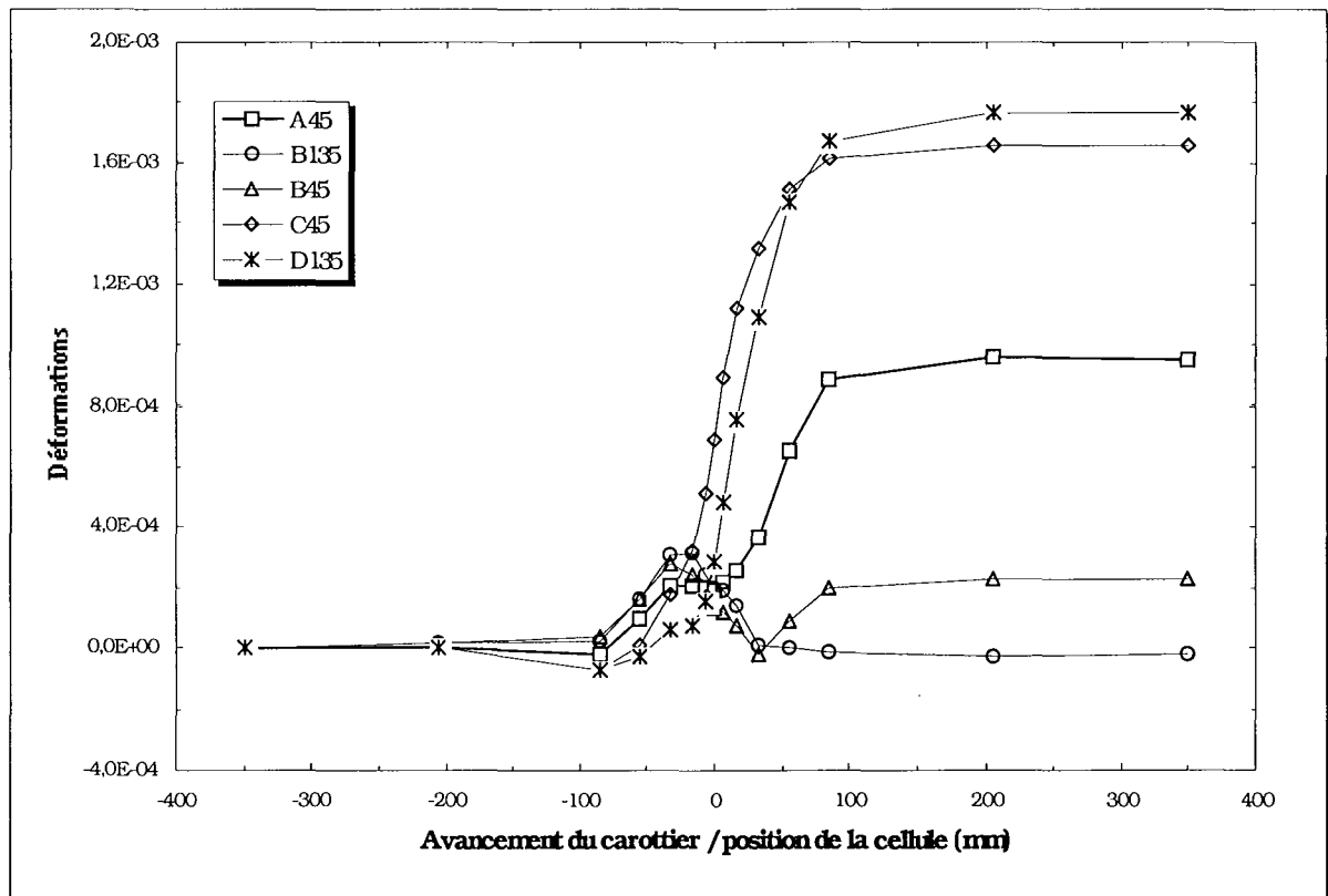
Fig. A2.7 - Évolution de la déformation des jauges inclinées matériau isotrope transverse, chargement déviatorique T3, orientation ( \beta=90^\circ , \theta=45^\circ ).
