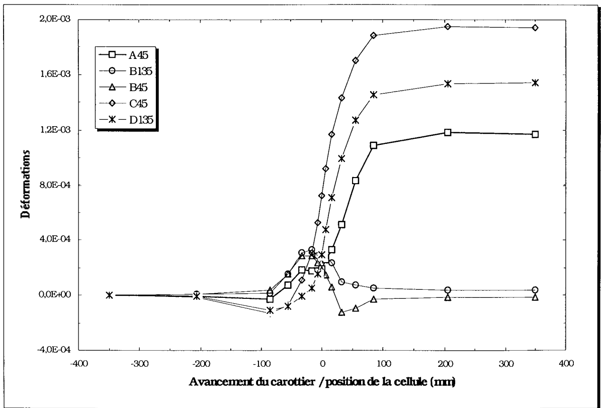
Fig. 85 - Évolution de la déformation des jauges circulaires matériau isotrope transverse, chargement déviatorique T_2 , orientation ( \beta=30^\circ , \theta=60^\circ ).
