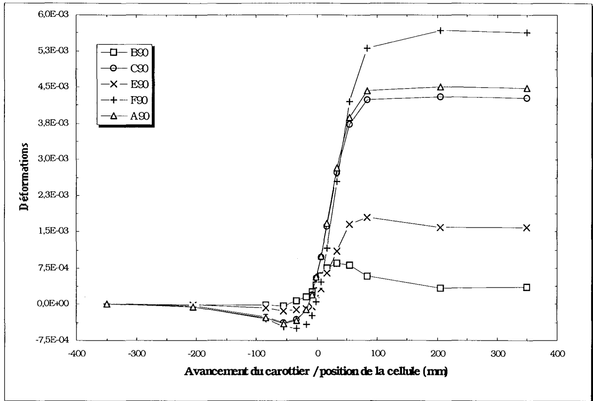
Fig. 80 - Évolution de la déformation des jauges circulaires, matériau isotrope transverse, chargement déviatorique T_2 , orientation ( \beta=90^\circ , \theta=30^\circ ).
