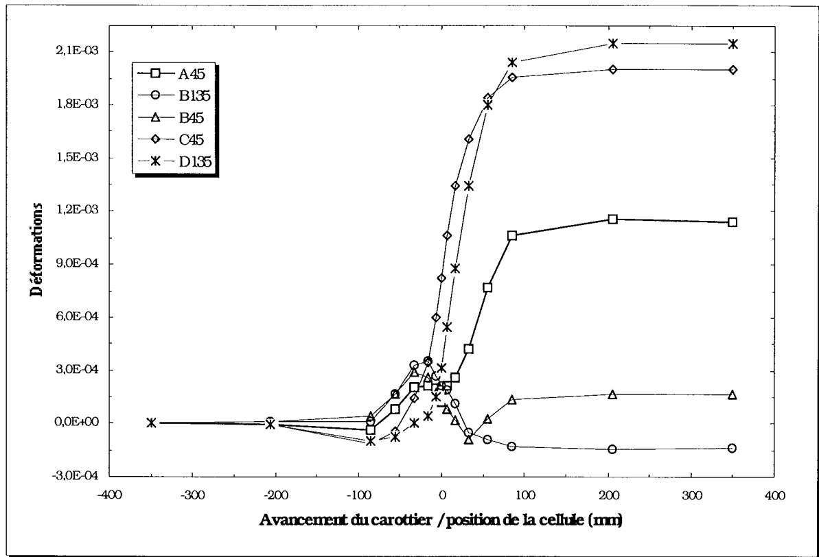
Fig. 75 - Évolution de la déformation des jauges inclinées matériau isotrope transverse, chargement déviatorique T_2 , orientation ( \beta=90^\circ , \theta=45^\circ ).
