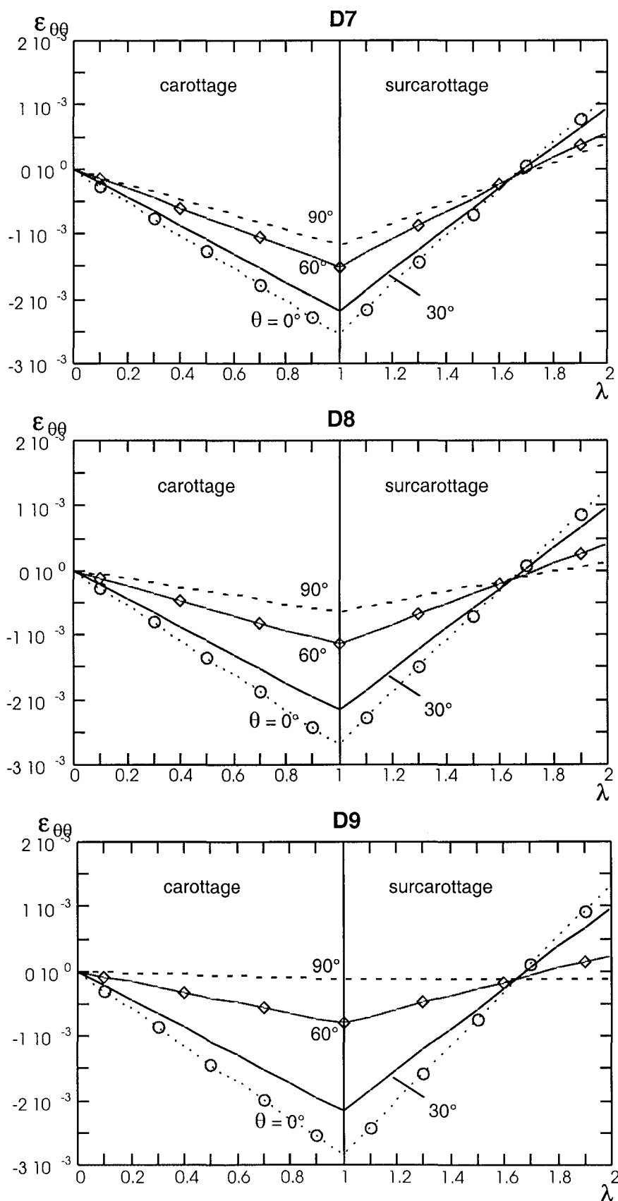
Figure A1.7 - Déformation orthoradiale \epsilon_{\theta\theta} ( r' = 1 ) en fonction du taux de déconfinement \sigma_H = -36 MPa (D7 : \sigma_h = -24 MPa ; D8 : \sigma_h = -18 MPa ; D9 : s_h = -12 MPa)
