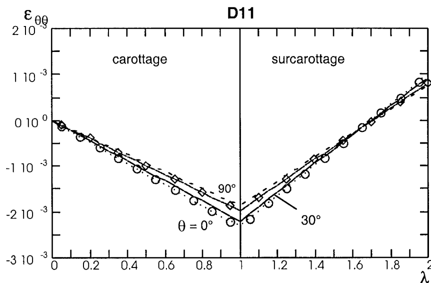
Figure A1.9 - Déformation orthoradiale \varepsilon_{\theta\theta} ( r' = 1 ) en fonction du taux de déconfinement D11 : \sigma_H = -36 MPa , \sigma_h = -32,73 MPa K = 1,1
