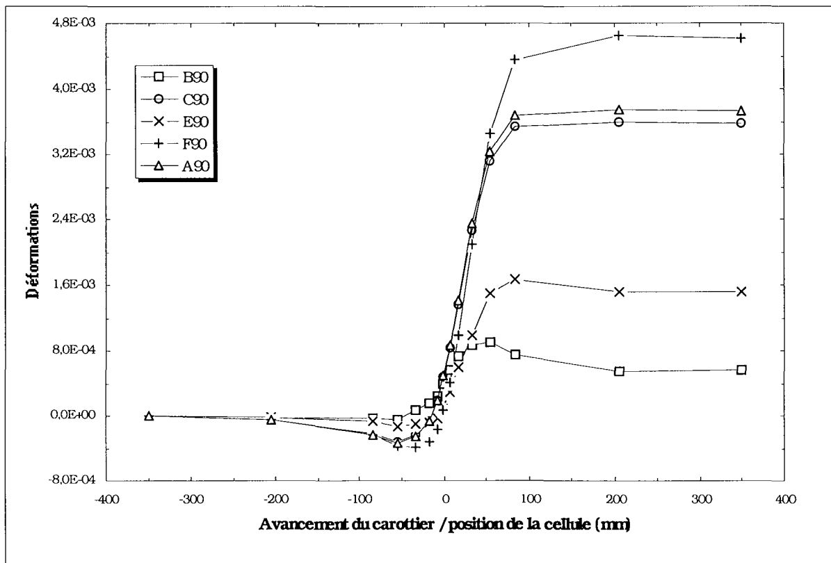
Fig. A2.12 - Évolution de la déformation des jauges circulaires matériau isotrope transverse, chargement déviatorique T3, orientation ( \beta=90^\circ , \theta=30^\circ ).
