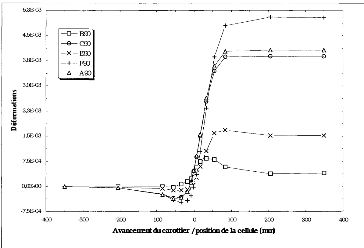
Fig. 74 - Évolution de la déformation des jauges circulaires matériau isotrope transverse , chargement déviatorique T_2 , orientation ( \beta=90^\circ , \theta=45^\circ ).
