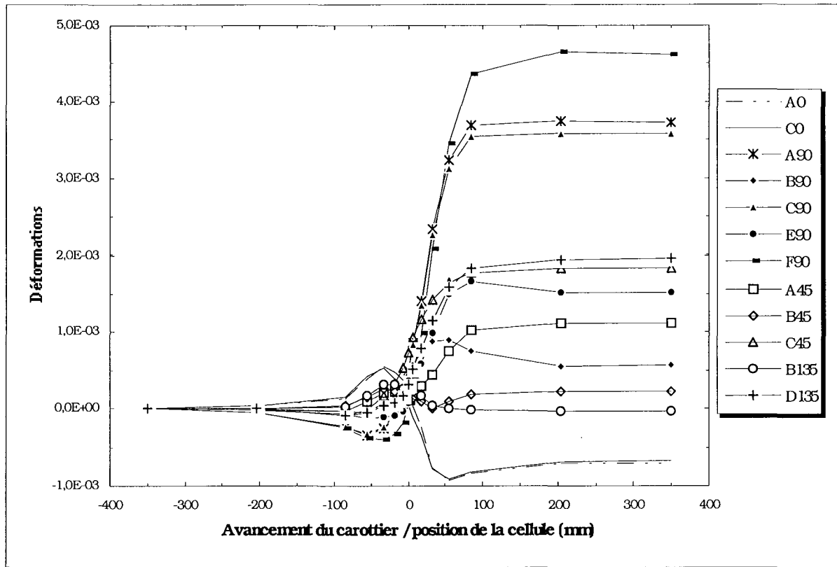
Fig. A2.11 - Évolution de la déformation de la totalité des jauges matériau isotrope transverse, chargement déviatorique T3, orientation ( \beta=90^\circ , \theta=30^\circ ).
