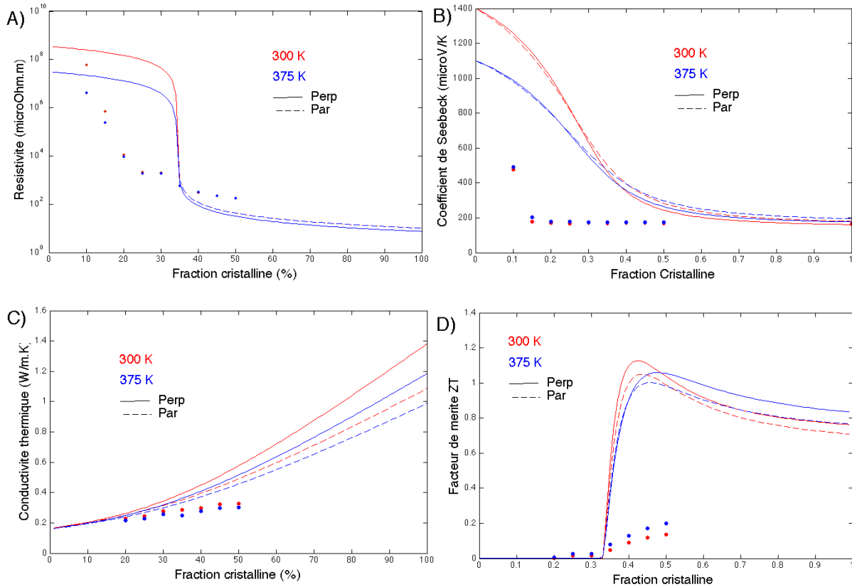
Figure V-33 : Comparaison des propriétés prédites par le modèle et des valeurs expérimentales réellement mesurées. En (A), la résistivité électrique, en (B), le pouvoir thermoélectrique, en (C), la conductivité thermique et en (D), le facteur de mérite ZT. Ces propriétés sont explicitées pour deux températures (300 et 375K) ainsi que pour les deux directions relatives aux propriétés de la phase cristalline native. Les courbes en trait plein représentent la direction perpendiculaire tandis que les courbes en trait pointillé, la direction parallèle.
