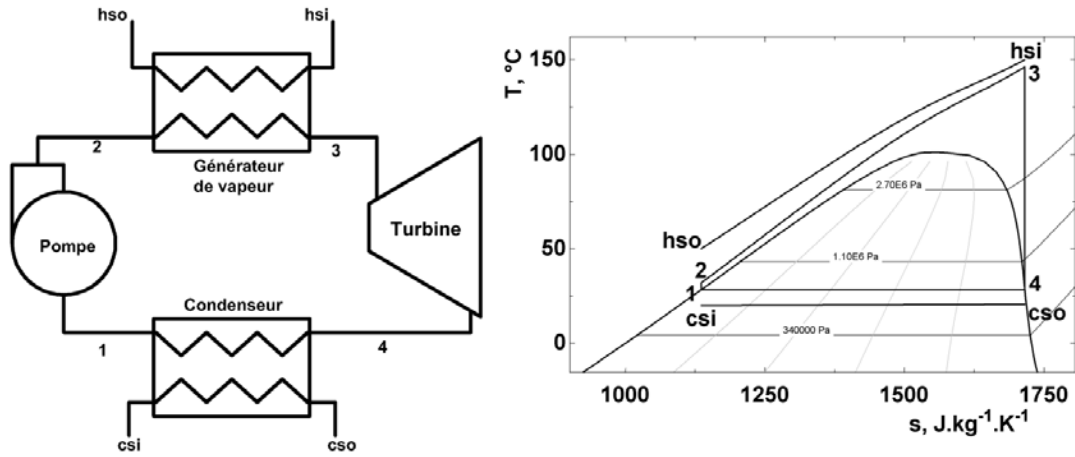
Figure 5. 19. Diagramme schématique et diagramme T-s pour le cycle ORC supercritique
