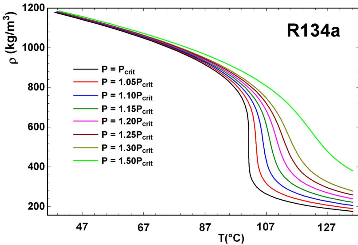
Figure 5. 12. Variation de masse volumique du R134a en fonction de température aux pressions supercritiques (REFPROP v.9.1)
