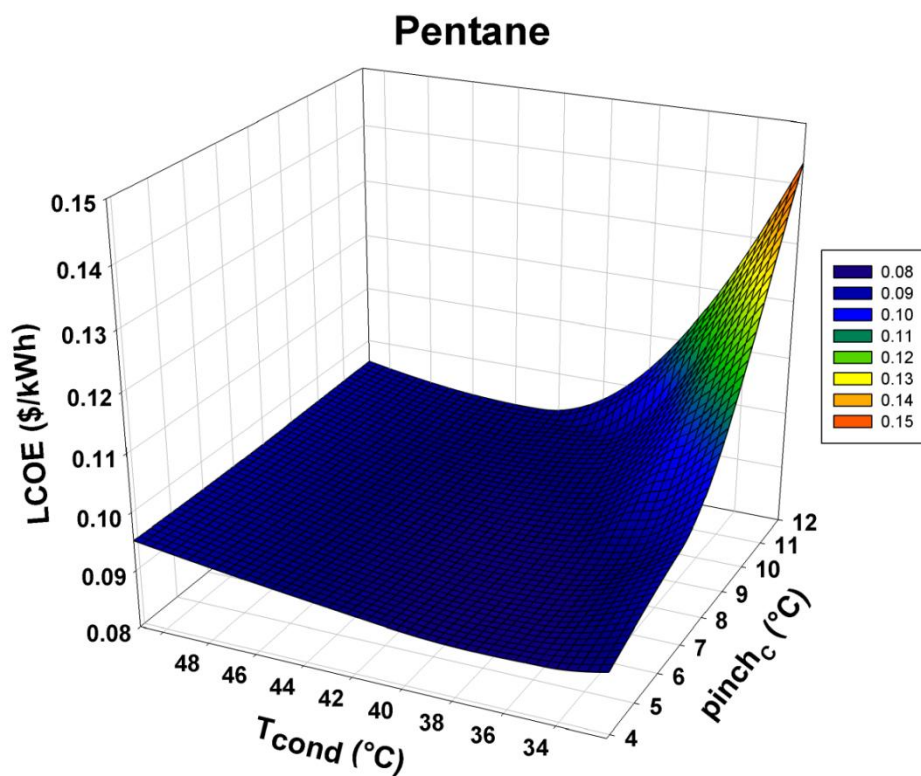
Figure 6. 11. Evolution du LCOE en fonction de température de condensation et de la valeur du pincement de transfert de chaleur à basse pression pour le cycle basé sur n-Pentane
