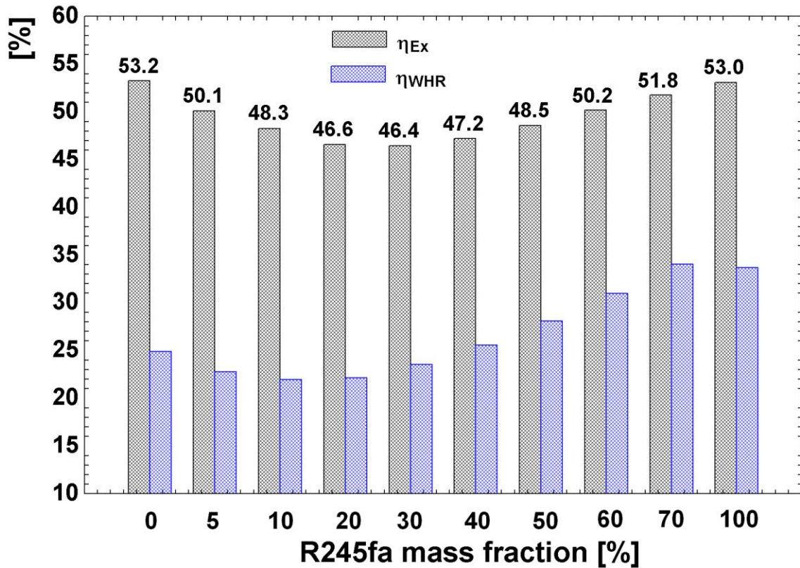
Figure 6. 5. Rendement exergetique maximal et taux de recuperation d'exergie du cycle ORC utilisant differents fluides de travail
