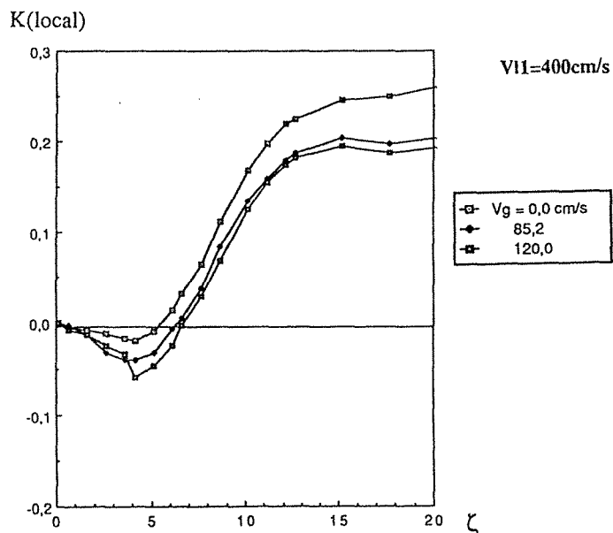
Fig. 4.9 Evolution du coefficient local de la chute de pression en écoulement diphasique dans le voisinage immédiat de l'élargissement \phi_{20}/60\text{mm} pour V_{l1} = 200 cm/s 300 cm/s 400 cm/s
