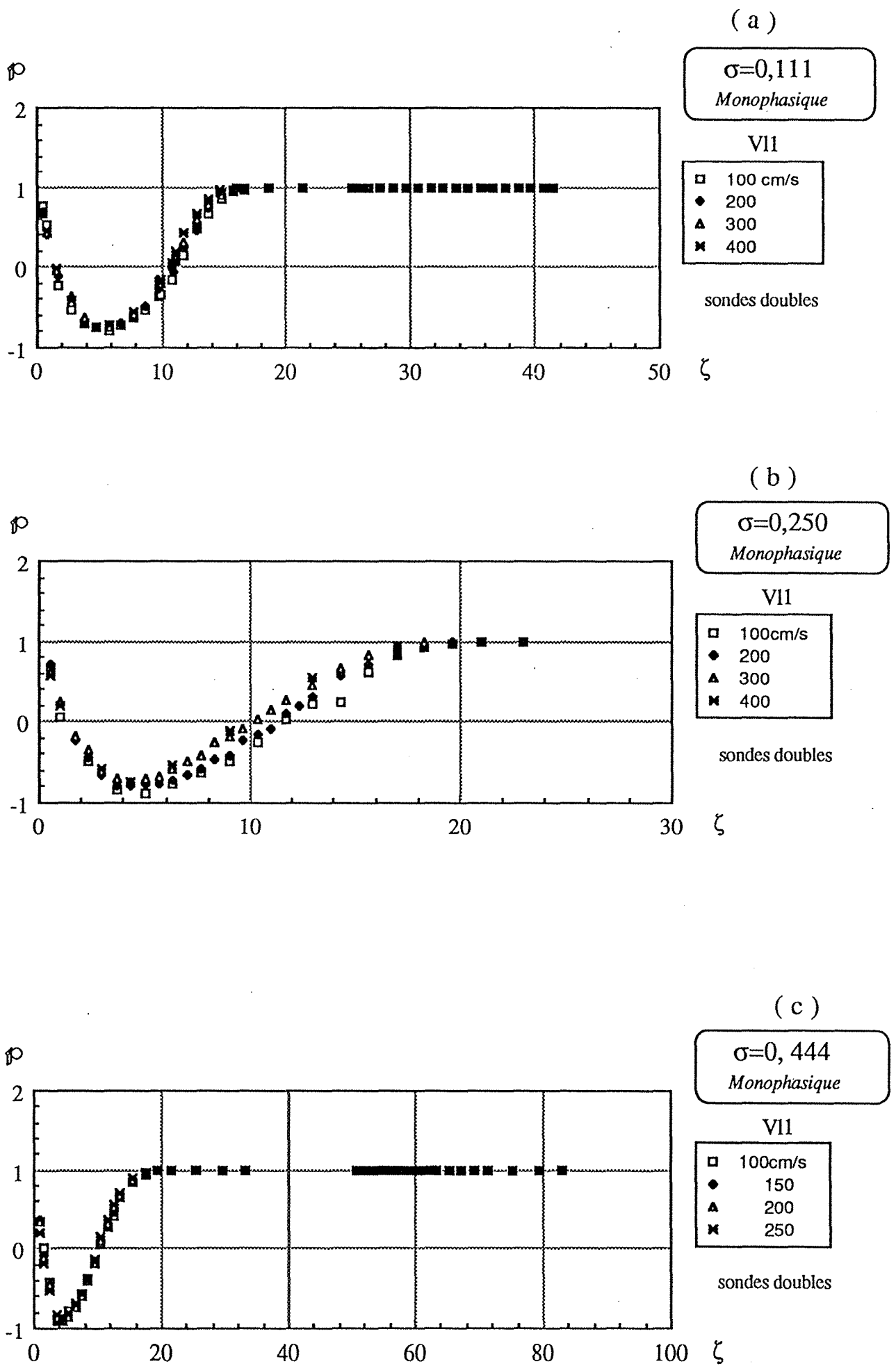
Fig.5.4 Evolution de la fonction intégrale de densité de probabilité lors d'un écoulement monophasique dans les élargissements: (a) \sigma=0,111 (b) \sigma=0,250 (c) \sigma=0,444 .
