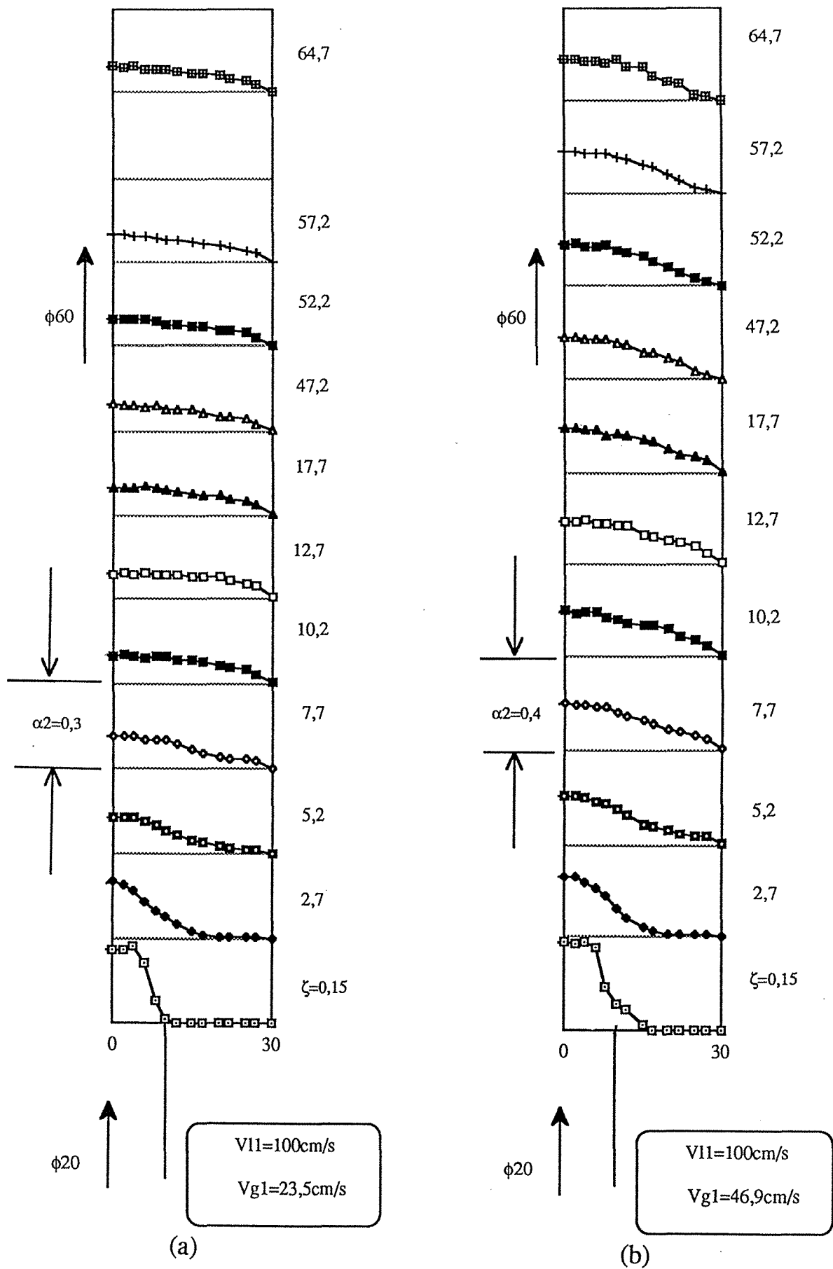
Fig.4.16 Evolution du profil du taux de vide en aval de l'élargissement \phi 20/60 mm avec V_{11}=100 cm/s et (a) V_{g1}=23,5 cm/s (b) V_{g1}=46,9 cm/s.
