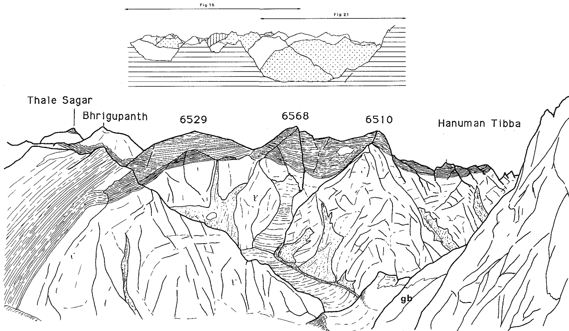
Fig. 21: Panorama réalisé à partir du sommet du Thelu Bamak (petit col en rive droite à 5700 m.). On y voit le glacier du Bhrigupanth et la géométrie générale du contact sommital du leucogranite ( \gamma ) qui dessine une grande structure antiforme. L'arête à l'avant plan est constituée par le granite de Bhairongathi (gb). On comparera avec les coupes présentées en Fig. 33a.
