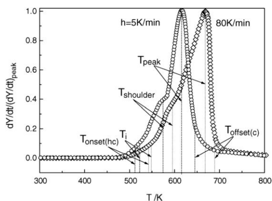
Figure 67 : Températures caractéristiques sur les courbes DTG normalisées de pyrolyse de hêtre à 5 et 80°C.mn -1 .
