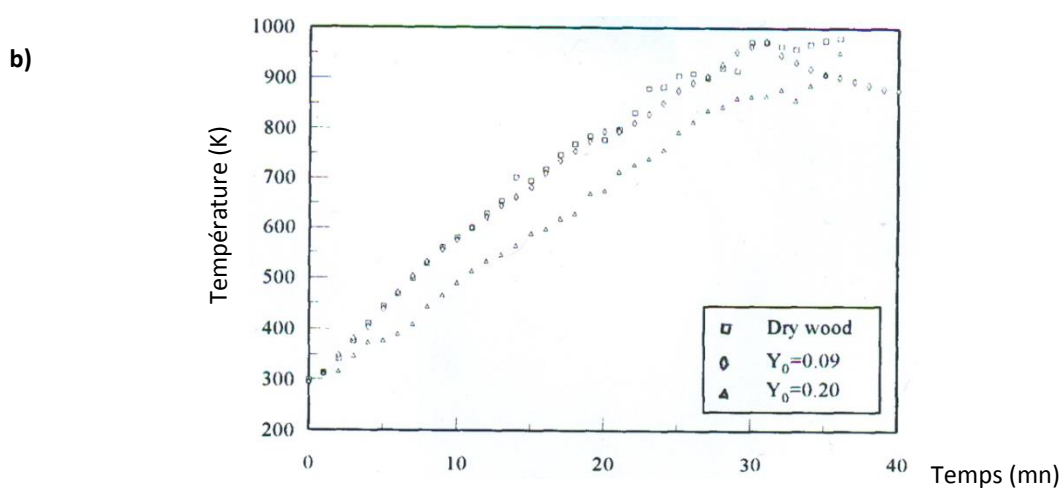
Figure 64 (suite) : Influence de l'humidité sur la température de surface (b) [Bilbao et al., 1996].
