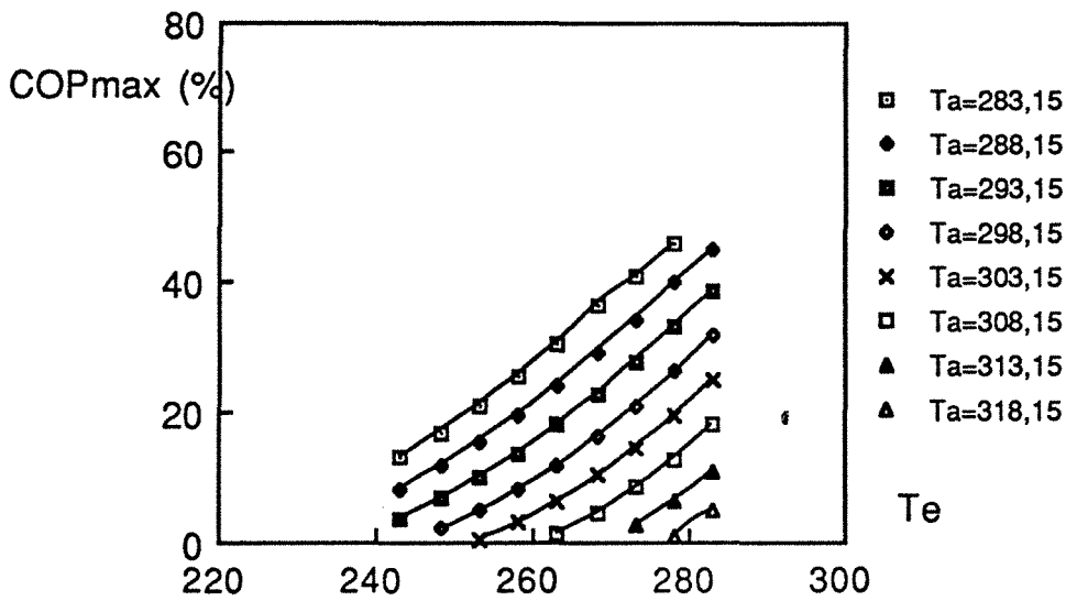
Figure 12. L'évolution des COP max pour le couple Ethanol - Zéolithe 5A
