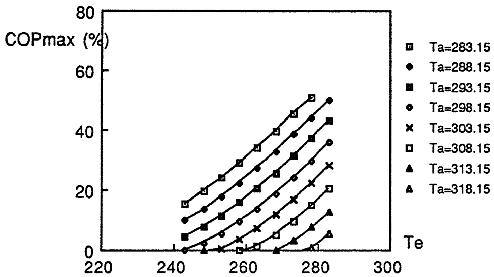
Figure 4. L'évolution des COP max pour le couple Ethanol-AC35/1.8
