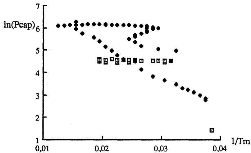
Figure VI-37. Cycle obtenu pour la puissance de 100W
