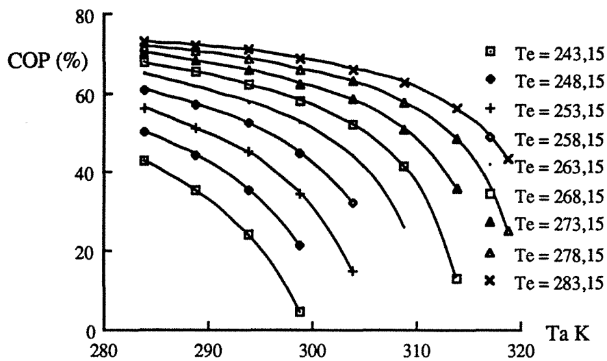
Figure III.12.1 Variation du COP intrinsèque avec T_a à T_g = 100^\circ\text{C} Méthanol-AC40/3
