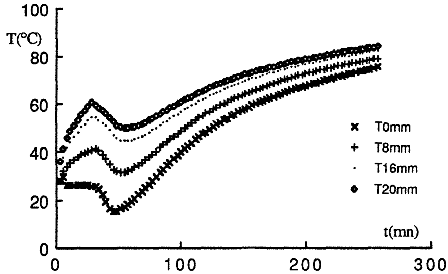
Figure VII-14. Evolution de la température selon le modèle , charge 400ml, P_u=100\text{W} T_0 = 298\text{K} , T_{\infty} = 293\text{K} , C_{wi} = C(303\text{K}, 0,078\text{bar}) , K_i = 20\text{W/m}^2\text{C} , K_0 = 8\text{W/m}^2\text{C} .
