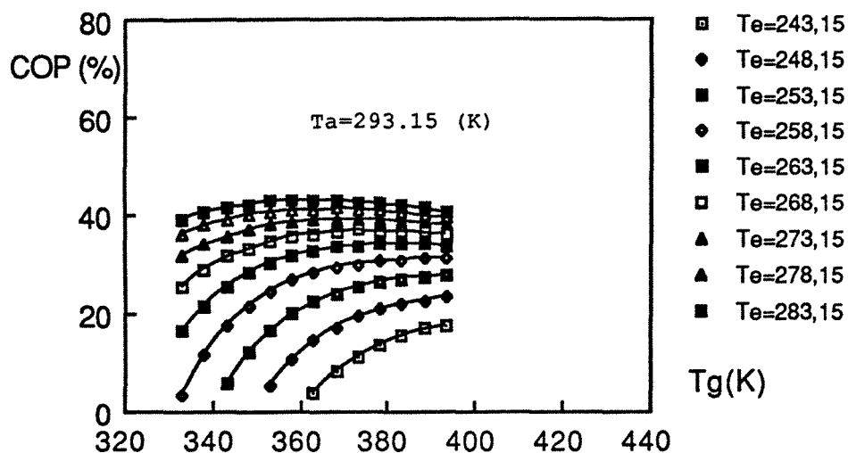
Figure 16. COP i en fonction de T g pour Carbon 208C - Ammoniac
