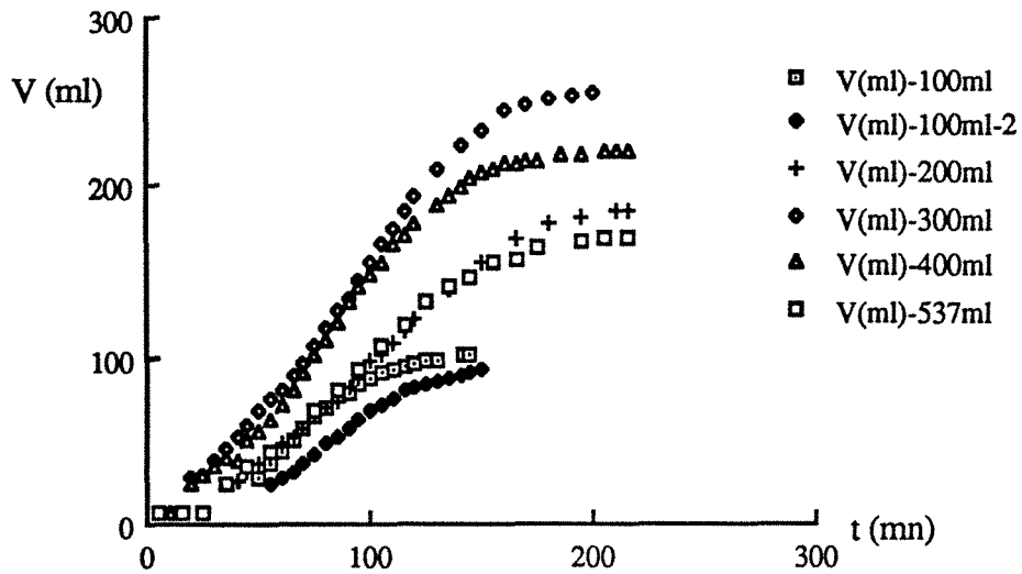
Figure VI-24 Volume cyclé pour différentes charges
