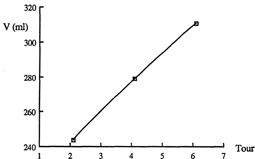
Figure VI-13 Volume cyclé dans le système pour différents tours de vanne
