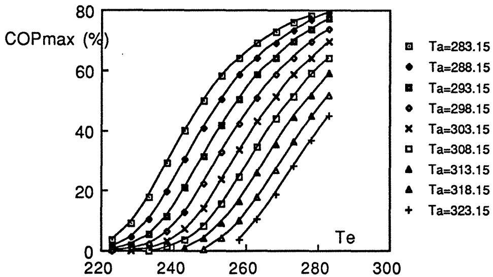
Figure 2. Evolution de COP max pour le couple Méthanol-NORIT RI EXTRA
