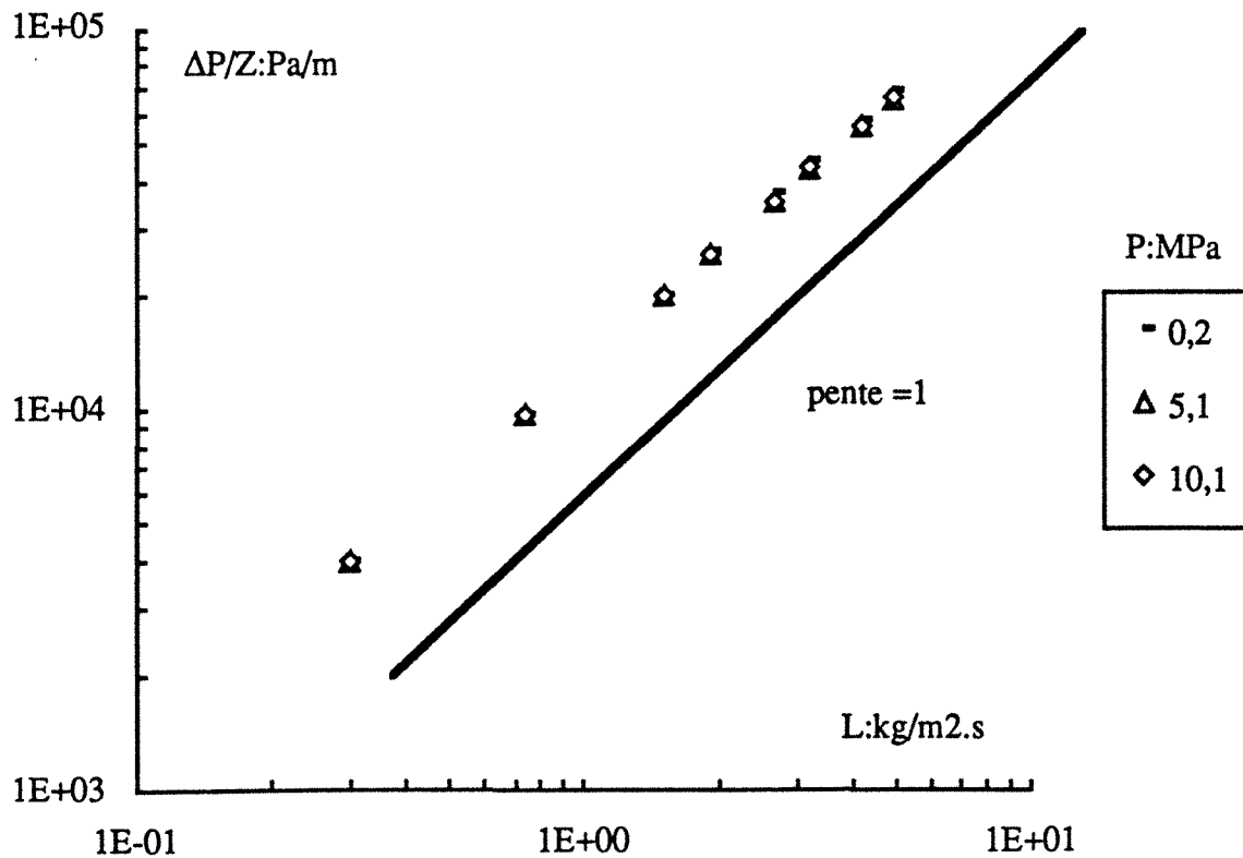
Figure I.5 Evolution de la perte de pression d'ETG en fonction du débit massique. Résultats de Pommier et Hasseni.
