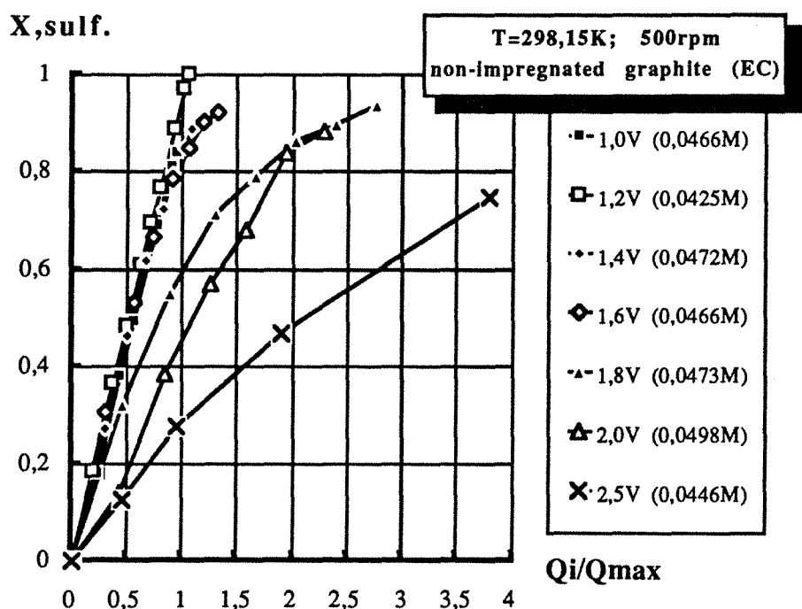
Figure IV.12 Conversion de sulfite en fonction de la charge réduite à différents potentiels de travail sur une électrode en graphite (EC). Tous les essais expérimentaux ont été réalisés à 298,15 K et en milieu \text{Na}_2\text{SO}_4 0,5 M.
