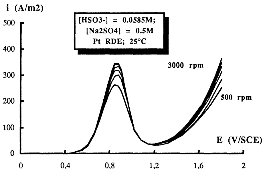
Figure III.7 Courbe intensité-potential de l'oxydation de hydrogénosulfite en sulfate sur électrode tournante en platine ( d=2\text{mm} ). Electrolyte support : \text{Na}_2\text{SO}_4 0,5M.
