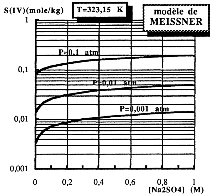
Figure II.13 Molalité en S(IV) en fonction de la concentration en Na 2 SO 4 à 50°C et pour trois pressions partielles différentes de SO 2 .
