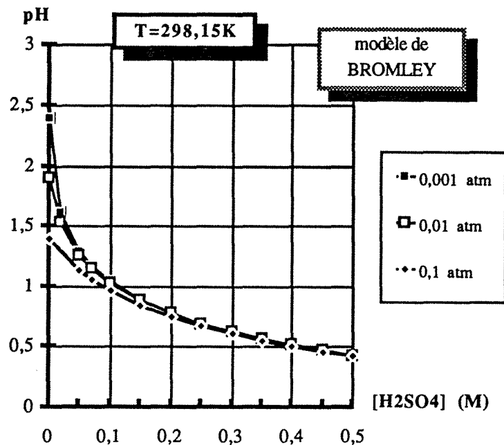
Figure II.17 pH d'une solution aqueuse d'acide sulfurique à 25°C en équilibre avec SO 2 à trois pressions partielles différentes. Les points des différentes courbes sont des valeurs théoriques.
