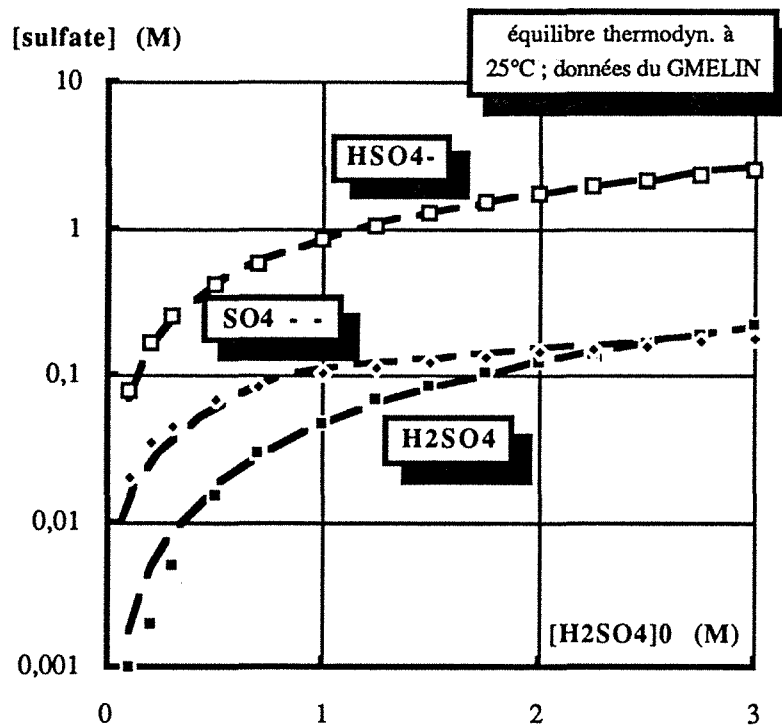
Figure II.5 Concentration en sulfate, bisulfate et acide sulfurique moléculaire en fonction de la concentration de l'acide sulfurique introduit.
