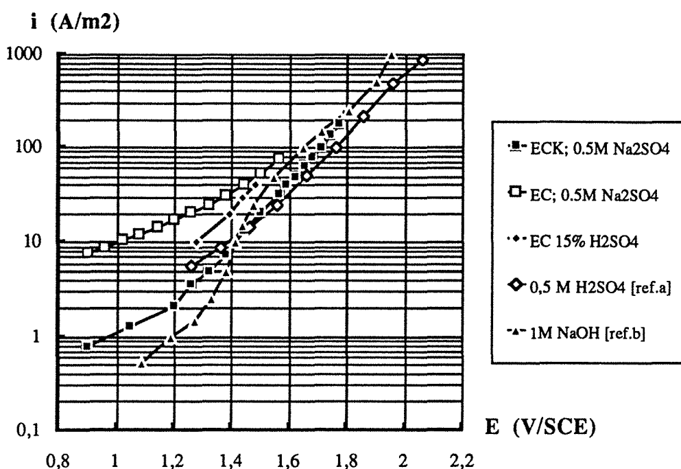
Figure II.10 Courbes voltammétriques sur des électrodes en graphite dans différents électrolytes; ref. a =[TARASEVICH et KHRUSCHEVA]; ref b=[DROSSBACH et SCHMITTINGER]
