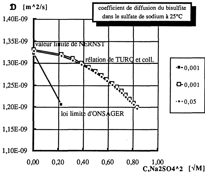
Figure III.18 Coefficients d'autodiffusion du bisulfite ( HSO_3^- ) en fonction de la concentration de l'électrolyte support Na_2SO_4 à 25°C.
