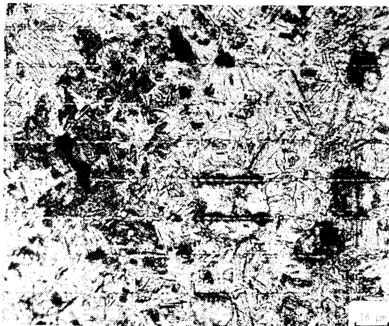
FIGURE III.20 Observation de la trace du palpeur sur la surface bainitique (espacement entre chaque ligne = 16 μm).
