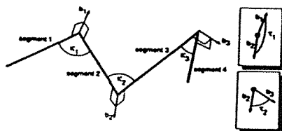
Figure 2.6. Une chaîne de segments 3D : \kappa_i l'angle entre segment_i et segment_{i+1} , \tau_i l'angle entre la normale à segment_i et la normale à segment_{i+1} et segment_{i+2} [Stein and Médioni, 1990].
