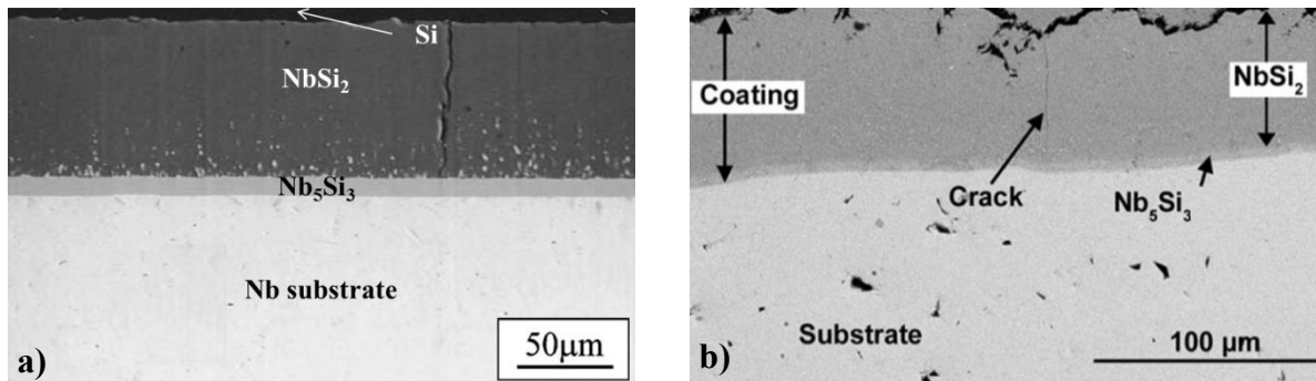
Figure I-11 : Comparaison entre a ) un couple de diffusion Nb/Si (16 h à 1350^\circ\text{C} [84]) et b ) un revêtement déposé par siliciuration haute activité sur un alliage C-103 ( \text{Nb-10Hf-1Ti-0.7Zr-0.5Ta-0.5W} en % at) (6 h 1100^\circ\text{C} [81])
