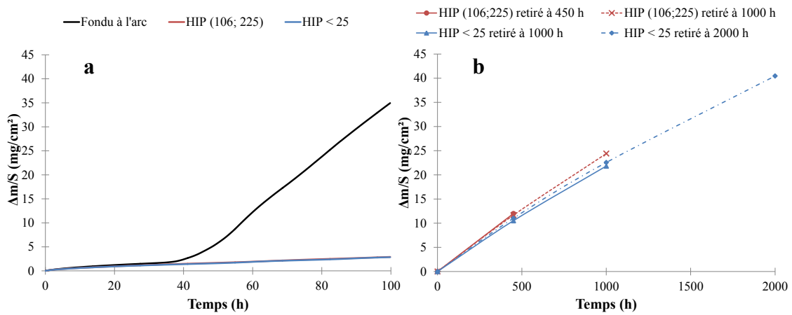
Figure III-11 : a) Courbes thermogravimétriques enregistrées en continu lors de l'oxydation isotherme de 100 h à 815°C des trois microstructures d'alliages Nb ss -Nb 5 Si 3 b) Variations de masse mesurées manuellement au cours de l'exposition à 815°C sur le long terme pour les alliages élaborés par métallurgie des poudres
