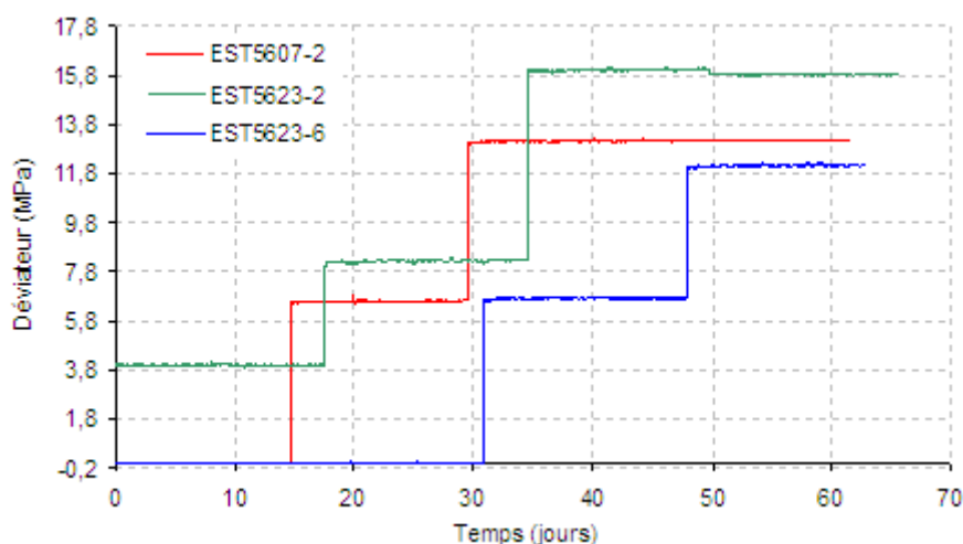
Figure 3.17 : Essais de fluage du LaEGO - Paliers de déviateurs imposés (Hoxha, 2004)
