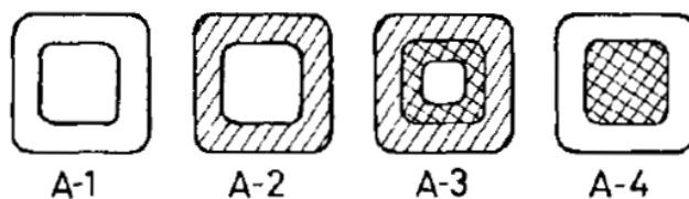
Figure 34 : Modèle pour la modification chimique du bois à l'échelle cellulaire ; A1 : non traité ; A2 : paroi cellulaire imprégnée sans dépôt dans le lumen ; A3 : paroi cellulaire imprégnée avec dépôt à la surface du lumen ; A4 : lumen rempli de produit, mais paroi cellulaire non imprégnée (79)
