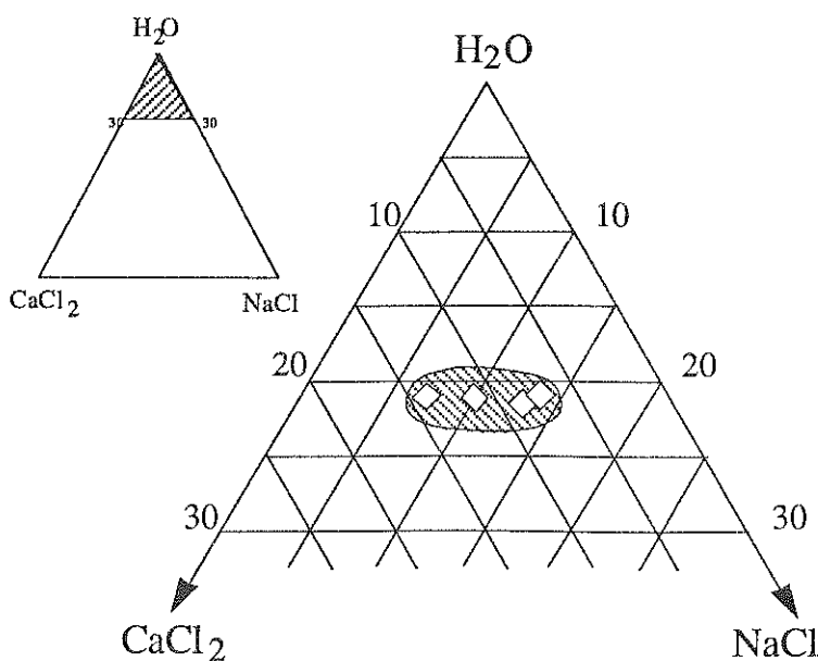
Figure 7.8 : composition des fluides L2
