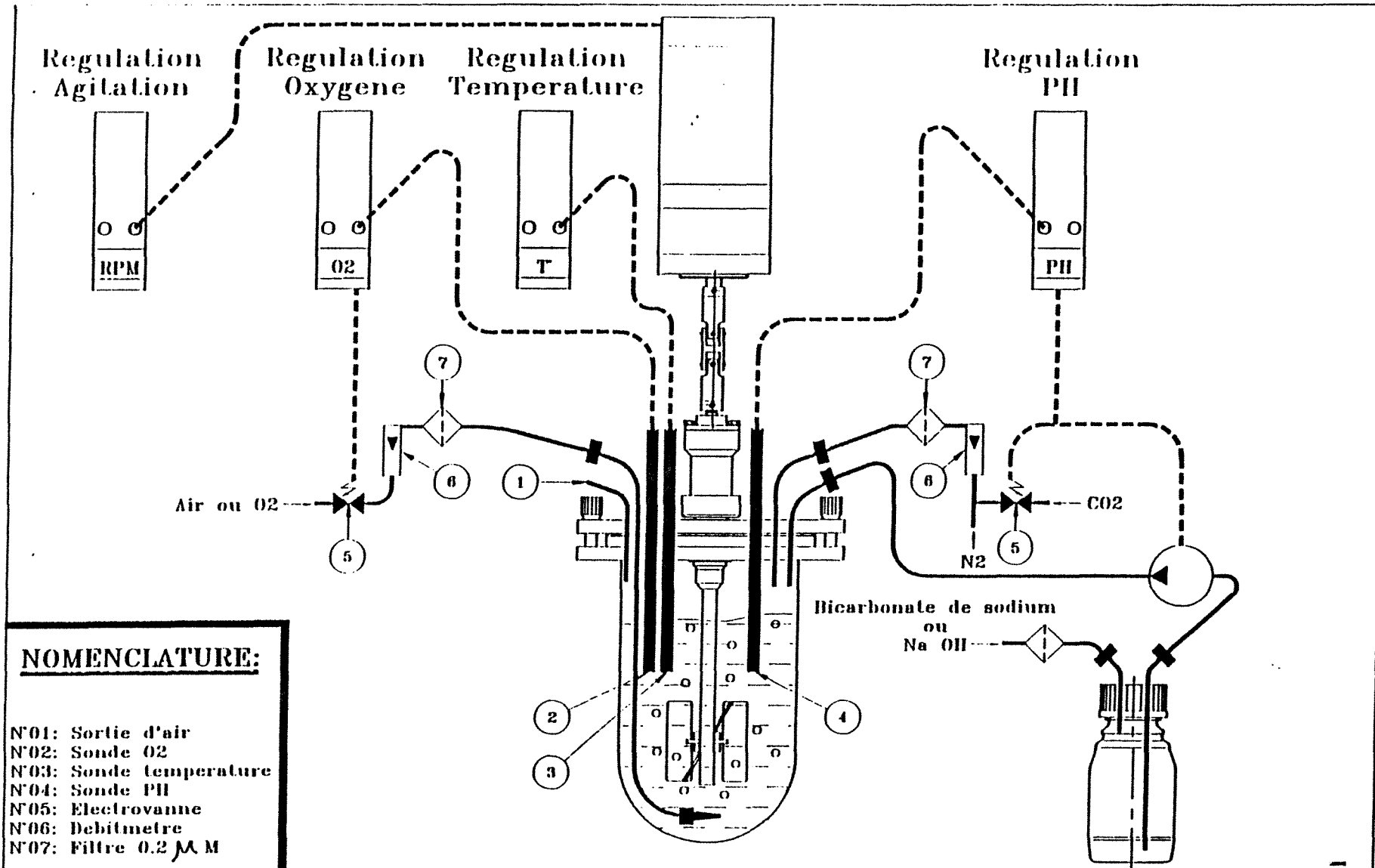
Figure 24: représentation schématique d'un réacteur agité et des différentes régulations.
