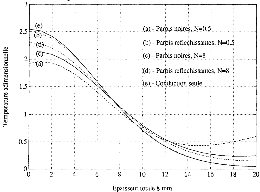
fig. 16: CHAMPS de TEMPERATURE au TEMPS t^*=0.05
