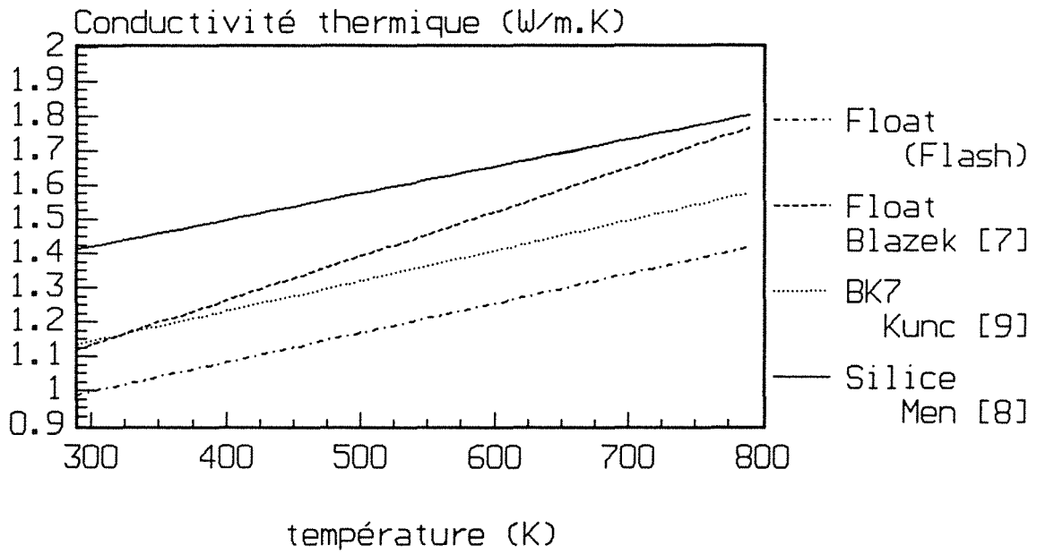
fig.29: Conductivité phonique de différents verres en fonction de la température
