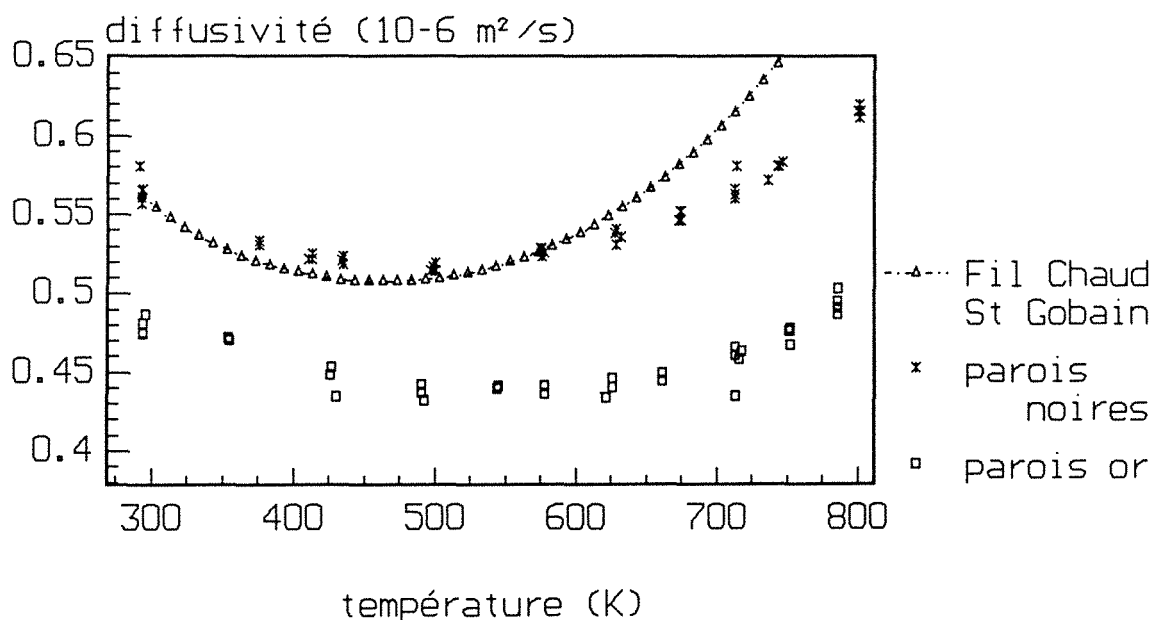
fig. 20: Diffusivité du verre float FC1 en fonction de la température par méthode flash (ref 7011, épaisseur=2mm, %Fe2O3=0.09)
