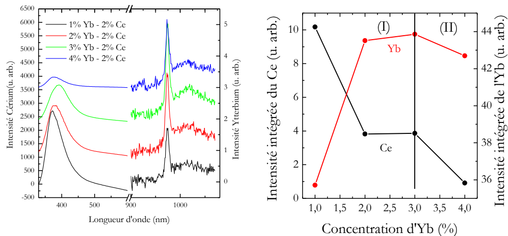
Figure 5-26 (a) Spectres de photoluminescence (mesurés à température ambiante) de films minces de \text{SiO}_2 co-dopés (Ce, Yb) et recuits à 500^\circ\text{C} , mesurés dans le visible et l'IR . (b) Evolution des intensités intégrées de luminescence du \text{Ce}^{3+} (en noir) et de l' \text{Yb}^{3+} (en rouge) en fonction de la concentration d'Yb pour une température de recuit de 500^\circ\text{C} .
