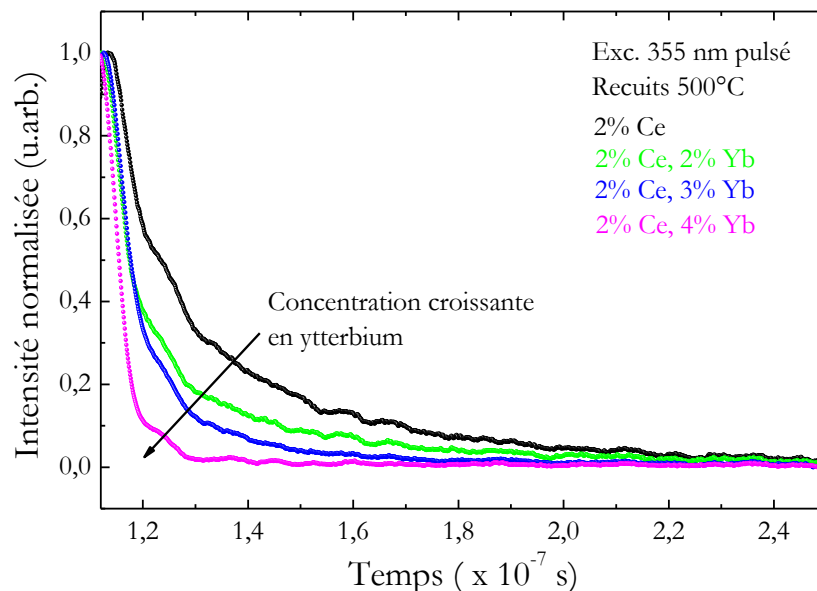
Figure 5-27 Déclins de luminescence mesurés sur les échantillons recuits à 500^\circ\text{C} avec une concentration de Ce fixée à 2% et une concentration d'Yb variant entre 2 et 4%.
