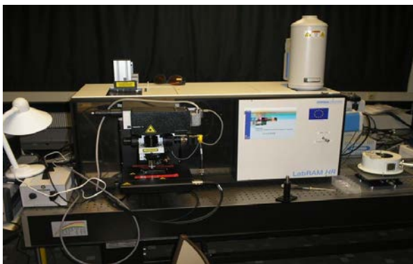
Figure 2-12 Photographie du spectromètre Raman (à gauche) et schéma de principe (à droite).
