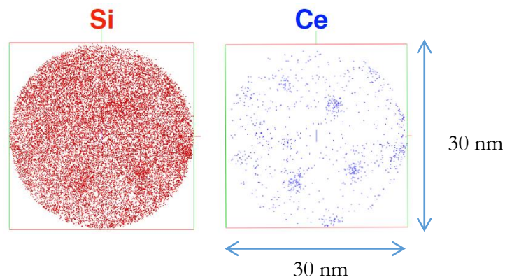
Figure 4-7 Cartographie des atomes de Si et de Ce obtenue par sonde atomique tomographique d'un film mince de SiO 1,5 dopé avec 3% de cérium et non recuit. Les tranches mesurent 30 x 30 x 5 nm 3 .
