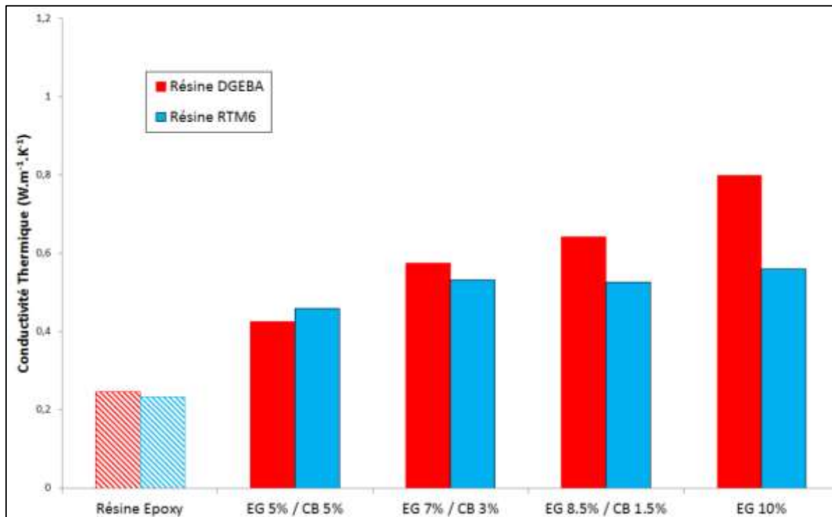
Fig. IV-23 – Conductivité thermique des composites EG/CB en fonction du rapport massique des charges et de la matrice époxy utilisée
