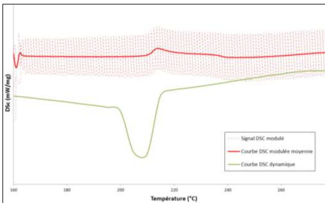
Fig. III-6 – Analyse du pic endothermique par DSC modulée sous air, 1K/min, P = 60 sec, A = 0,5K
