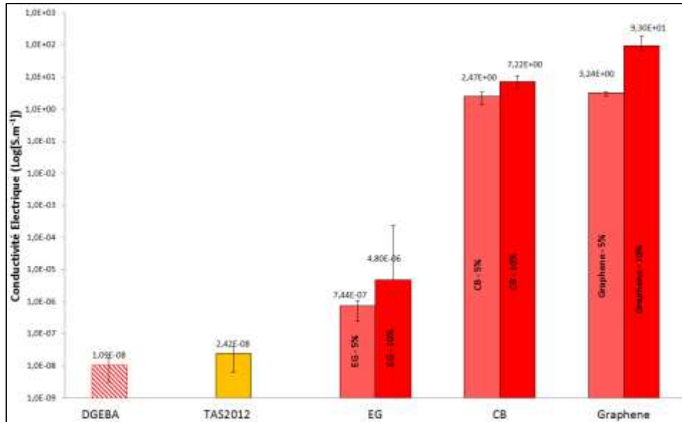
Fig. V-28 – Conductivités électriques des nanocomposites à base de graphène
