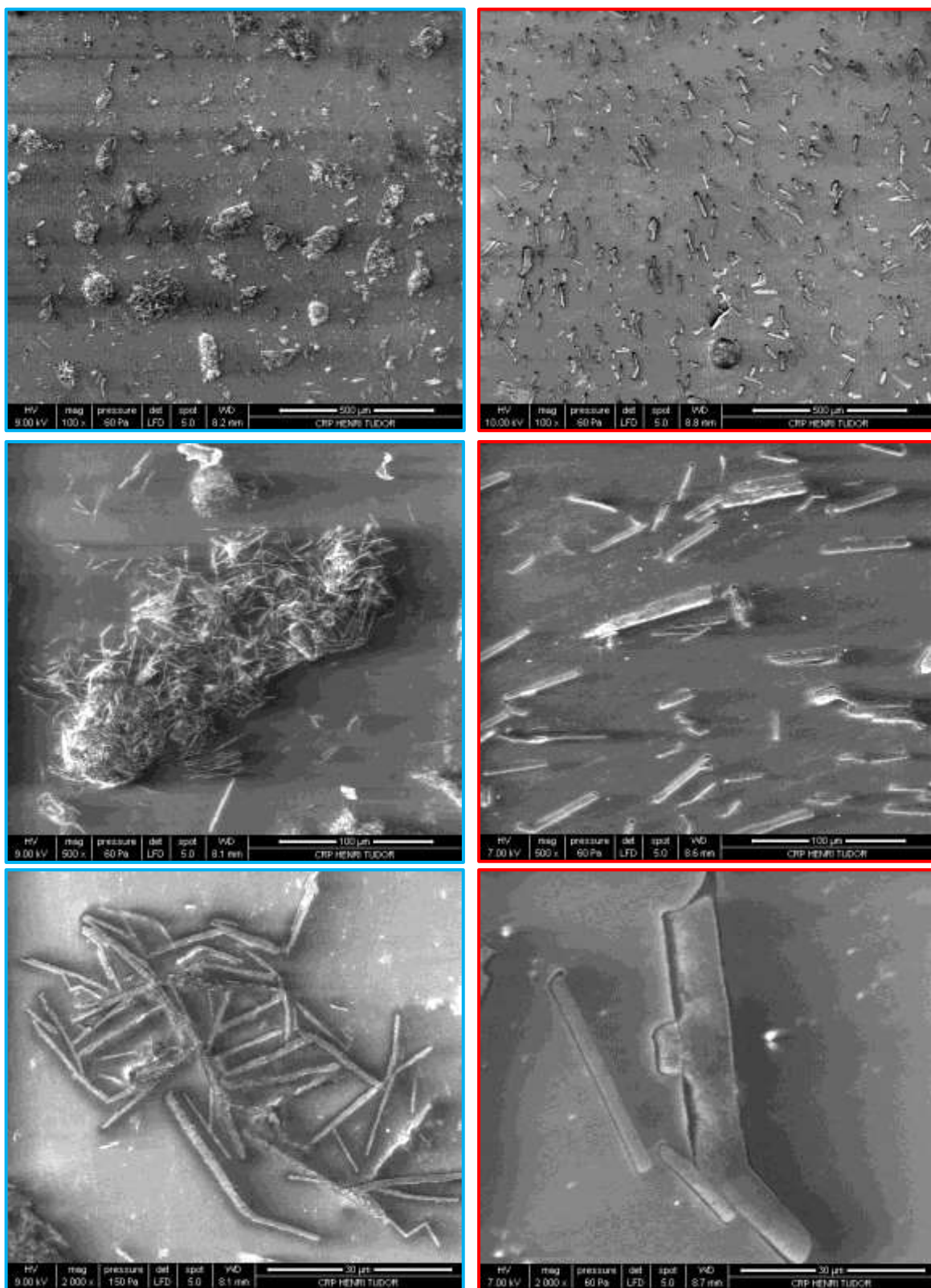
Fig. III-55 – Observations MEB des échantillons NB482-10% (à g.) et NB501-10% (à d.)
