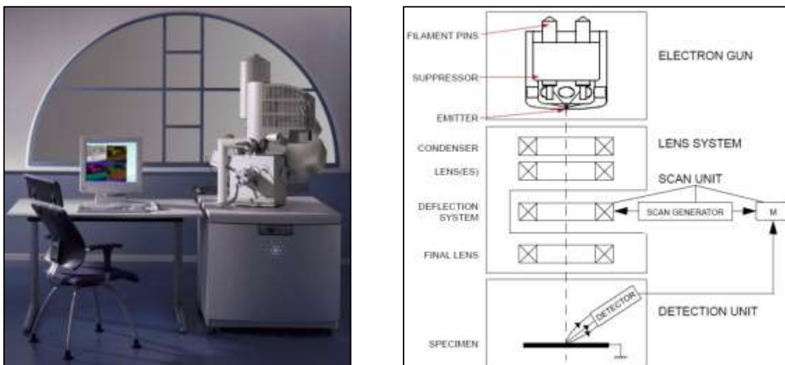
Fig. II-27 – Quanta FEG SEM (à d.) & principe du MEB (à d.)
