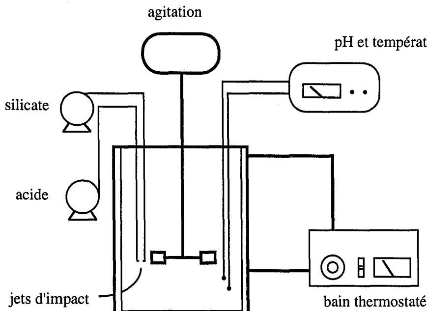
Figure IV-1 : Montage expérimental
