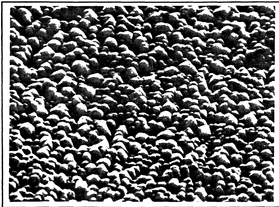
Figure V-13 : Morphologie d'un revêtement de zircone réalisé à 480 °C sur un substrat en Zircaloy-4, dans les conditions de référence modifiées ( DH_2=8 \text{ Ncm}^3/\text{mn} ) (M.E.B.) : a) section transversale b) surface du dépôt de zircone.
