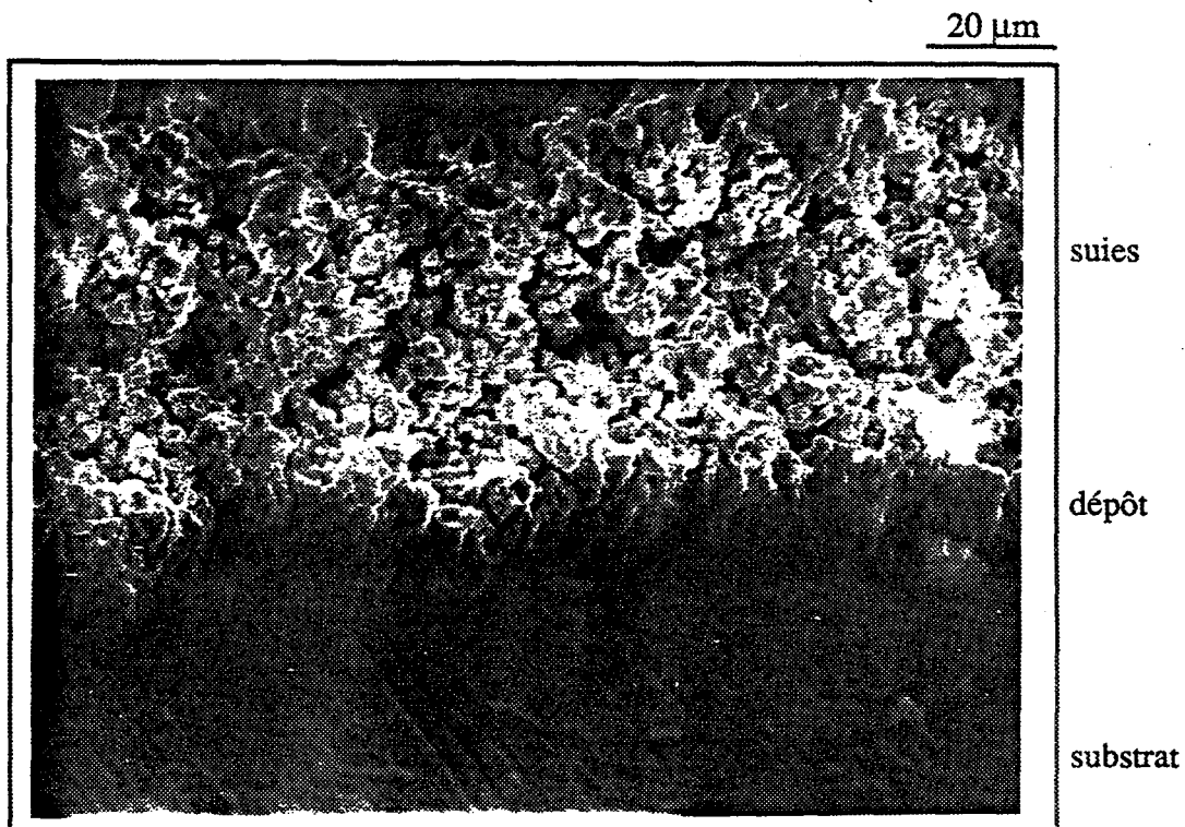
Figure IV-16 : Morphologie du dépôt CVD de zircone (section transversale) synthétisé à 300 °C par hydrolyse de \text{ZrCl}_4 (M.E.B.). (côte z = 3 cm).
