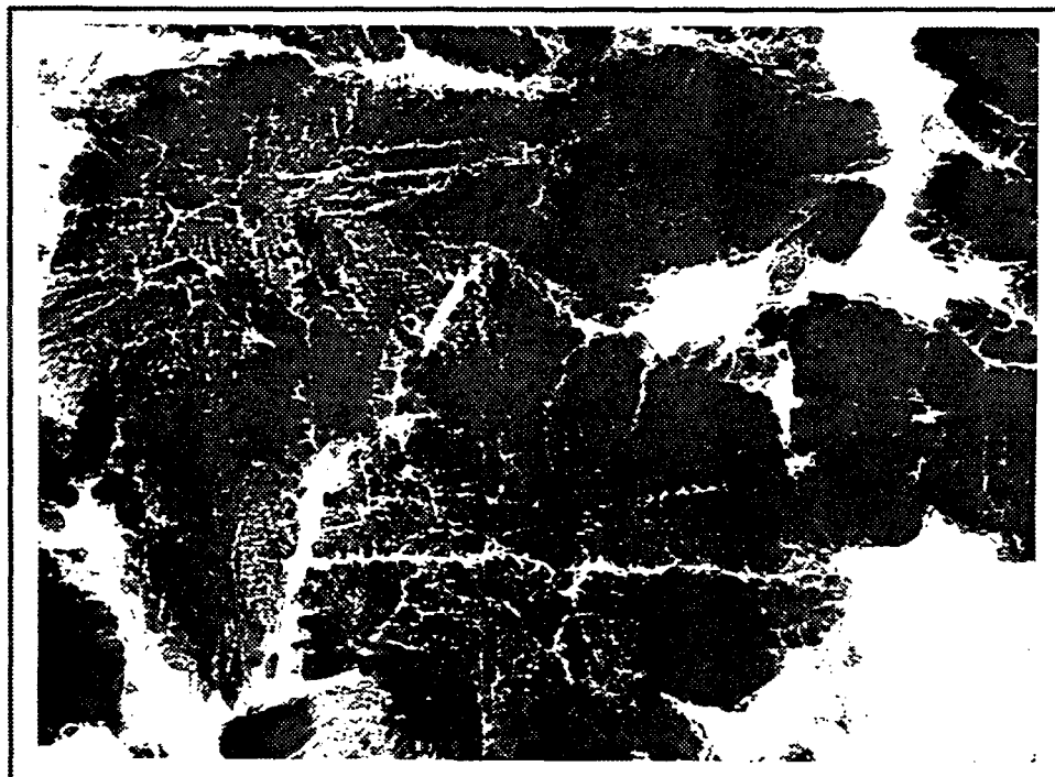
Figure V-12 : a) Observation en sens travers d'une colonne de zircone b) observation en sens parallèle de deux colonnes voisines (T.E.M., fond clair). Lamme prélevée dans la partie la plus externe du dépôt. Traitement réalisé à 300 °C sur un substrat en Zircaloy-4, dans les conditions de référence.
