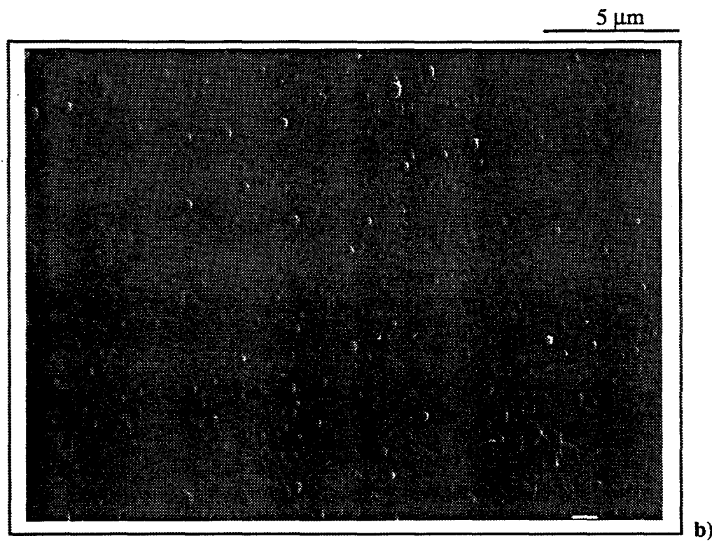
Figure V-16 : Observation des défauts de croissance à la surface de deux dépôts de zircone réalisés sur un substrat en Zircaloy-4, dans les conditions de référence, à différentes températures (M.E.B.) : a) 300 °C b) 460 °C.
