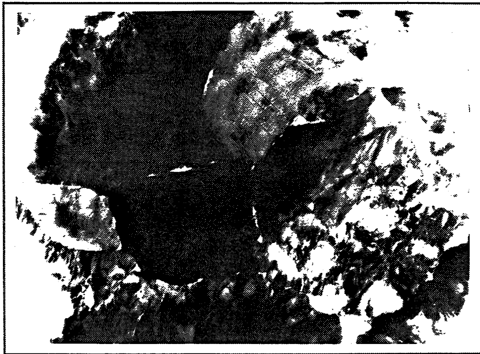
Figure V-10 : Observation en sens parallèle de la partie la plus externe du dépôt de zircone (T.E.M., fond clair). Traitement réalisé à 460 °C sur un substrat en Zircaloy-4, dans les conditions de référence.
