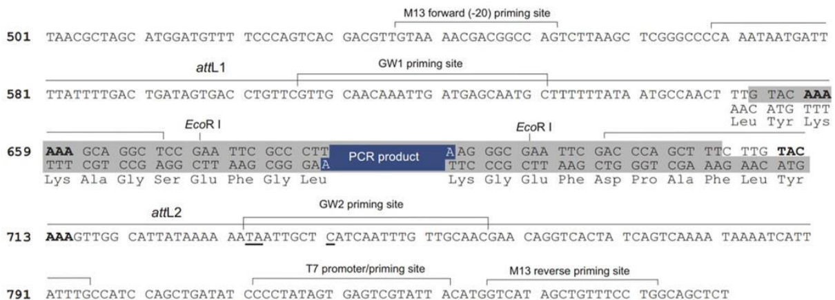
Figure 29 : Polylinker du vecteur pCR8®/GW/TOPO® (Invitrogen).
