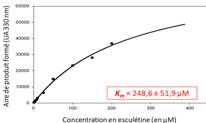
Figure 78 : Quantité de produit inconnu formé par CYP71AZ3 en fonction de la concentration en esculétine.
