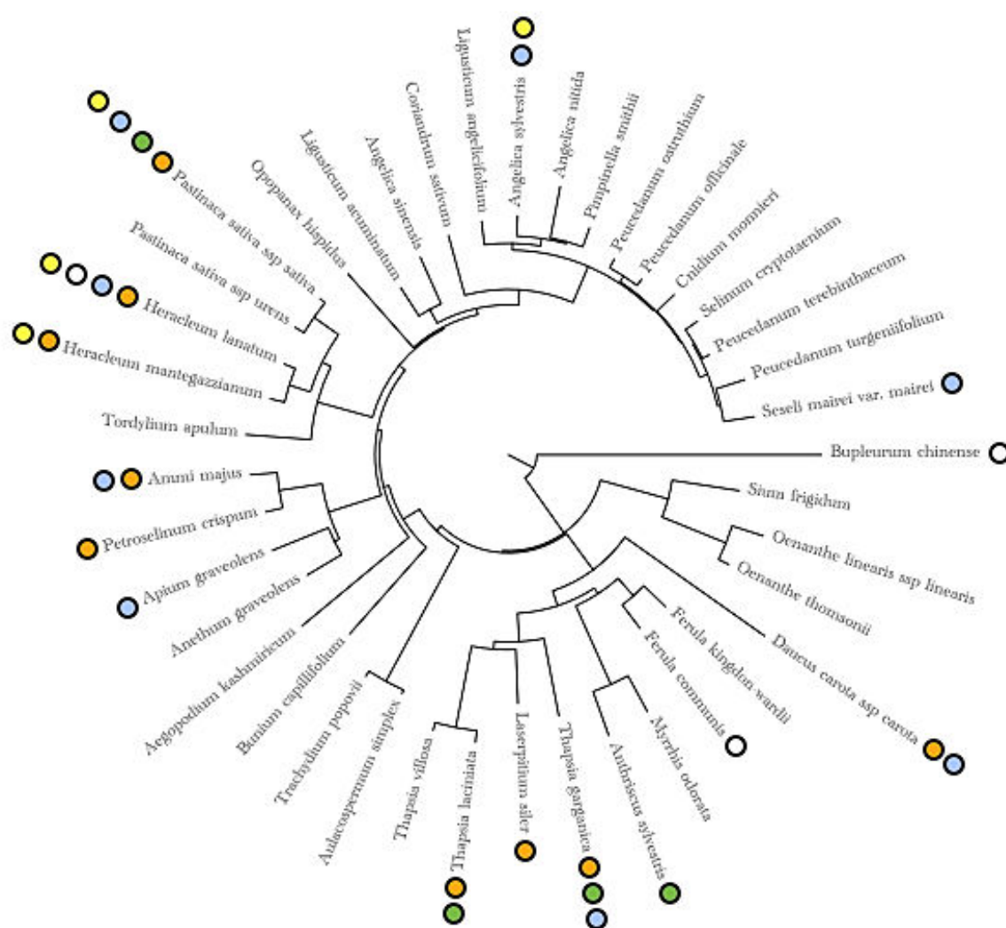
Figure 88 : Arbre phylogénétique de différentes Apioidées et occurrence de la sous-famille CYP71AJ. L’arbre a été construit à l’aide de MEGA5.2.2 à partir des séquences ITS identifiées par Downie et ses collaborateurs (Downie et al. , 2001). En bleu : espèces chez qui une psoralène synthase ou une psoralène synthase putative a été identifiée ; en jaune : angélicine synthase ou angélicine synthase putative ; en orange : clade 1, inconnu ; en vert : clade 2, inconnu ; en blanc : inconnu.
